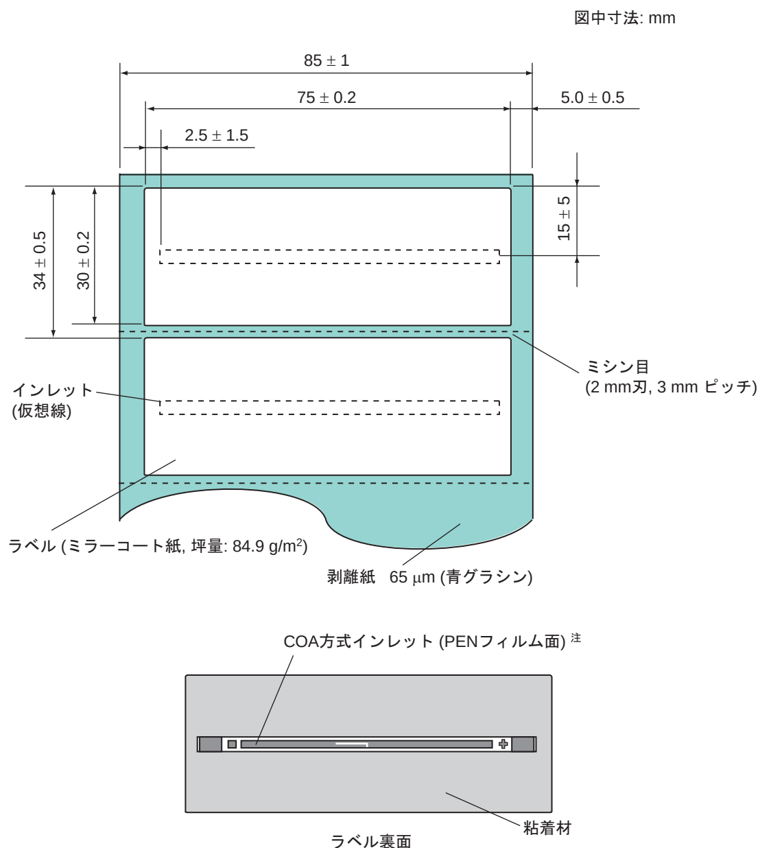
図 1 紙ラベル型インレットの構造 (HKT100***FL001 の例)
