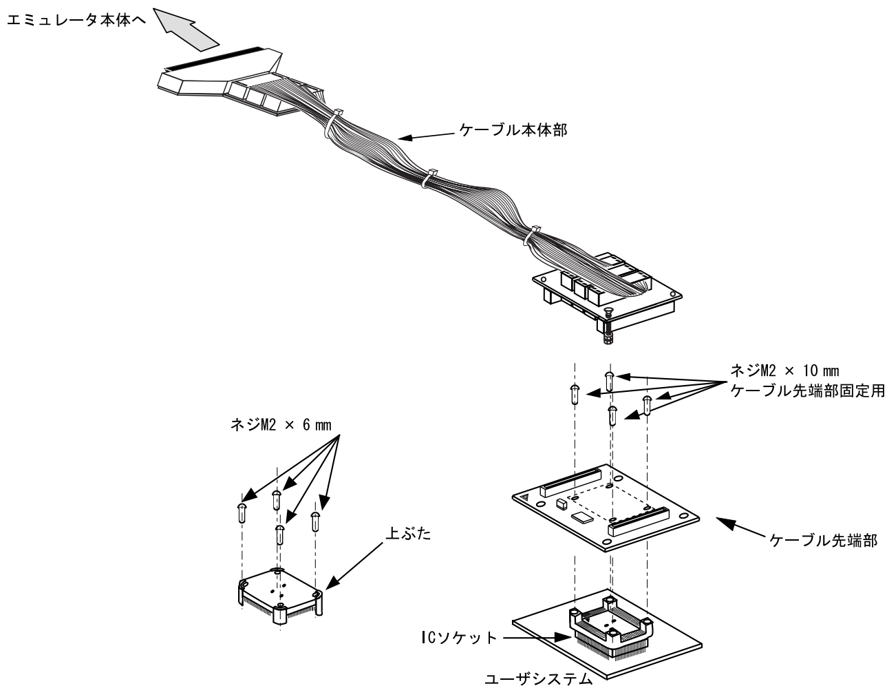
図 1 HS2678ECH61H ユーザシステムインタフェースケーブル
