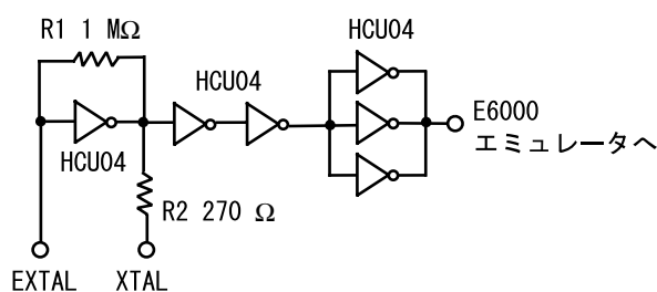
図 10 クロック発振回路
