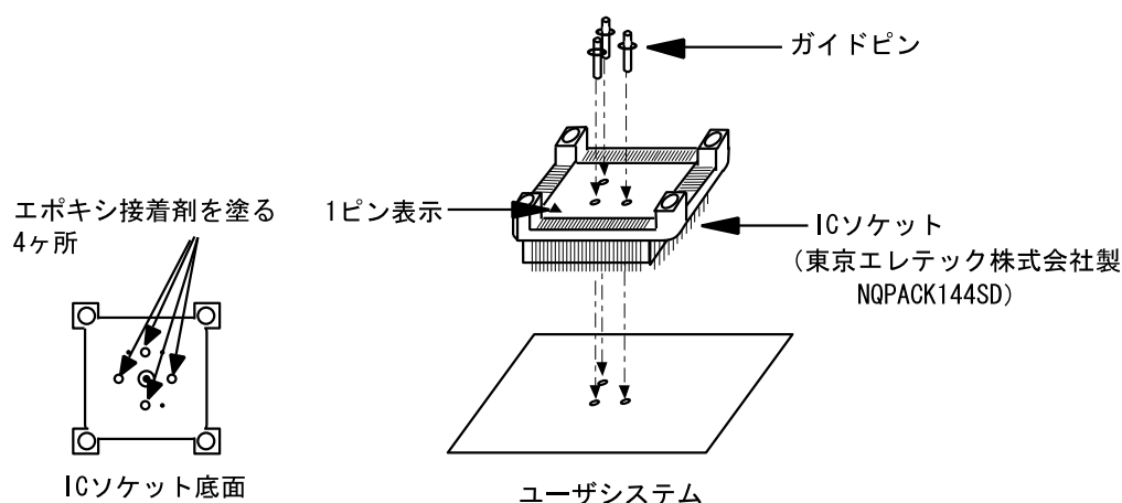
図3 ICソケットの位置決め
