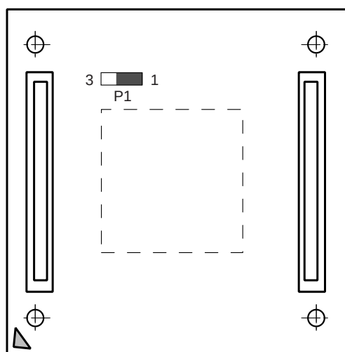
図 12 P1 ショートコネクタ
