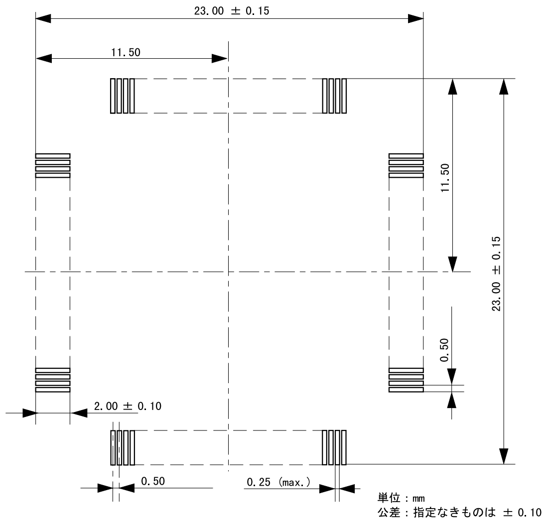
図6 推奨マウントパッド寸法
