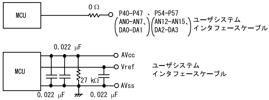
図 2-4 P40-P47、P54-P57、Vcc、AVcc、AVss、Vref信号回路
