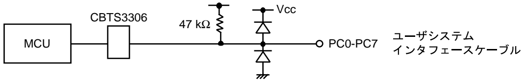
図 7-4 PC0-PC7 信号回路
