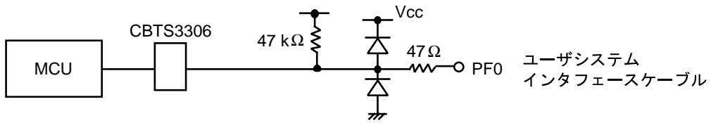
図 7-3 PFO 信号回路
