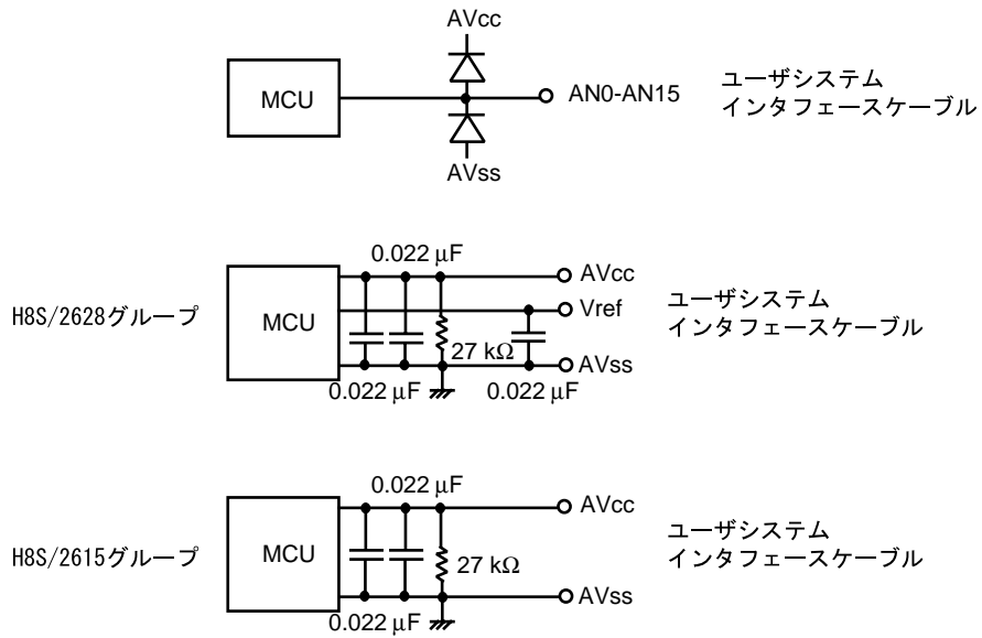
図 7-5 AN0-AN15, Avcc, Avss, Vref 信号回路
