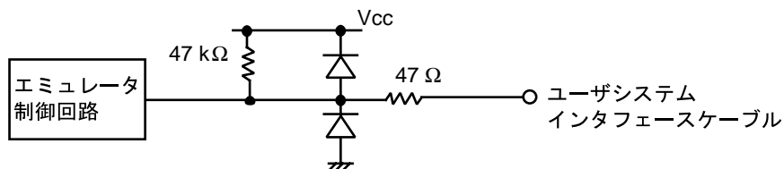
図 7-2 モード端子、NMI、STBY、RESET 信号回路
