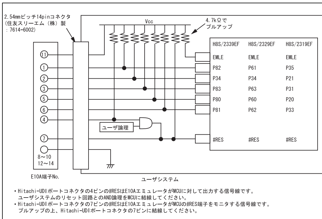
図 6.2 E10A との接続例
