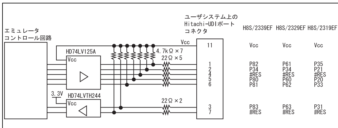
図 6.6 エミュレータ内インタフェース回路 (参考)
