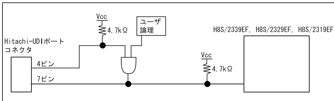
図 6.5 #RES 端子の結線
