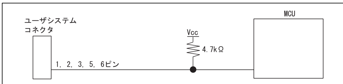
図 1.4 E10A-USB エミュレータと MCU の接続
