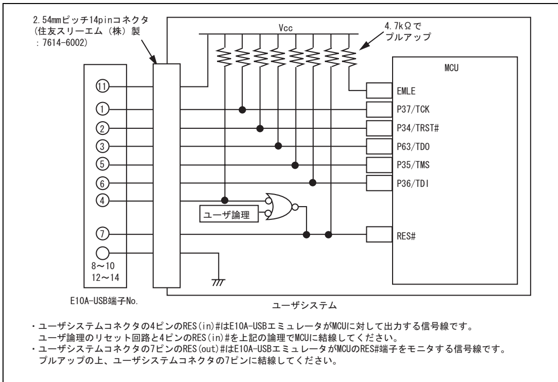
図 1.3 E10A-USB の接続例
