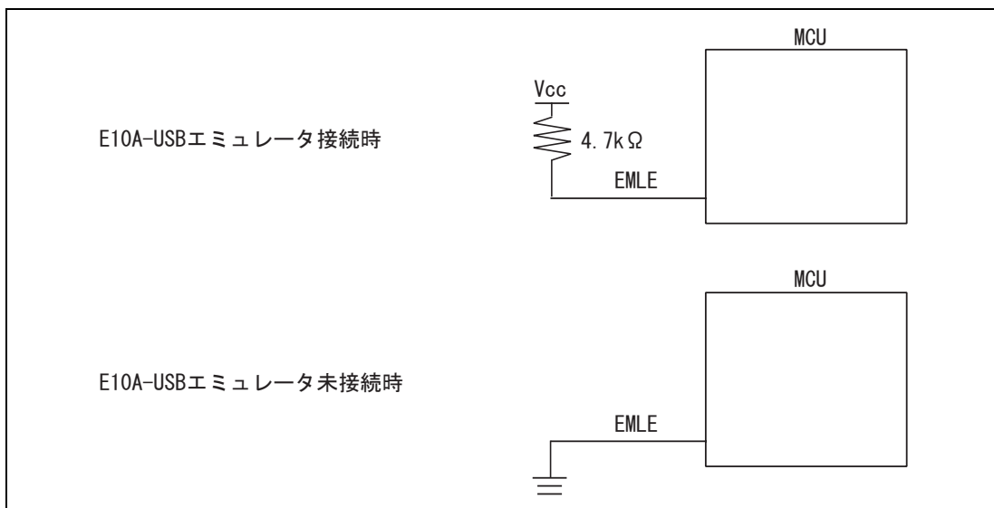
図 1.5 E10A-USB エミュレータと EMLE 端子
