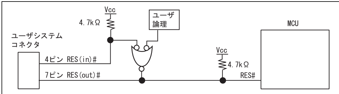
図 1.6 RES#端子の結線
