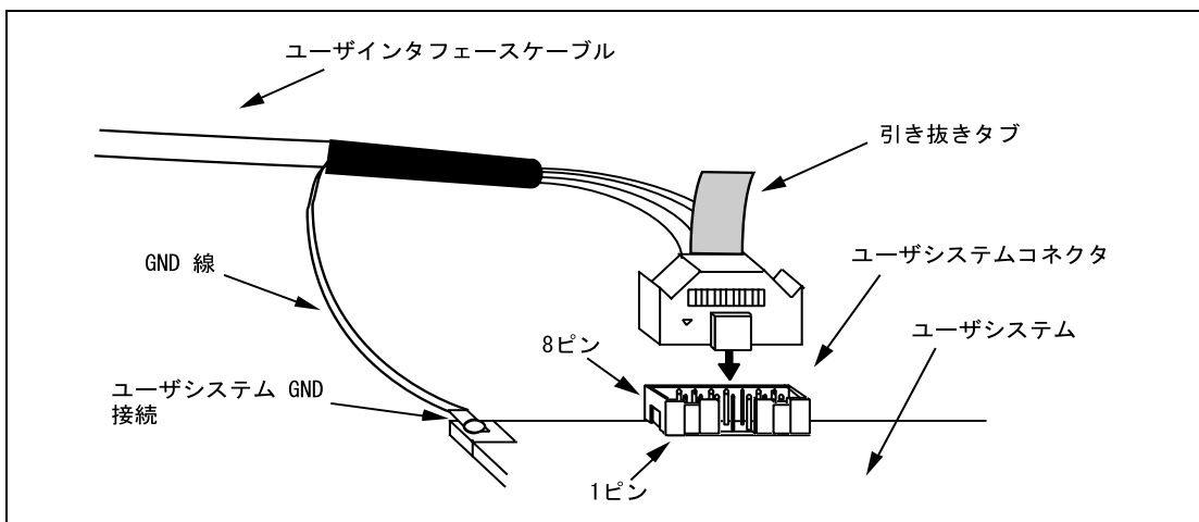
図 1.1 14 ピンストレートタイプコネクタ使用時のユーザシステム側のユーザインタフェースケーブル接続方法
