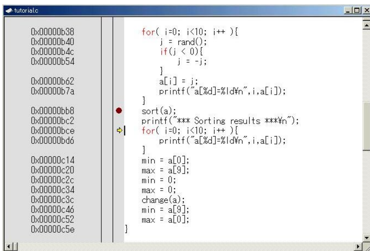
図 5.26 Source ウィンドウ ( Step Over )
