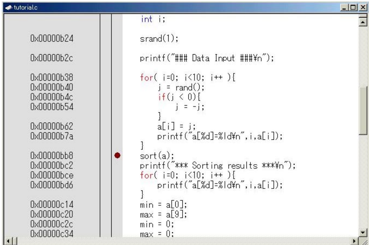
図 5.4 Source ウィンドウ (ブレークポイントの設定)
