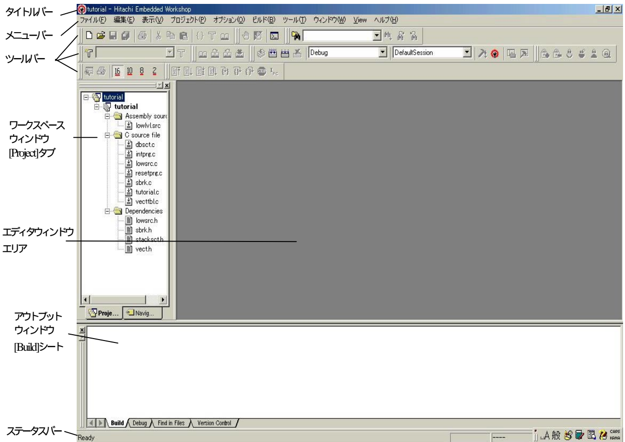
図 2.12 HEWのウィンドウ構成
