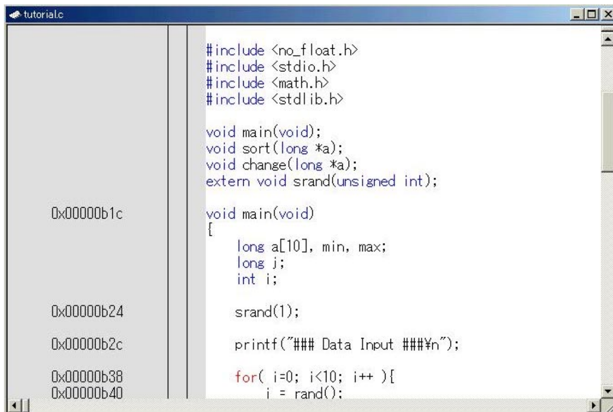
図 5.3 Source ウィンドウ（ソースプログラムの表示）
