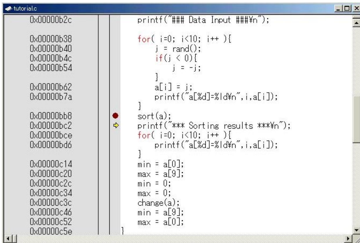
図 5.24 Source ウィンドウ ( Step Out )
