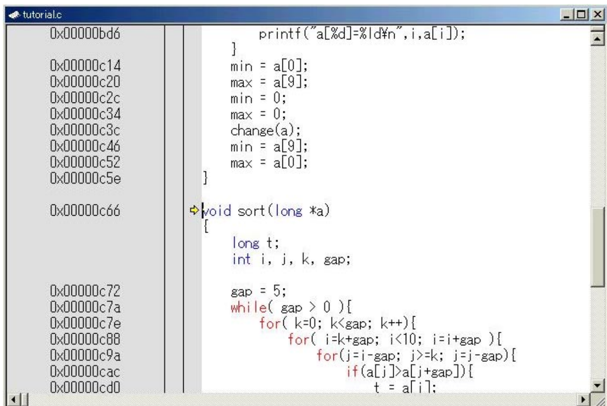
図 5.22 Source ウィンドウ ( Step In )
