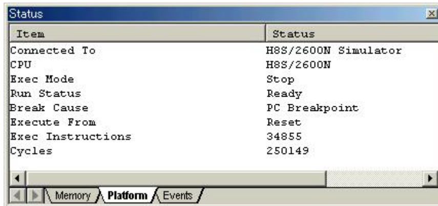
図 5.12 Status ウィンドウ
