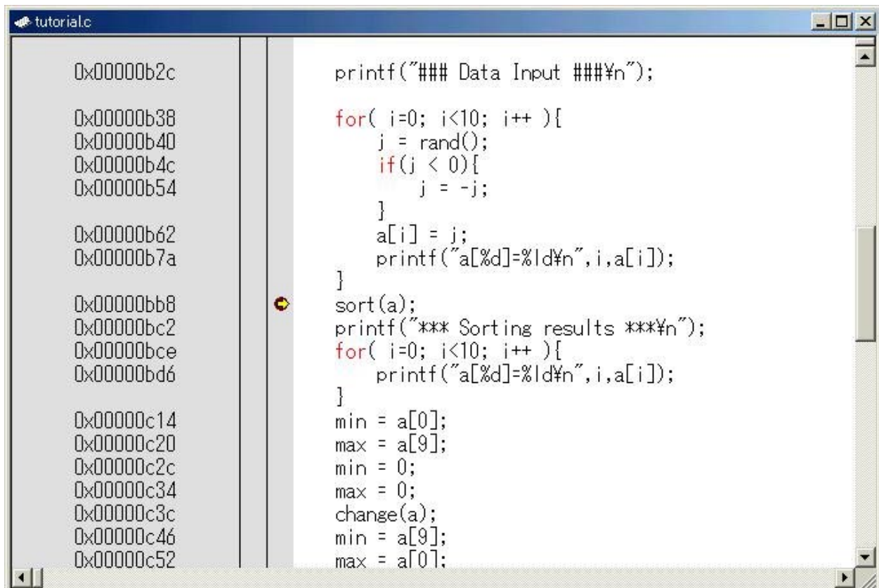
図 5.11 Source ウィンドウ (ブレーク状態)
