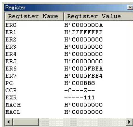
図 5.13 Register ウィンドウ
