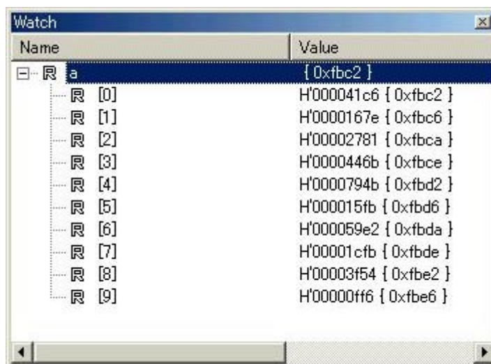
図 5.20 Watch ウィンドウ
