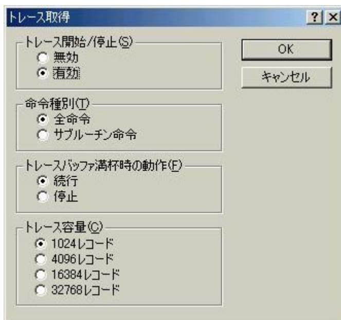
図 5.8 トレース取得ダイアログボックス
