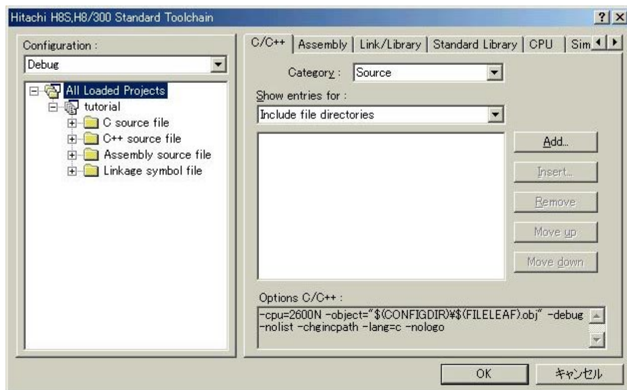
図 4.1 C/C++コンパイラのオプション設定ダイアログボックス
