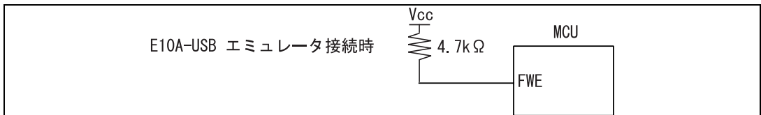
図 1.7 FWE 端子の結線
