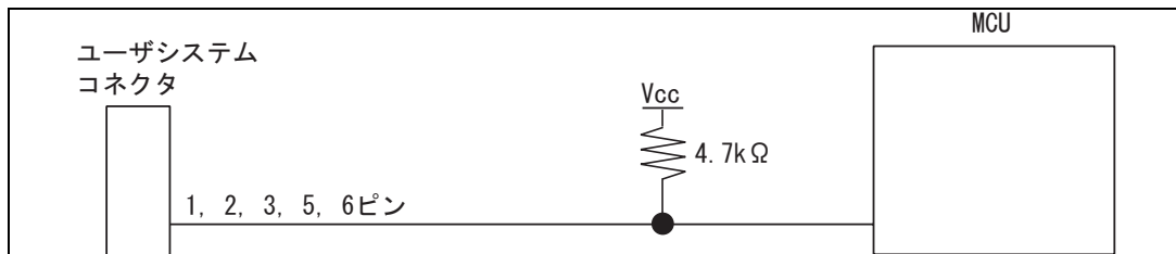
図 1.4 E10A-USB エミュレータと MCU の接続
