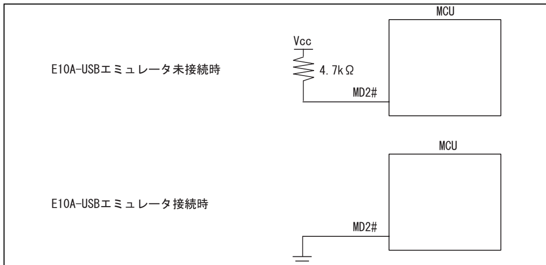
図 1.5 E10A-USB エミュレータと MD2# 端子
