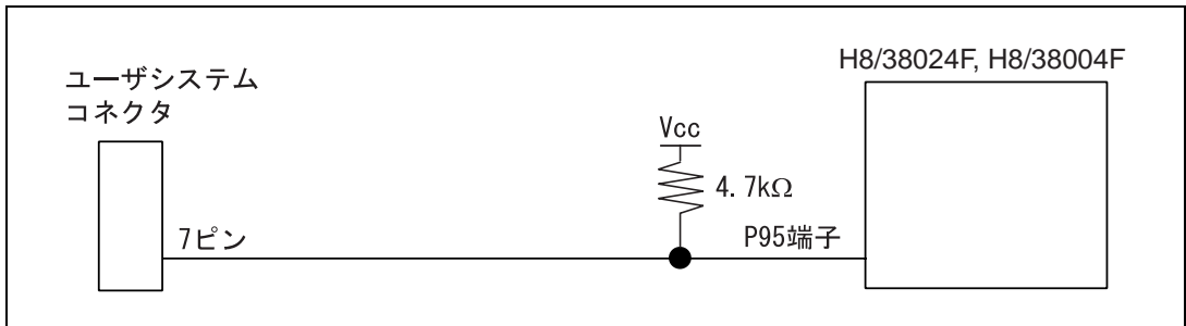
図 6.4 E10T エミュレータと P95 端子の直接接続
