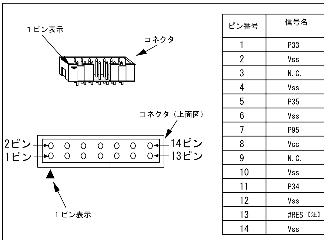
図 6.1 コネクタのピン配置
