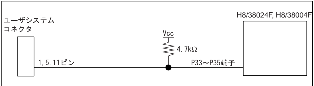
図 6.3 E10T エミュレータと MCU の接続
