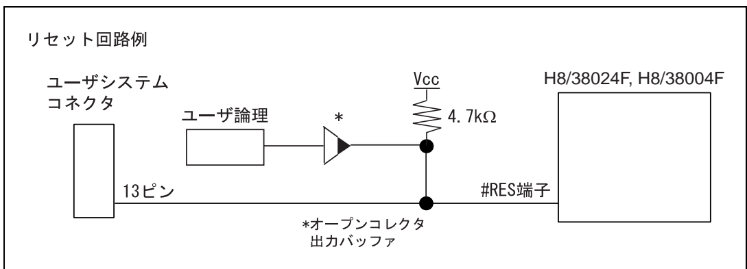
図 6.5 リセット回路例
