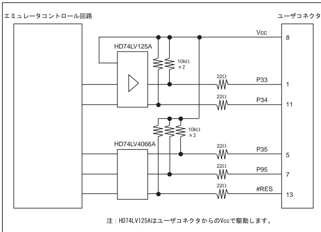
図 6.6 エミュレータ内インタフェース回路 (参考)
