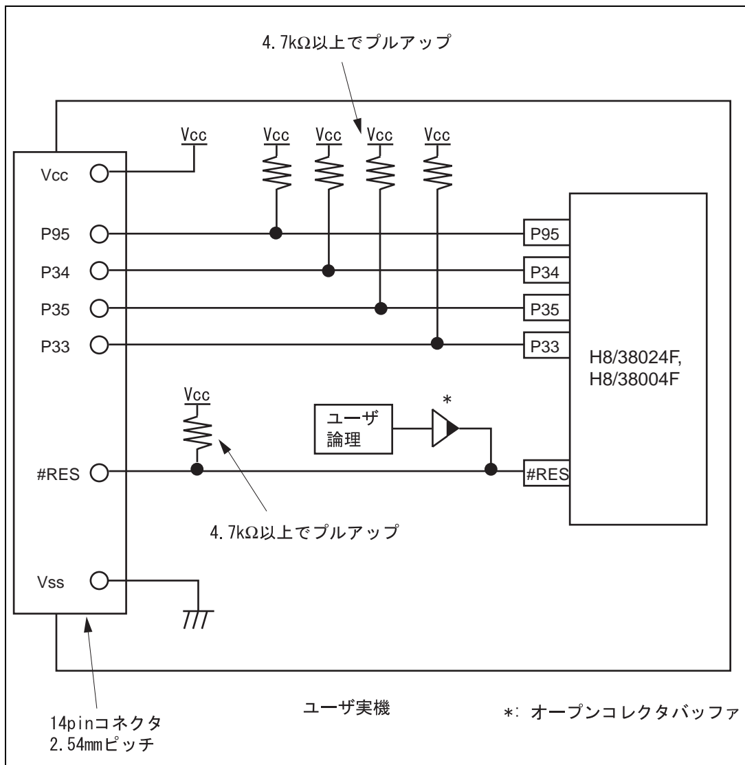
図 6.2 E10T 接続例
