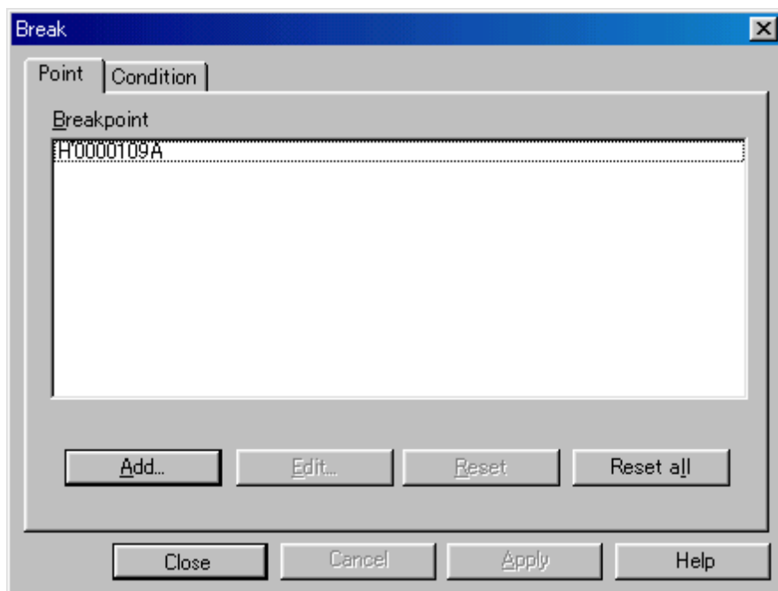
図 3.36 [ Point ] ページ ([ Break ] ダイアログボックス) (ソフトウェアブレークポイント設定後)
