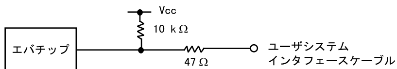
図 7-2 OSC1 および X1 信号
