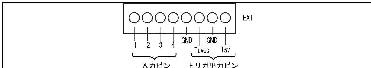
図 2-7 外部プローブコネクタ
