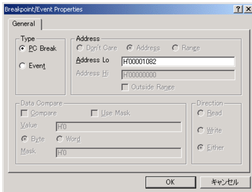
図 6-33 [Breakpoint/Event Properties]ダイアログボックス
