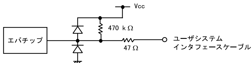
図 7-1 ユーザインタフェース信号回路
