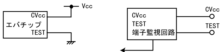
図 7-5 CVcc、TEST 信号
