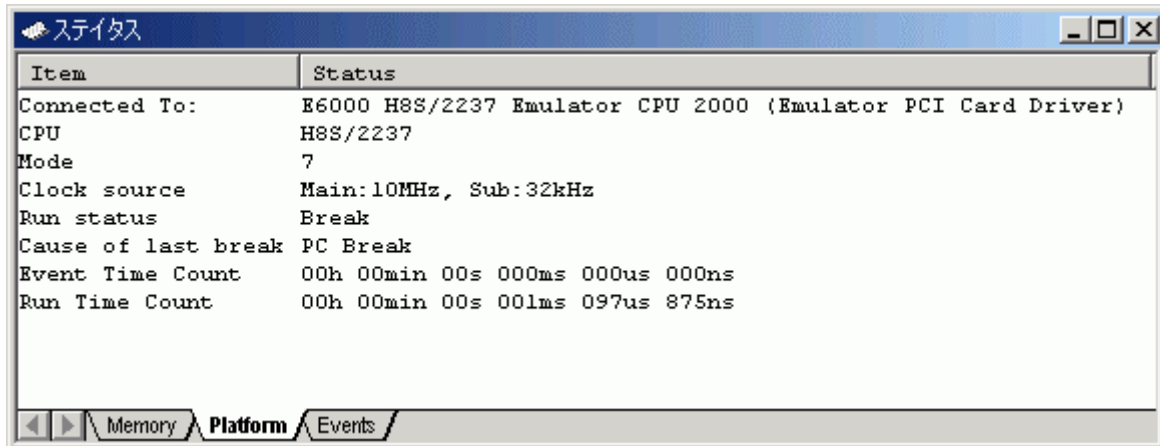
図 6-36 [ステータス]ウィンドウの表示内容 (PC ブレーク)
