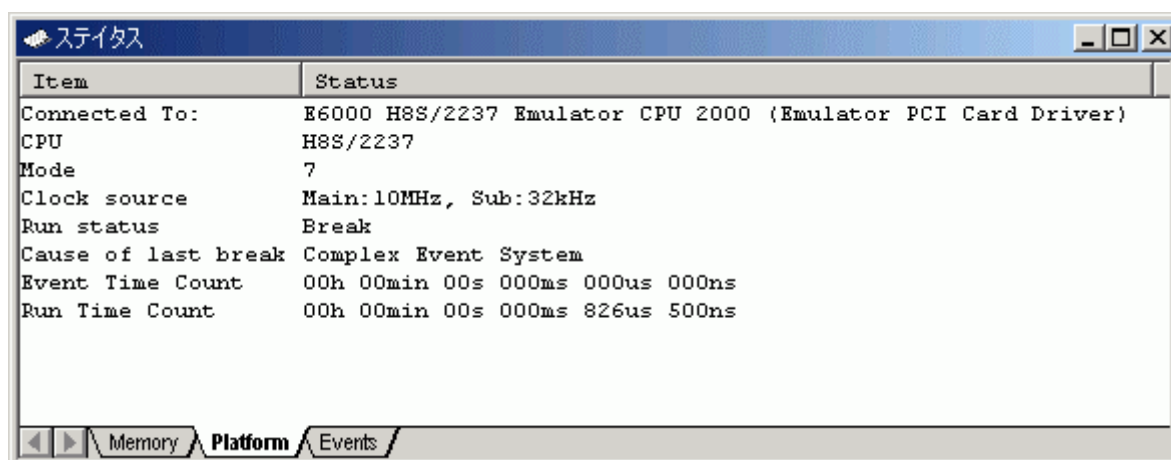
図 6-41 [ステータス]ウィンドウの表示内容
