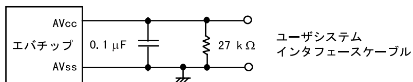
図 7-4 AVcc、AVss 電源端子
