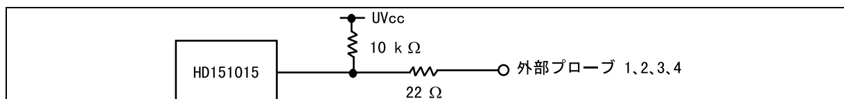
図 2-8 外部プローブインタフェース回路
