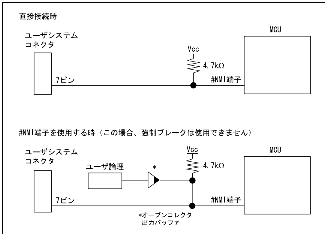
図 6.4 E10T エミュレータと#NMI 端子の接続
