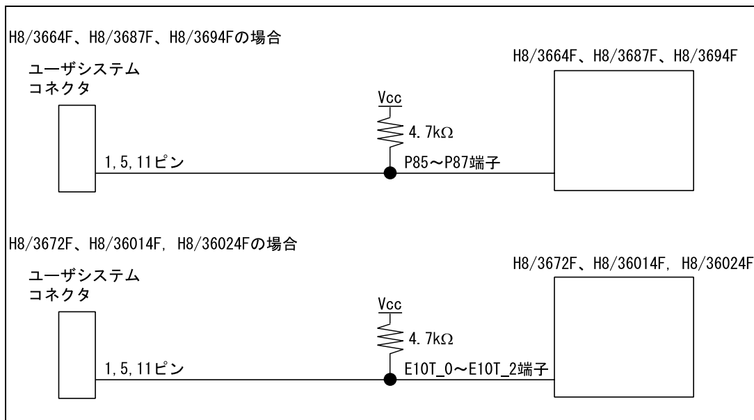
図 6.3 E10T エミュレータと MCU の接続
