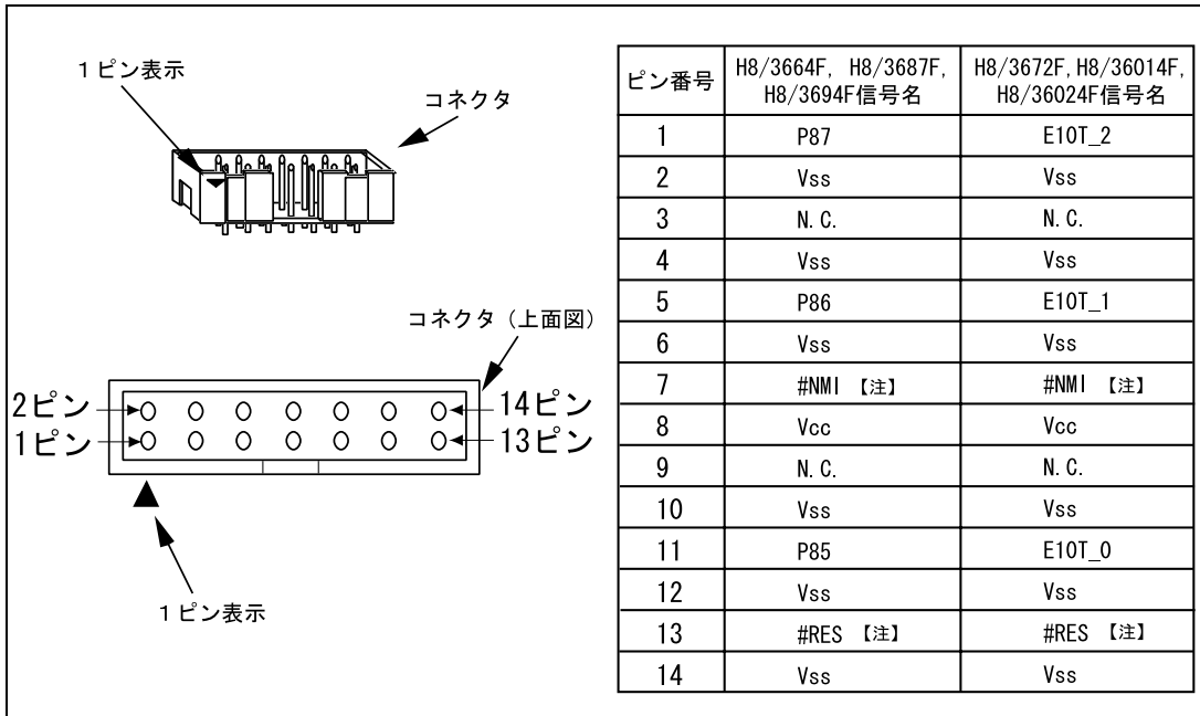
図 6.1 コネクタのピン配置
