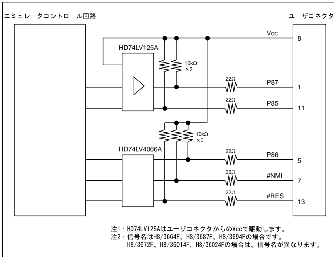
図 6.6 エミュレータ内インタフェース回路 (参考)
