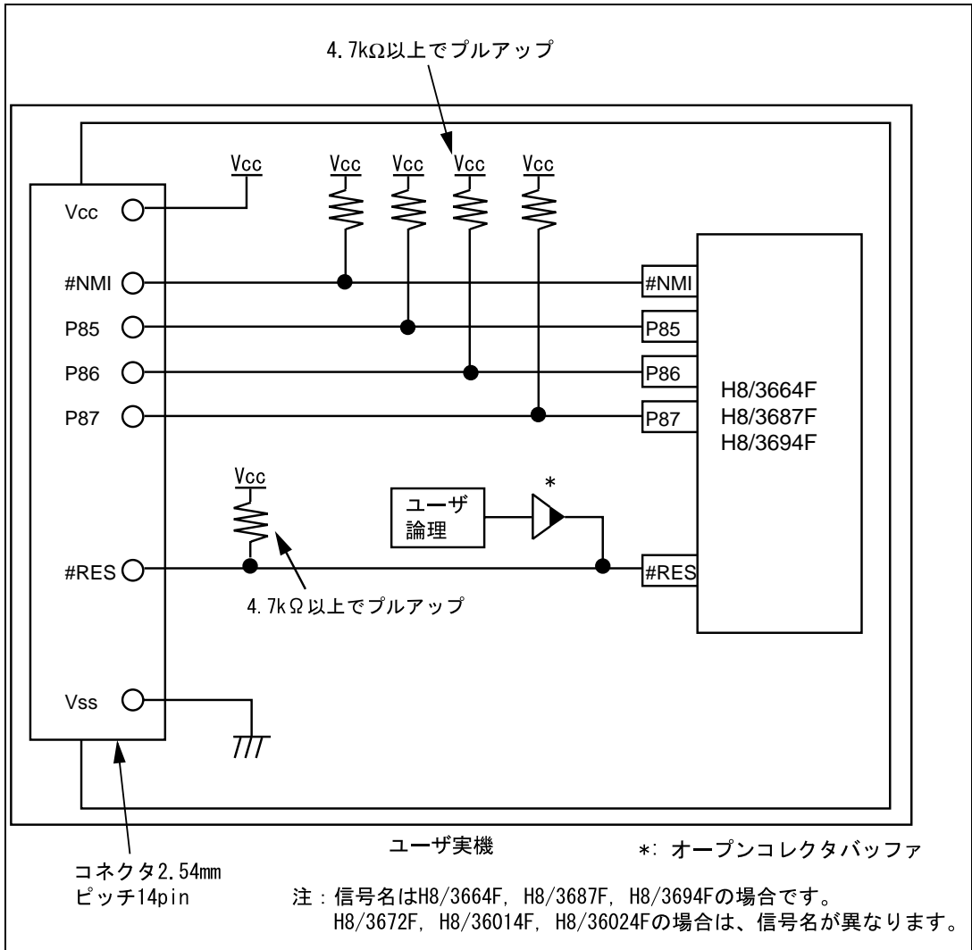
図 6.2 E10T の接続例
