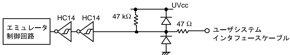
図 7-2 /RES 信号、NMI 信号回路
