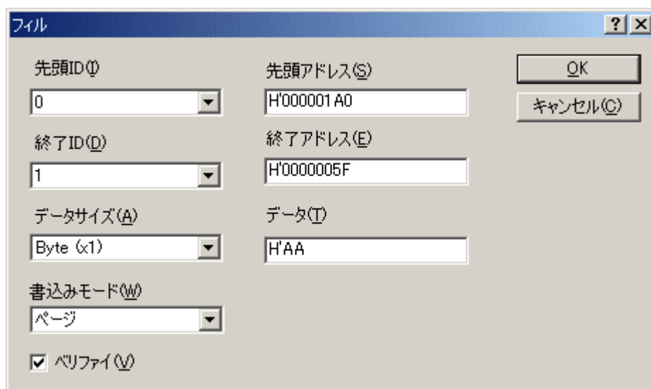
図 8-6 フィルダイアログボックス
