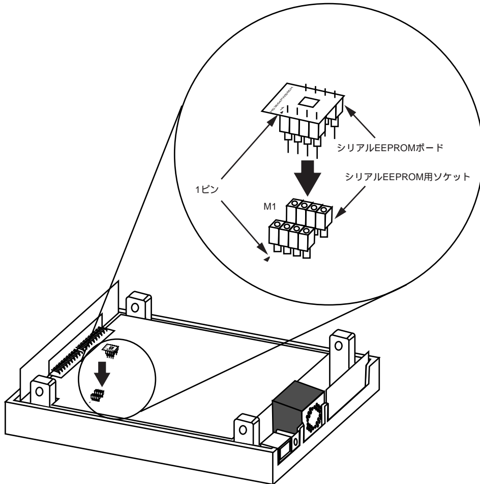
図 7-6 シリアルEEPROM ボードの実装
