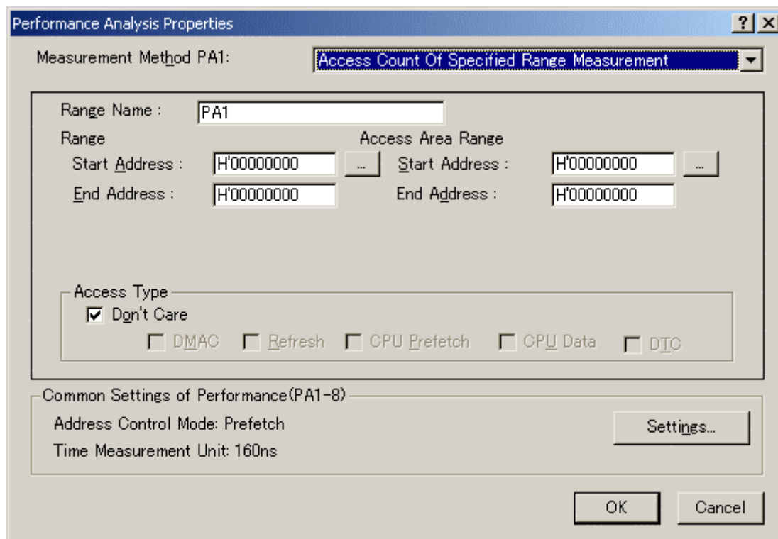
図 5-64 Access Count Of Specified Range Measurement 設定
