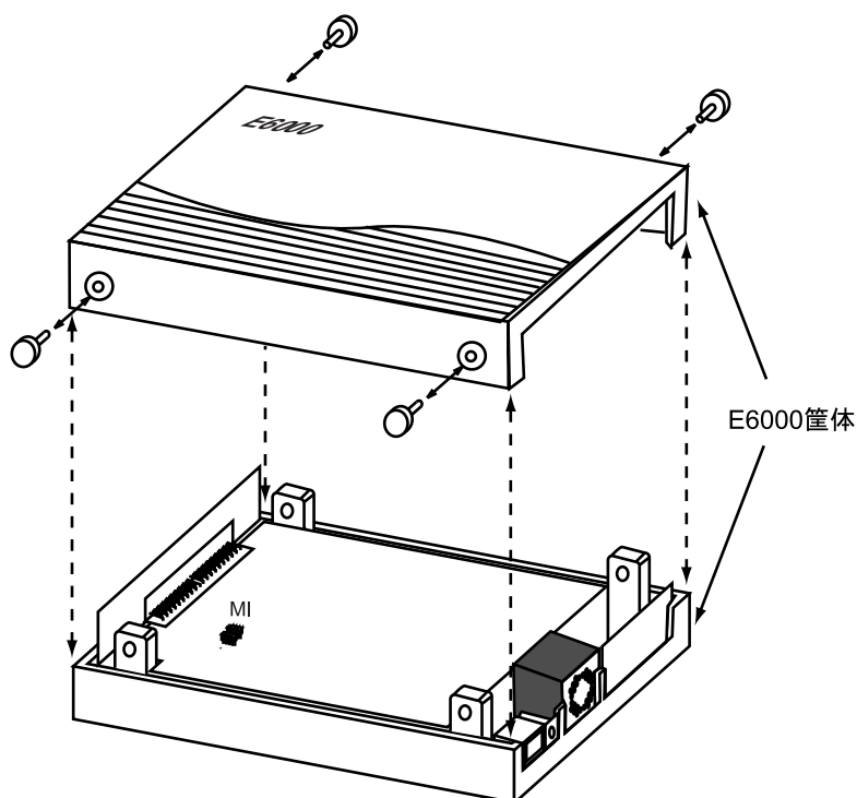
図 7-5 E6000 エミュレータ筐体の取り外し、取り付け方法
