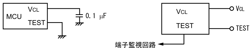
図 7-4 V CL 、TEST 信号回路
