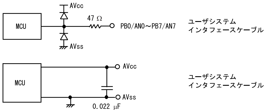
図 7-3 PB0-PB7、AVcc、AVss 信号回路
