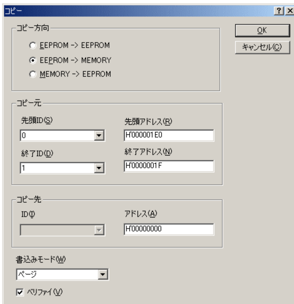
図 8-8 コピーダイアログボックス (EEPROM MEMORY)
