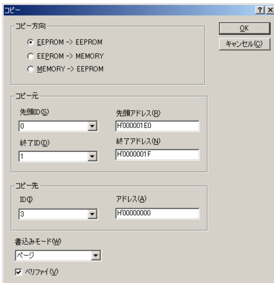
図 8-7 コピーダイアログボックス (EEPROM EEPROM)
