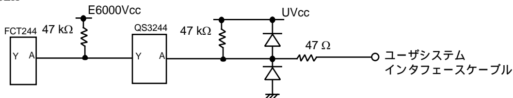
図 7-2 CLK 信号回路
