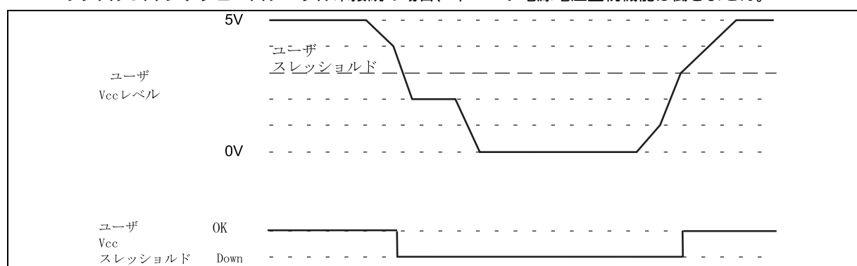
図 2-7 ユーザシステムと E6000 との Vcc の関係
