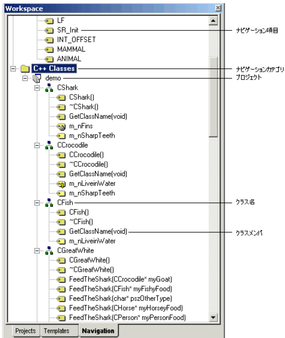
図 13.1: [Navigation]ビュー
