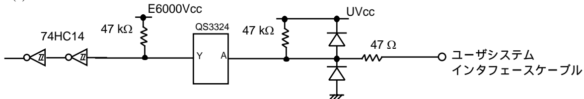
図 7-3 RESET 信号回路
