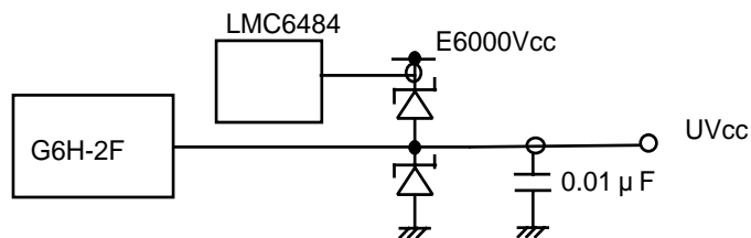
図 7-1 Vcc 信号回路
