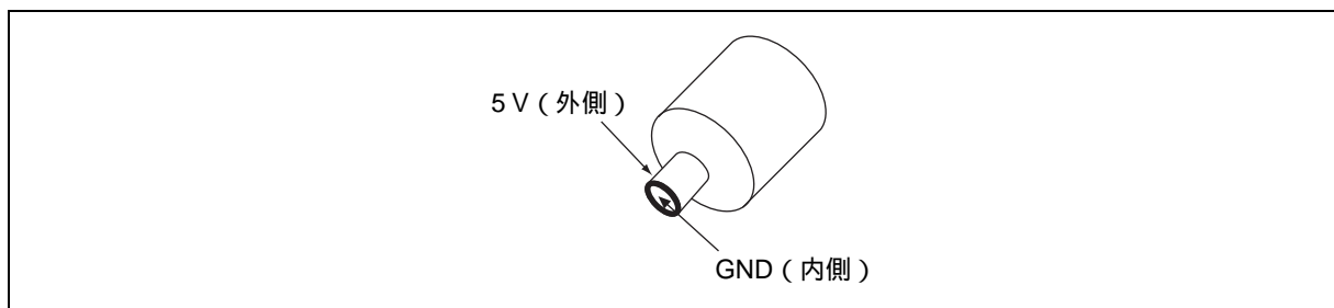
図 2-4 電源プラグ
