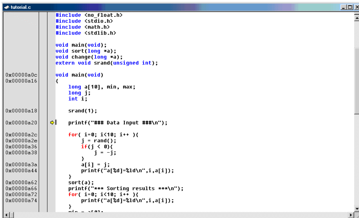
図 4.16: Editor カラム
