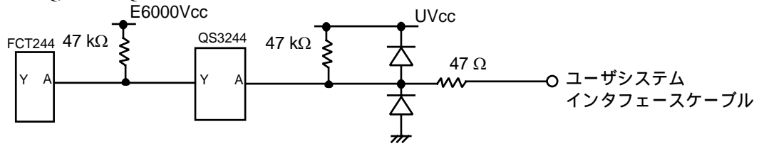
図 7-4 I/O-1/IRQ, I/O-2/IRQ 信号回路
