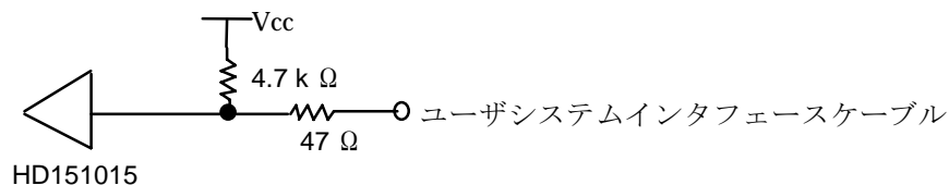
図 7-69 OSC1、X1
