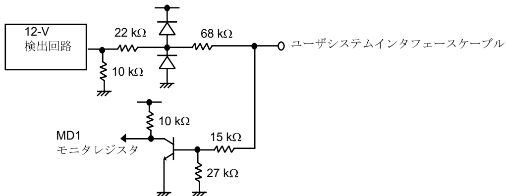
図 7-4 MD1
