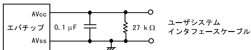
図 7-77 AVcc、AVss
