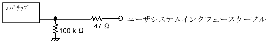
図 7-64 P20 ~ P27
