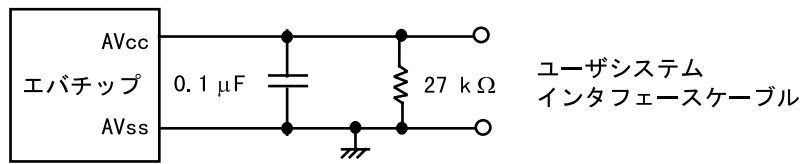
図 7-36 AVcc、AVss
