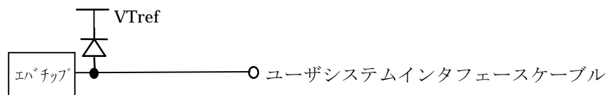
図 7-66 TONED、TONEM
