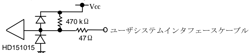
図 7-74 RESET、TEST
