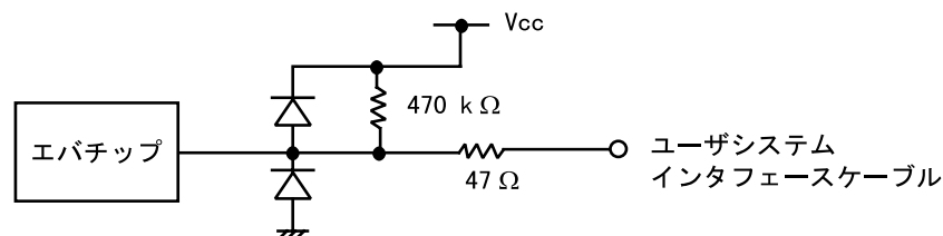
図 7-59 ユーザインタフェース信号回路
