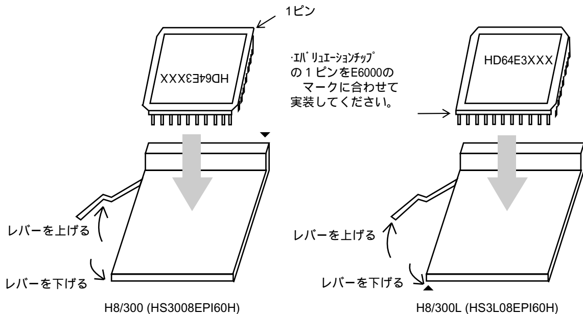
図 7-1 エミュレーションチップの実装方法
