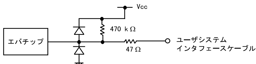
図 7-51 ユーザインタフェース信号回路
