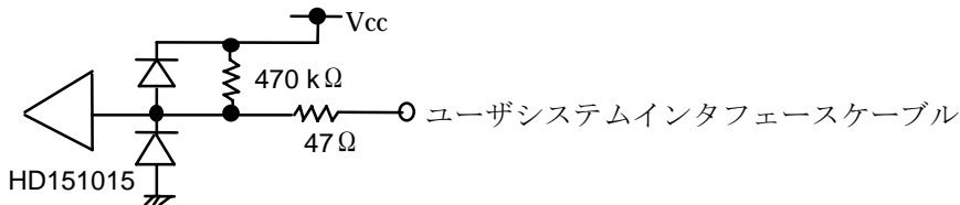
図 7-31 \overline{\text{RES}} 、NMI、MD0
