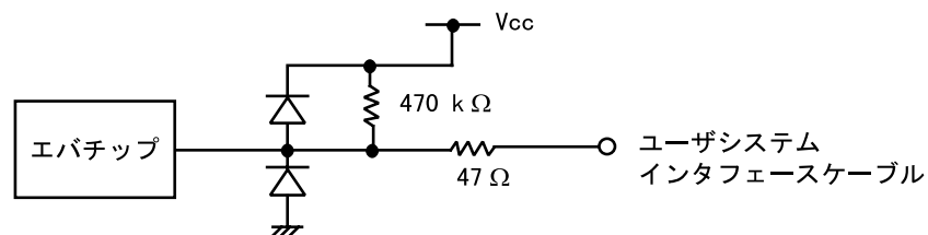
図 7-37 ユーザインタフェース信号回路
