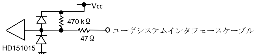
図 7-53 RES、TEST、MD0
