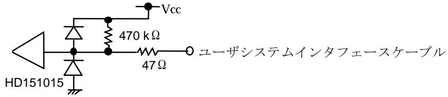
図 7-40 EXTAL
