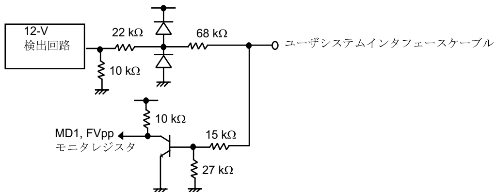
図 7-39 MD1、FVpp
