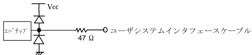
図 7-65 V1、V2、V3
