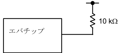
図 7-41 \overline{\text{STBY}}
