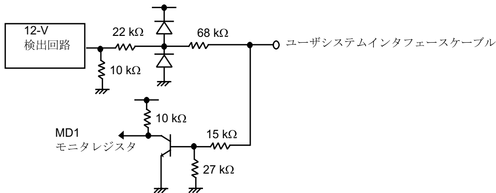
図 7-32 MD1
