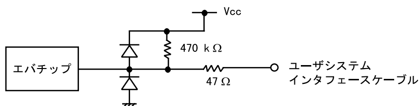
図 7-73 ユーザインタフェース信号回路
