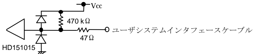
図 7-10 RES、NMI、MD0
