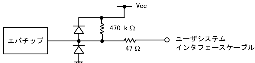
図 7-16 ユーザインタフェース信号回路
