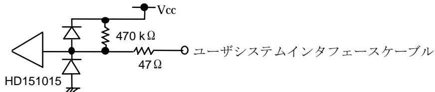
図 7-68 \overline{\text{RES}} 、 \overline{\text{TEST}} 、 \overline{\text{NMI}}
