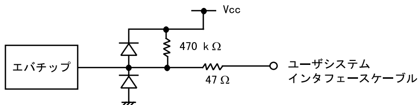
図 7-23 ユーザインタフェース信号回路
