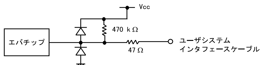
図 7-2 ユーザインタフェース信号回路
