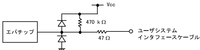
図 7-30 ユーザインタフェース信号回路
