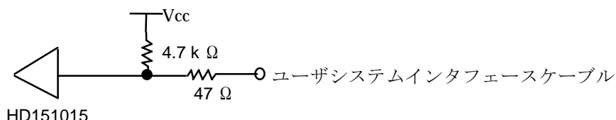
図 7-75 OSC1、X1
