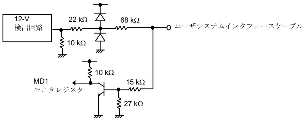
図 7-25 MD1
