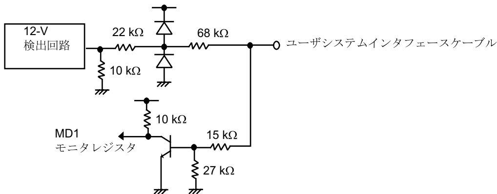
図 7-18 MD1
