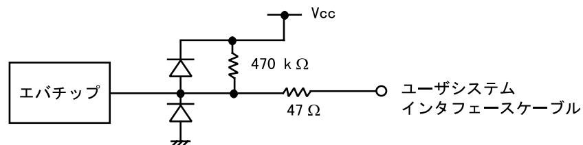
図 7-44 ユーザインタフェース信号回路
