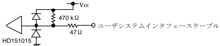
図 7-38 \overline{\text{RES}} 、NMI、MD0
