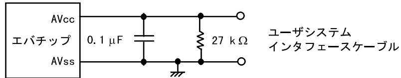
図 7-71 AVcc、AVss
