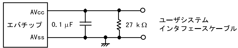
図 7-50 AVcc、AVss
