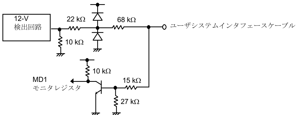
図 7-46 MD1
