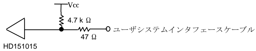
図 7-54 OSC1、X1
