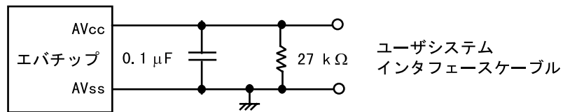
図 7-8 AVcc、AVss
