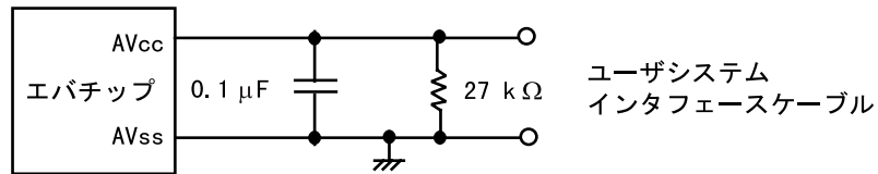
図 7-56 AVcc、AVss
