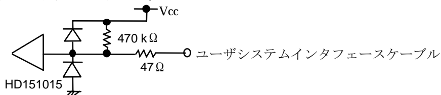
図 7-60 \overline{\text{RES}} 、TEST、 \overline{\text{NMI}}
