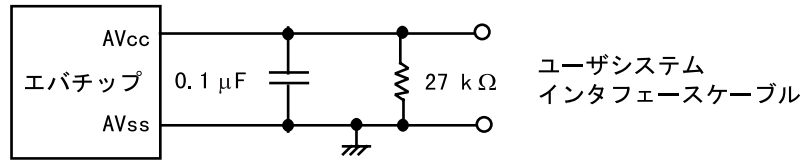
図 7-63 AVcc、AVss、AVref、VTref
