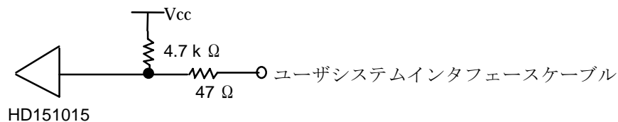
図 7-61 OSC1、X1
