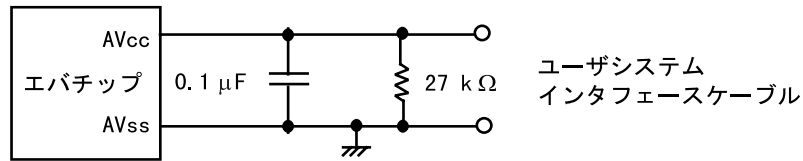
図 7-15 AVcc、AVss
