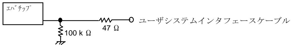
図 7-57 P20 ~ P27
