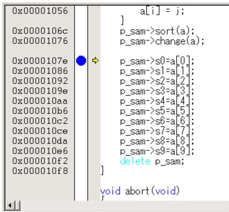
図 6.36 実行停止時の[Source]ウィンドウ (Break Condition 1)
