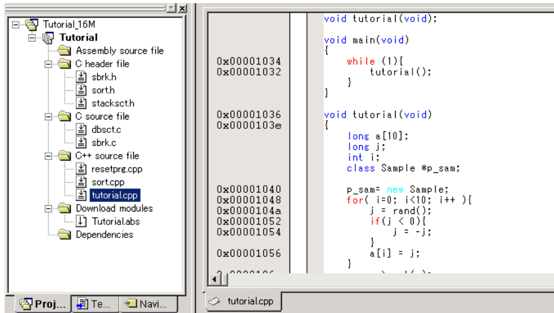
図 6.5 [Source]ウィンドウ (ソースプログラムの表示)
