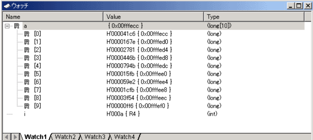
図 6.19 [ウォッチ]ウィンドウ (配列要素の表示)
