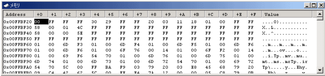
図 6.3 [メモリ]ウィンドウ
