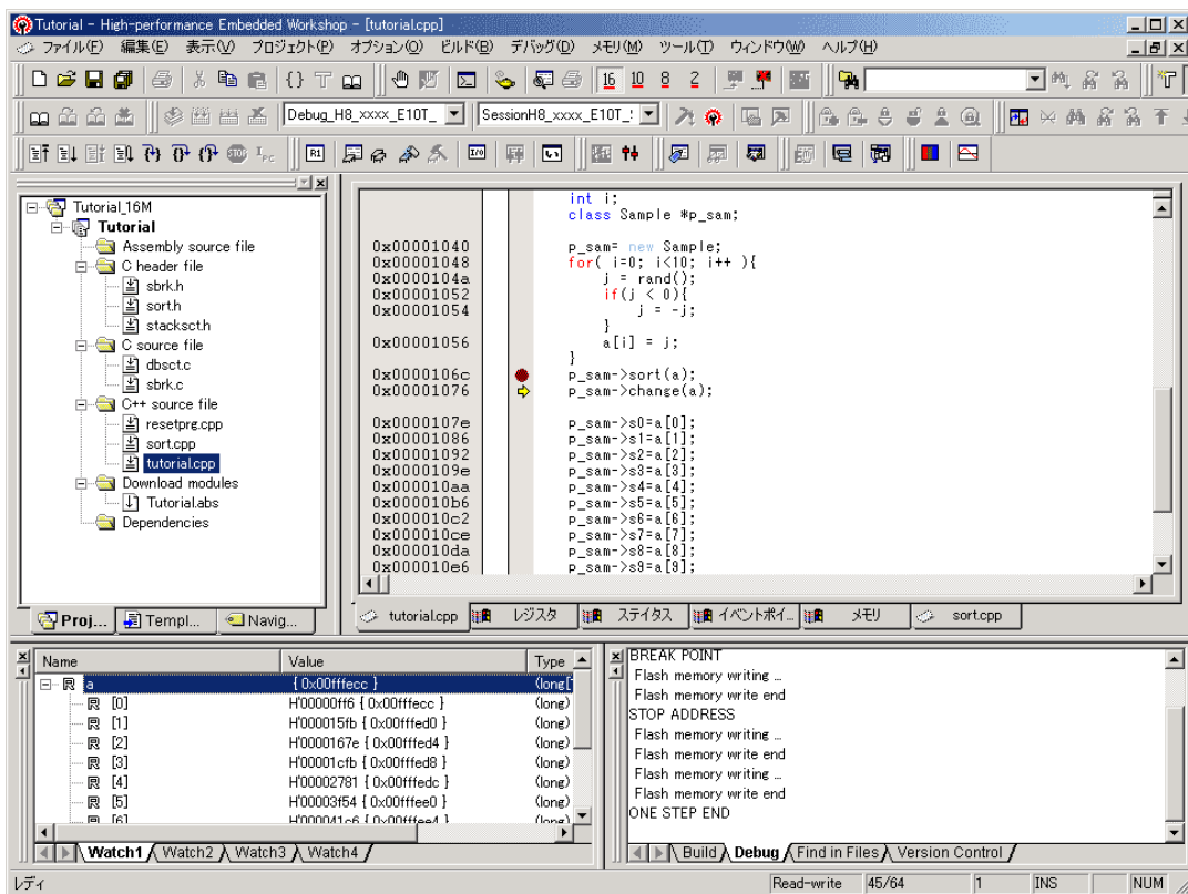
図 6.23 [HEW]ウィンドウ (ステップアウト)
