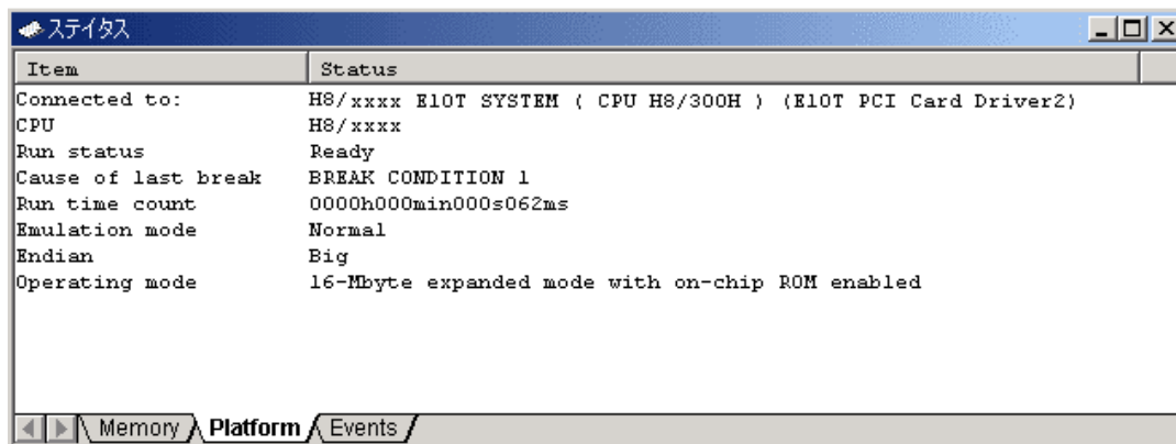
図 6.37 [ステータス]ウィンドウの表示内容 (Break Condition 1)
