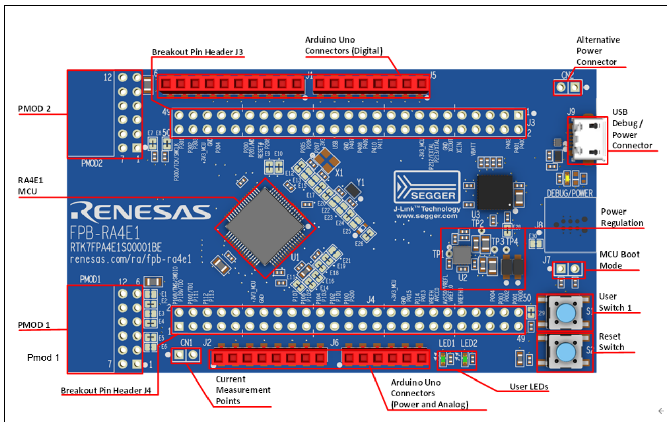
図 1 FPB-RA4E1 ボード (上面)
