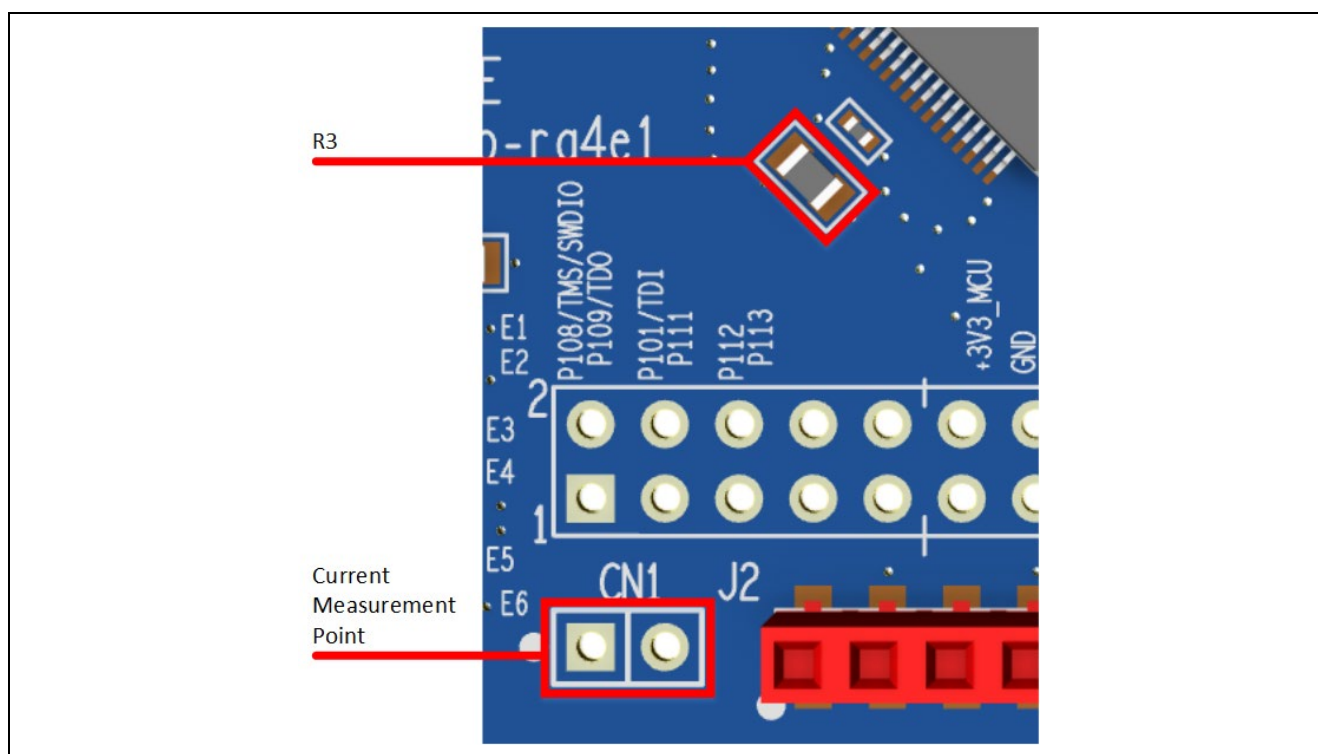
図 19 RA MCU +3.3 V 電流測定テストポイントと R3
