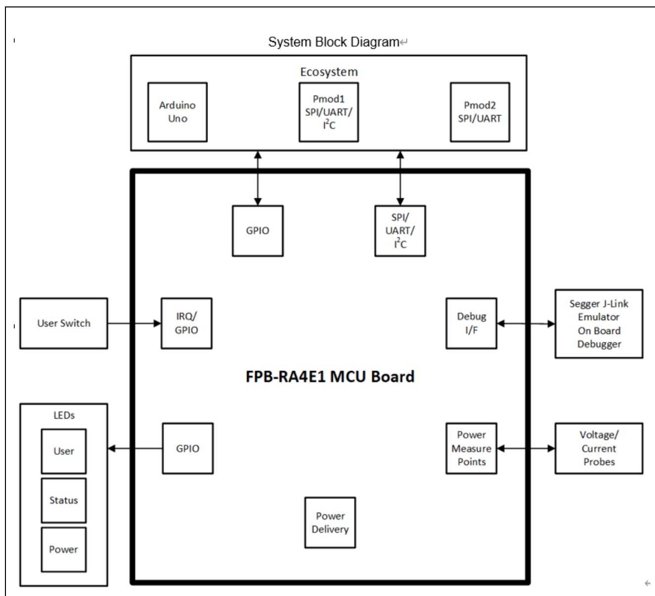
図 4 FPB-RA4E1 ボードブロック図
