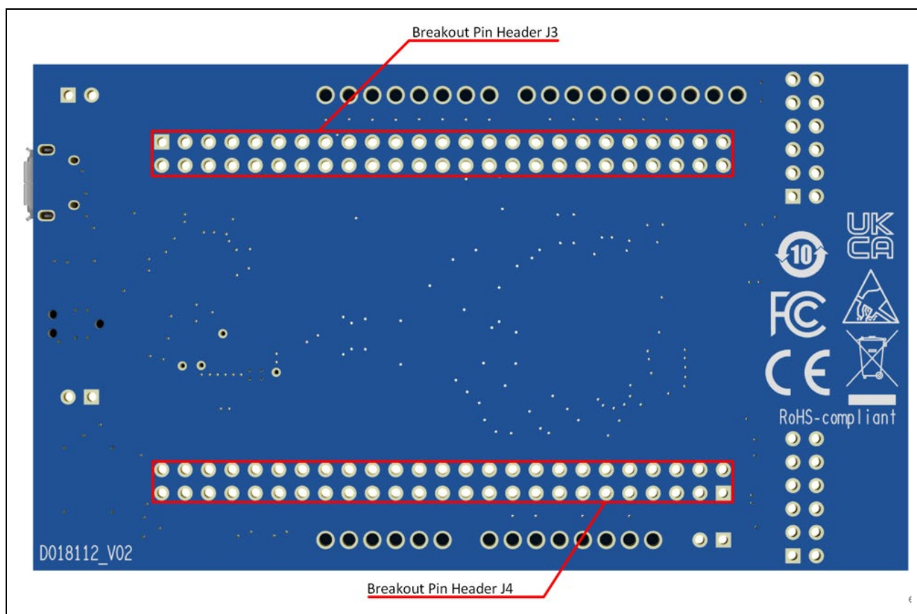
図 2 FPB-RA4E1 ボード (裏面)
