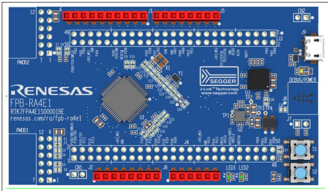
図 3 FPB-RA4E1 v1 評価ボード
