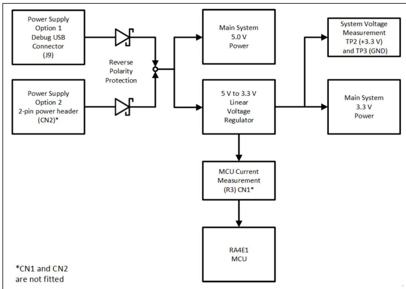
図 6 電源供給のオプション
