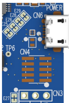
図 7 FPB-RA4E1 デバッグインタフェース
