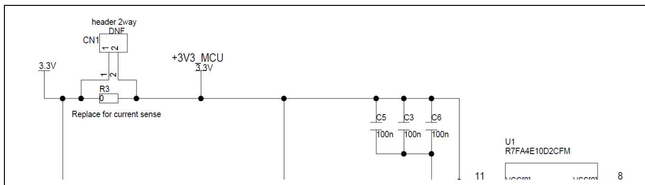
図 18 RA MCU +3.3 V 電流測定回路
