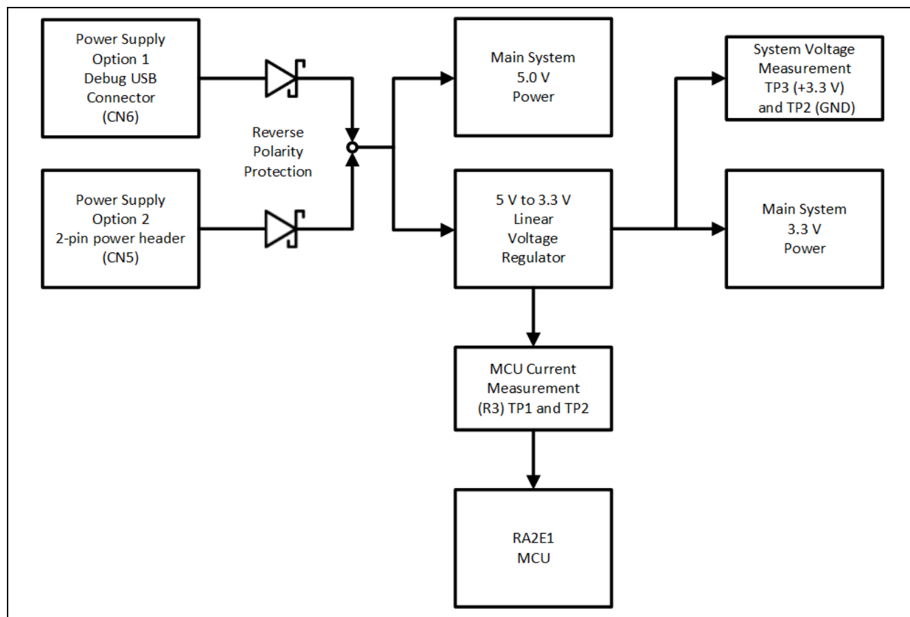
図6 電源供給のオプション
