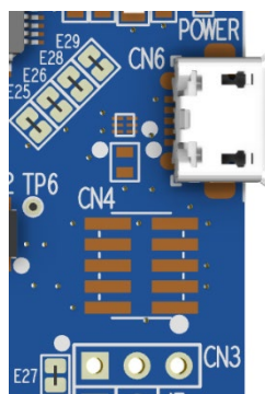
図 7 FPB-RA2E1 デバッグインタフェース
