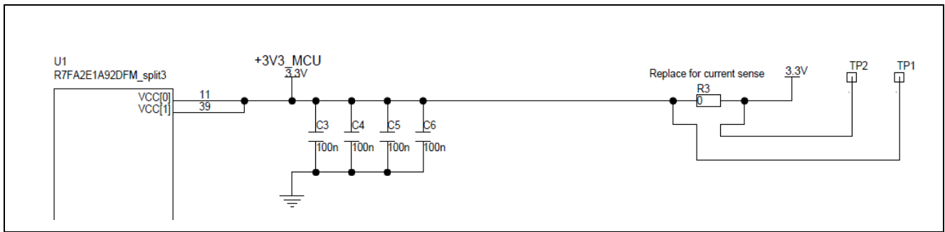
図 18 RA MCU +3.3 V 電流測定回路
