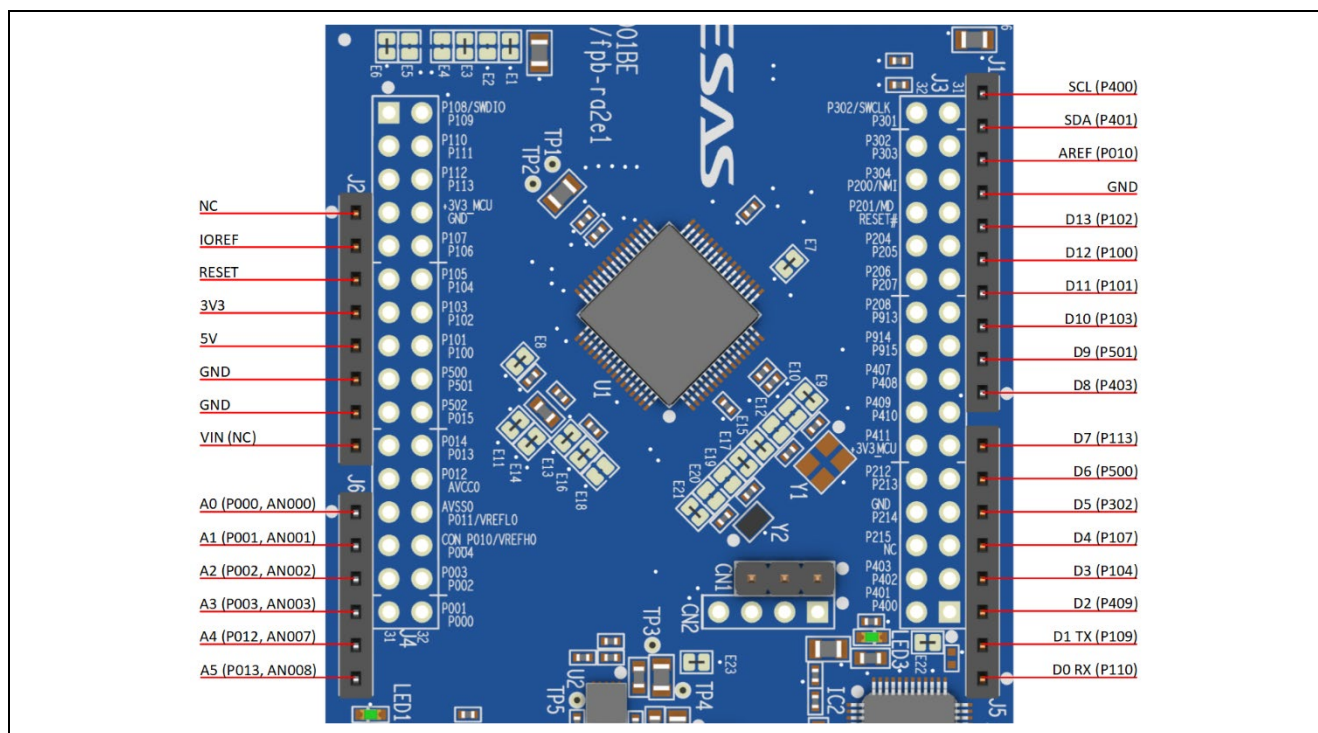
図 12 Arduino Uno コネクタ
