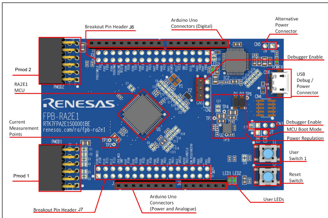
図 1 FPB-RA2E1 ボード (上面)
