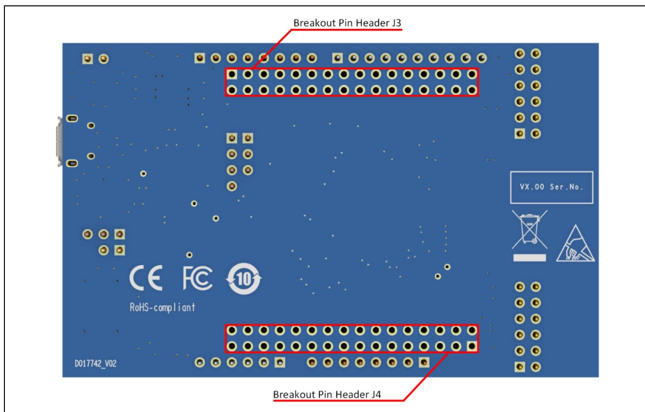
図 2 FPB-RA2E1 ボード (裏面)
