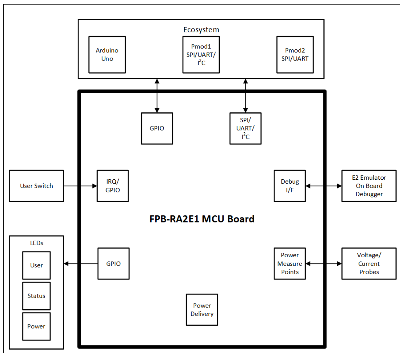
図 4 FPB-RA2E1 ボードブロック図
