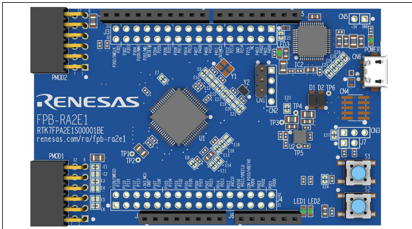
図 3 FPB-RA2E1 v1 評価ボード
