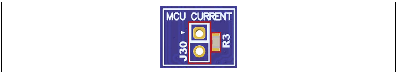
図 21 RA0E3 VCC 電流測定ポイント J30 と R3 (表面)
