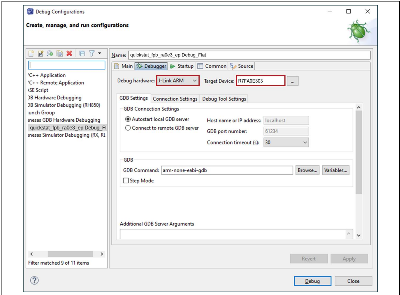
図 9 e 2 studio デバッグ設定
