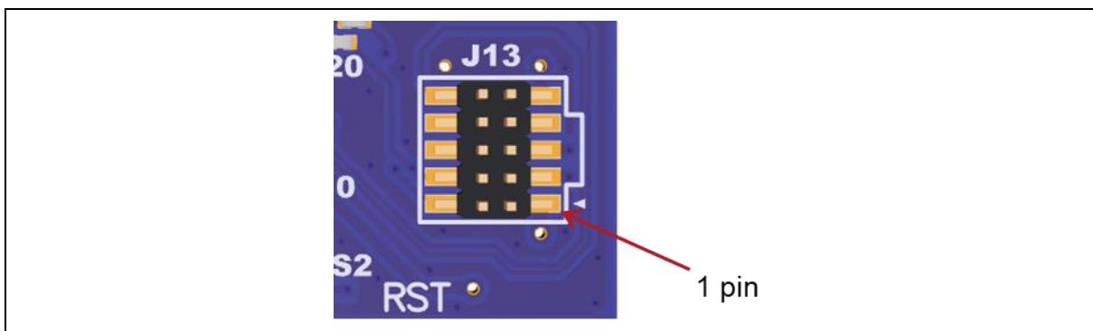
図 22 J13-1 の位置 (表面)
