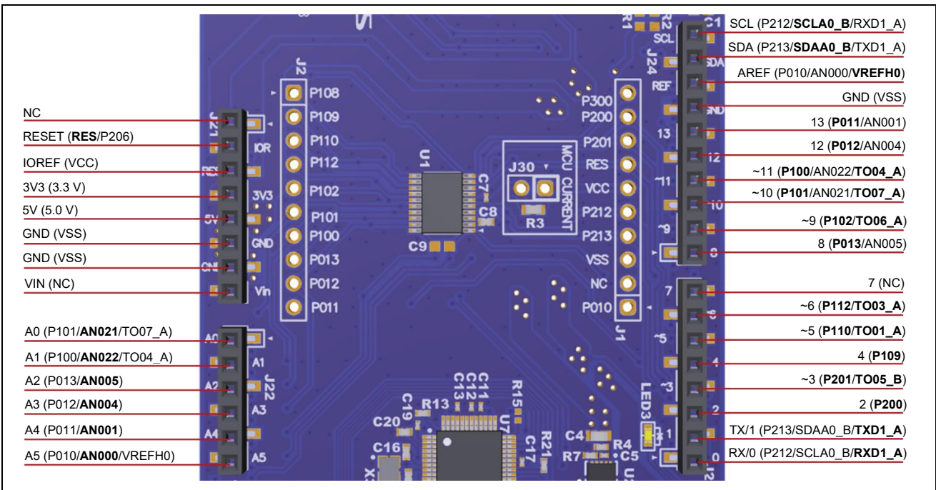
図 13 Arduino® コネクタ (表面)
