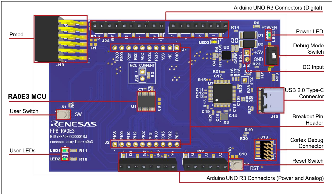
図 1 FPB-RA0E3 ボード (表面)
