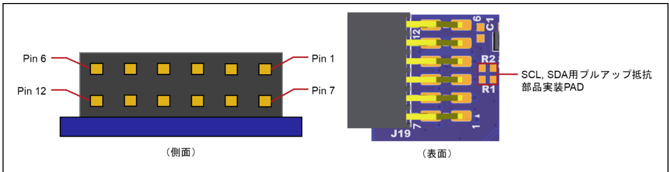
図 11 Pmod コネクタピンレイアウト
