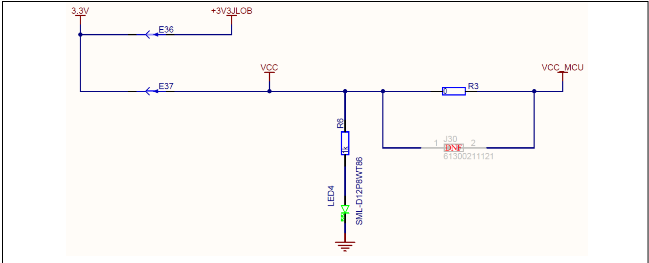
図 20 RA0E3 VCC 電流測定回路
