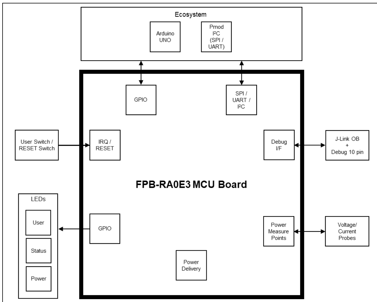
図 4 FPB-RA0E3 ボードブロック図
