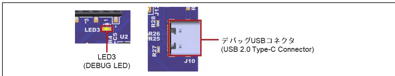
図 8 FPB-RA0E3 デバッグインタフェース (表面)
