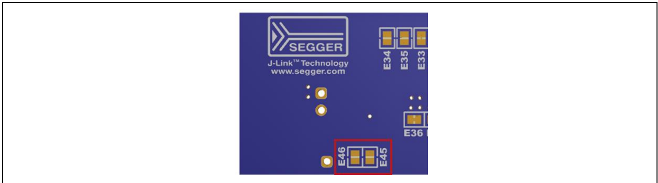
図 10 VCOM 用はんだジャンパ(裏面)
