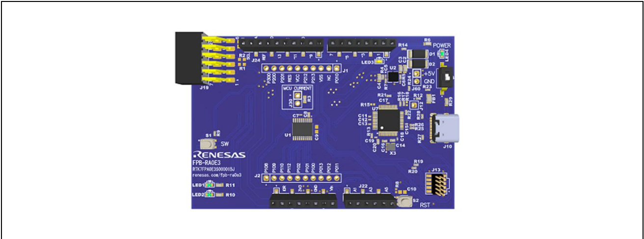
図 3 FPB-RA0E3 v1 評価キット構成
