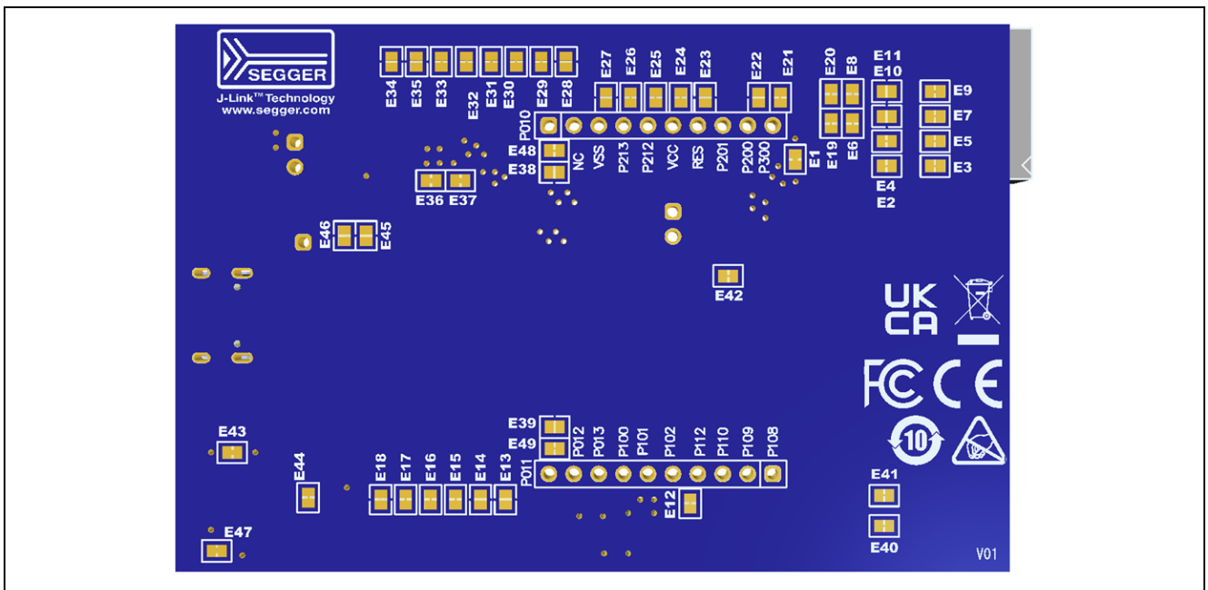
図 2 FPB-RA0E3 ボード (裏面)
