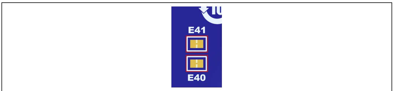
図 15 ユーザ LED 用 Jumper Trace Cut(ショート) (裏面)
