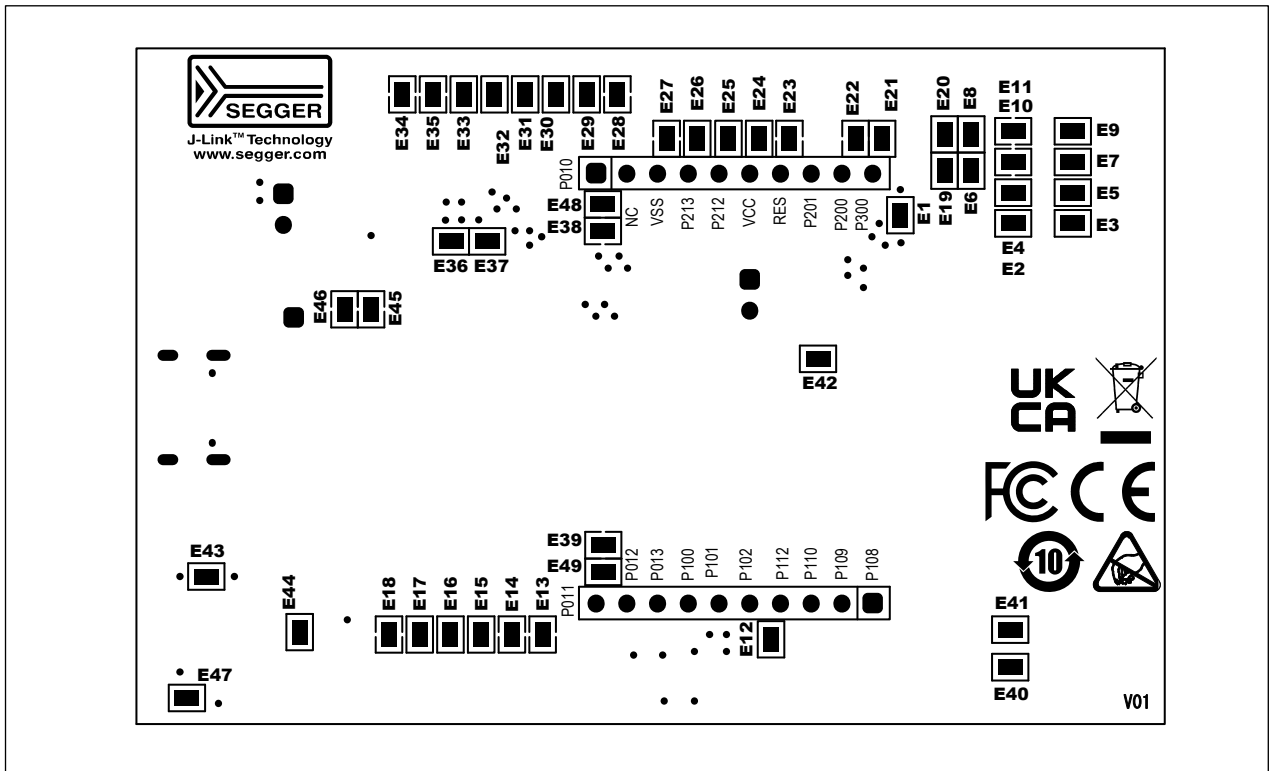
図 24 FPB-RA0E3 ボード下部部品配置図(裏面)
