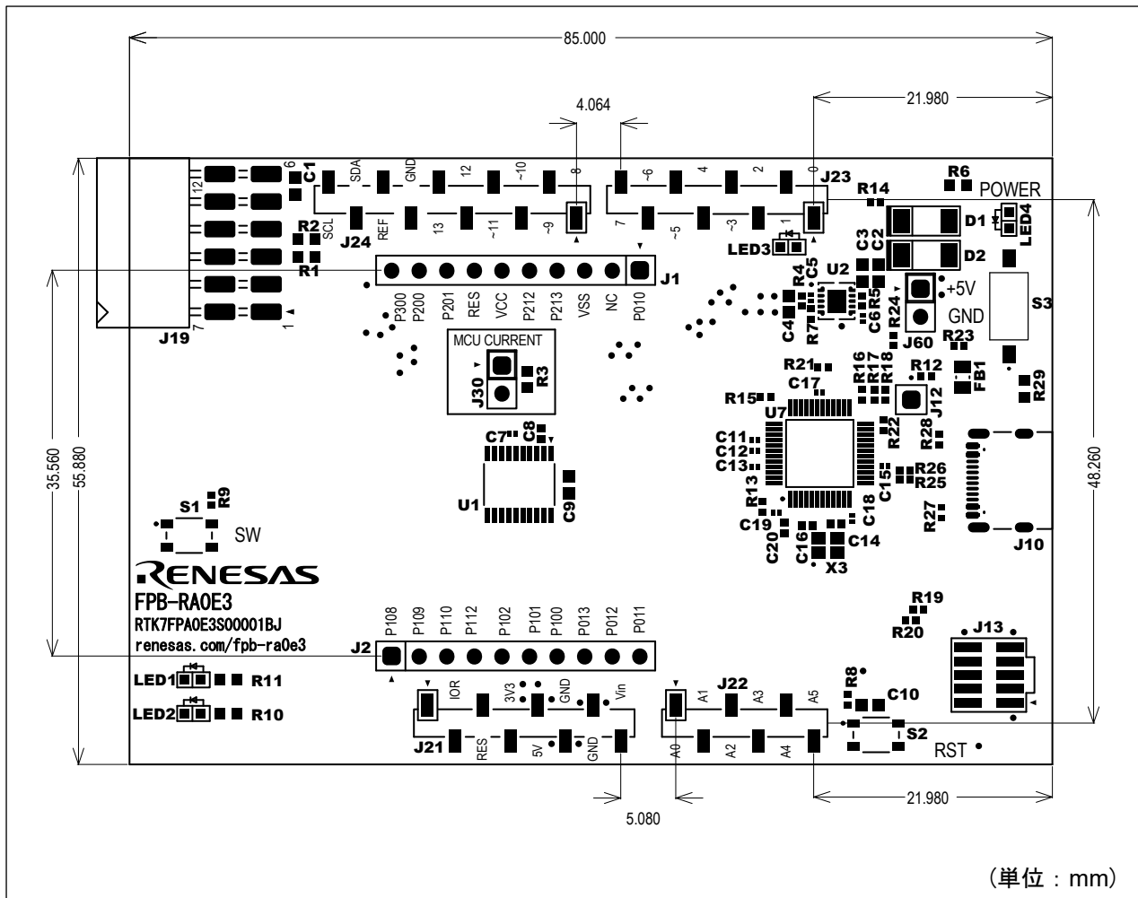
図 23 FPB-RA0E3 ボード部品配置図(表面)
