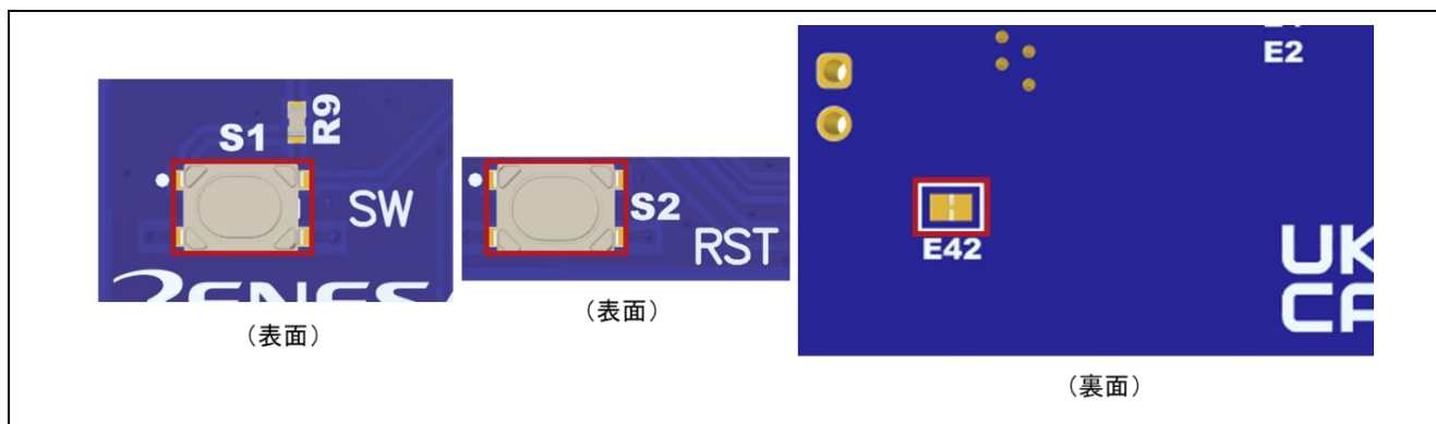
図 18 ユーザスイッチ (S1) とリセットスイッチ (S2) と Jumper Trace Cut (ショート) (E42)
