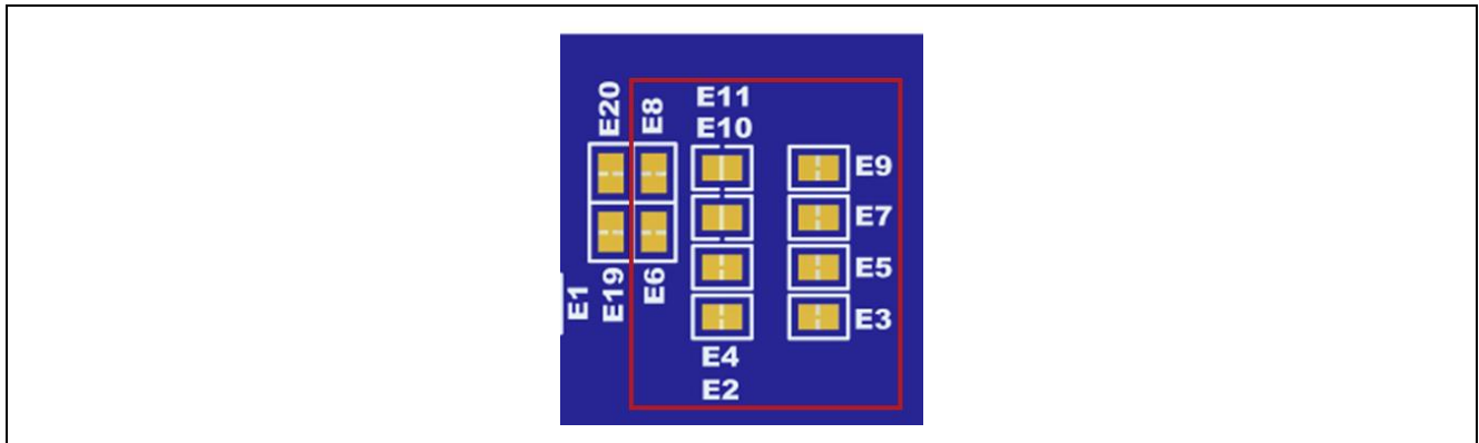
図 12 Pmod はんだジャンパ (裏面)
