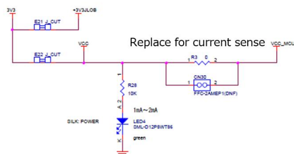
図 24 RA MCU +3.3 V 電流測定回路
