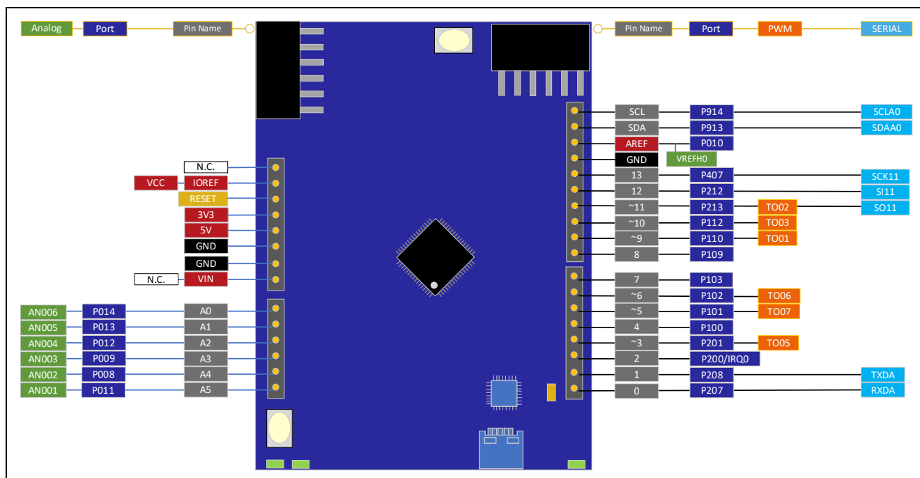
図 15 Arduino Uno コネクタ
