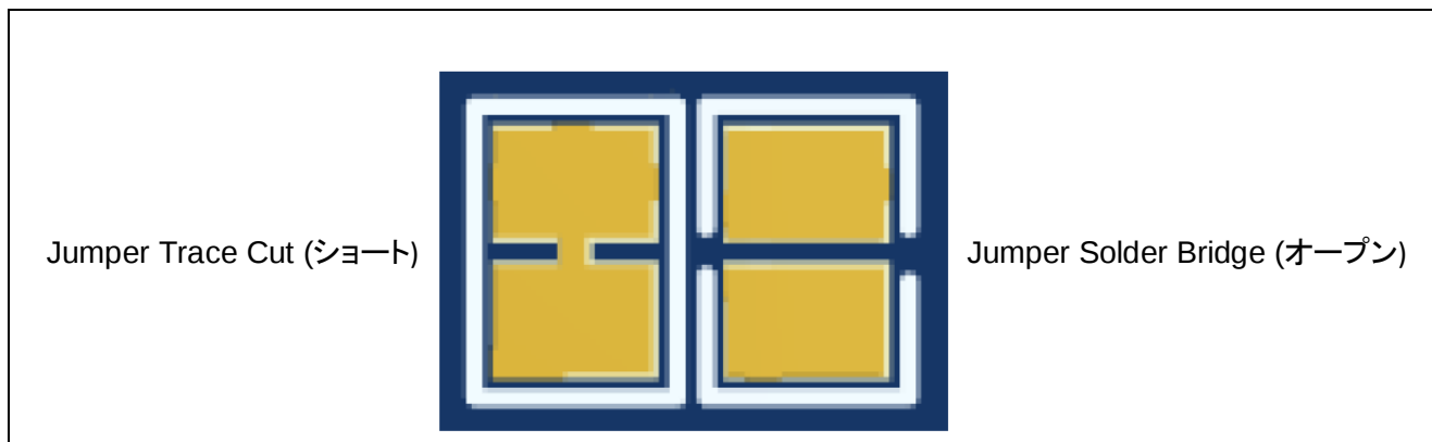
図 5 はんだジャンパ
