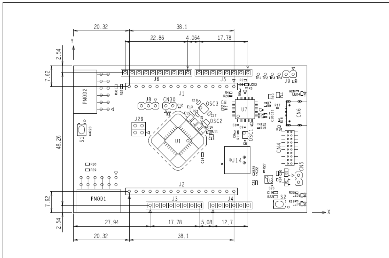
図 27 寸法図
