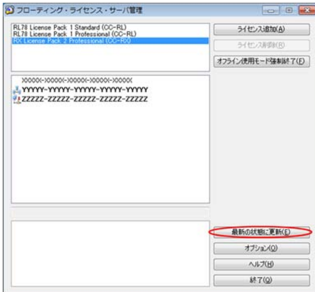
図 2.20 使用状況の表示を更新
