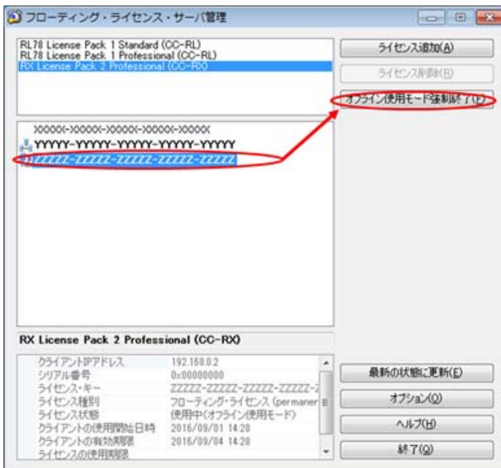
図 2.24 オフライン使用モードを強制終了する
