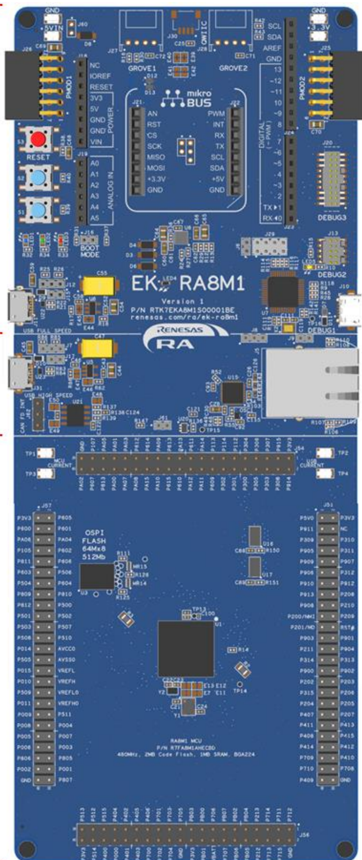
図 4. EK-RA8M1 ボード機能エリアの定義
