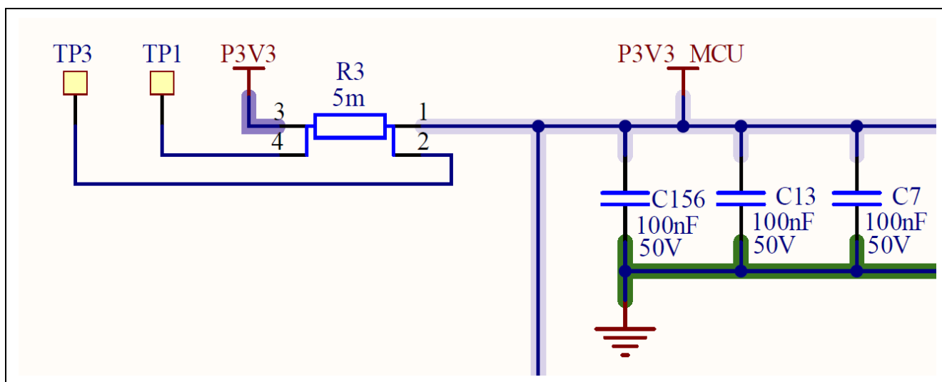
図 33. RA +3.3 V 電流測定回路
