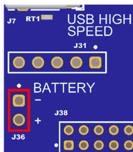
図 10. VBATT 電源 (J36) の位置
