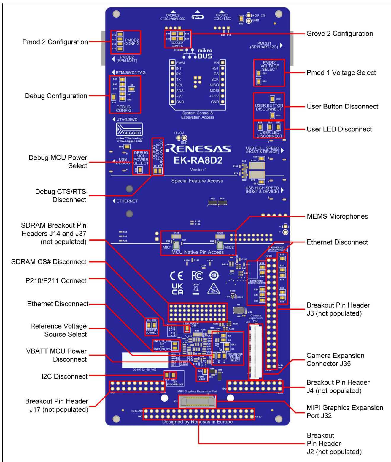
図 2. EK-RA8D2 ボード表面
