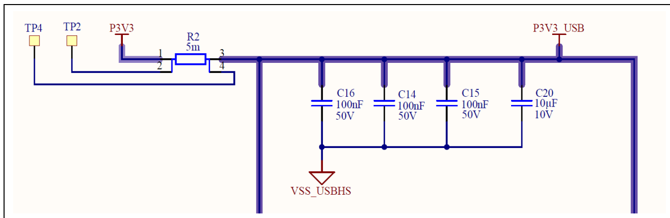
図 32. RA USB 電流測定回路
