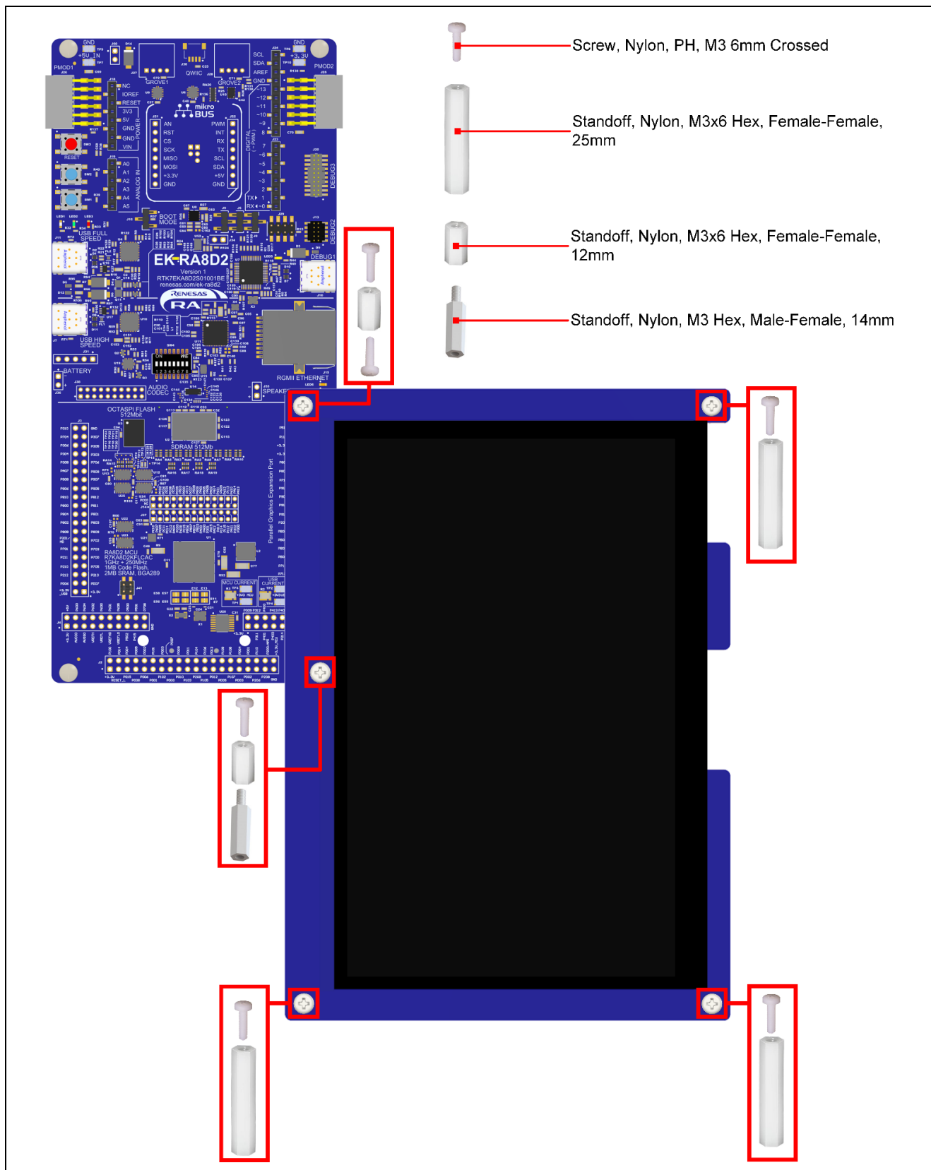
図 36. EK-RA8D2 ボードに接続されたパラレルグラフィックス拡張ボード 1
