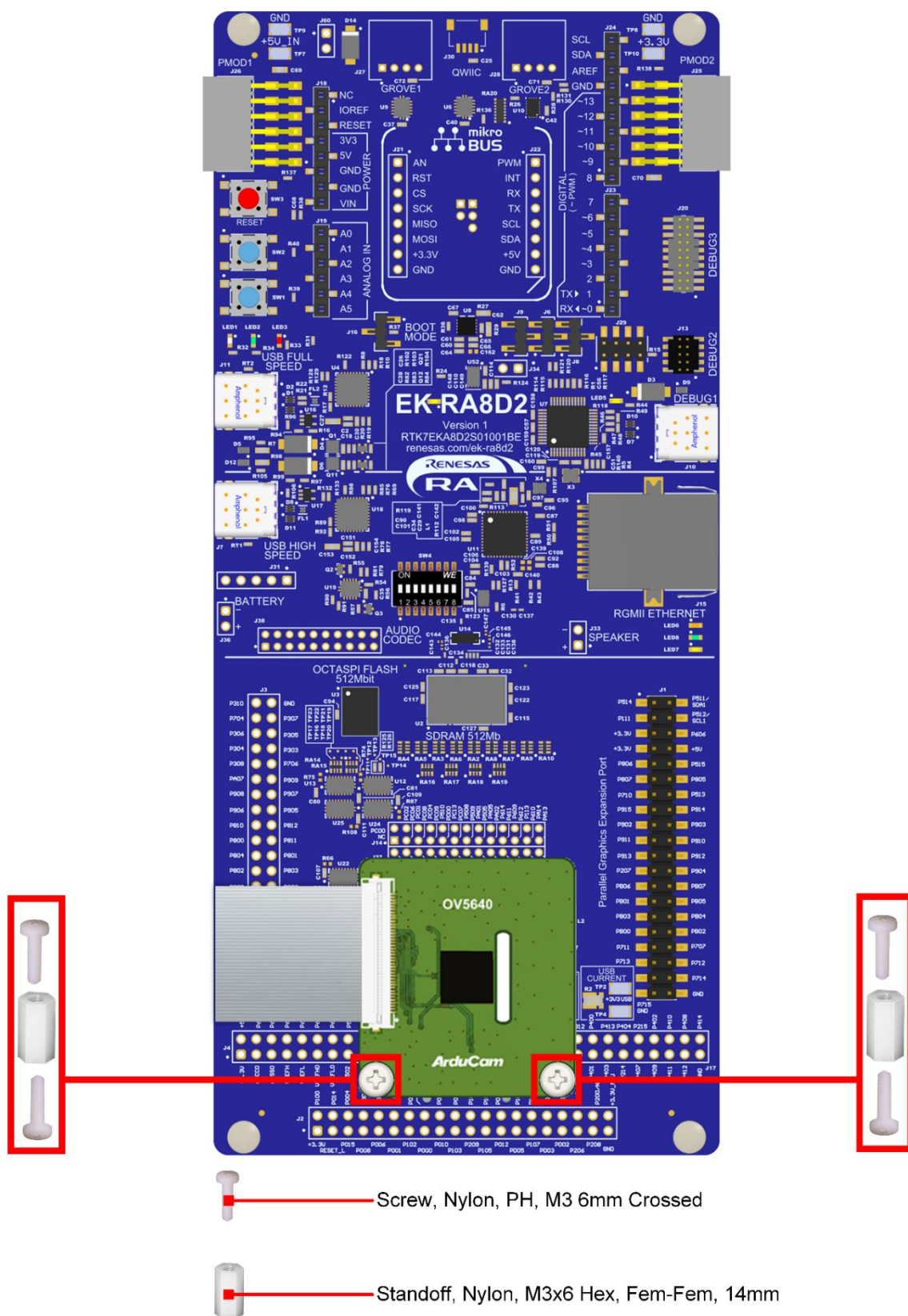
図 40. EK-RA8D2 ボードに接続されたカメラ拡張ボード
