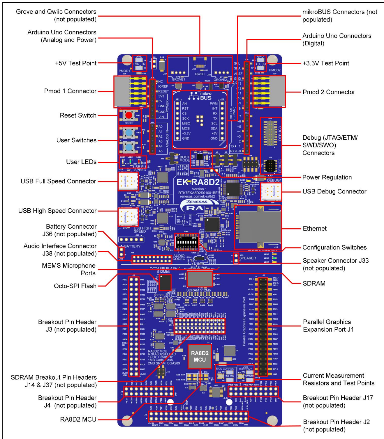
図 1. EK-RA8D2 ボード表面
