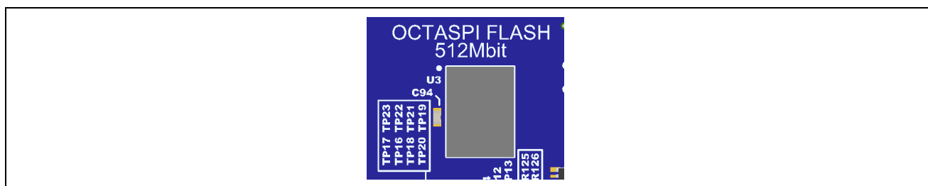
図 27. Octo-SPI フラッシュ (シルクスクリーン文字に“OCTASPI”とラベル付けされている)
