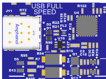
図 17. USB フルスピードコネクタ
