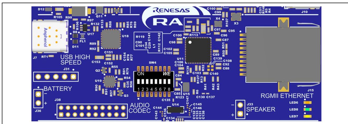
図 24. Special Feature Access エリア
