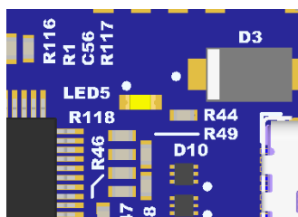
図 20. デバッグ LED
