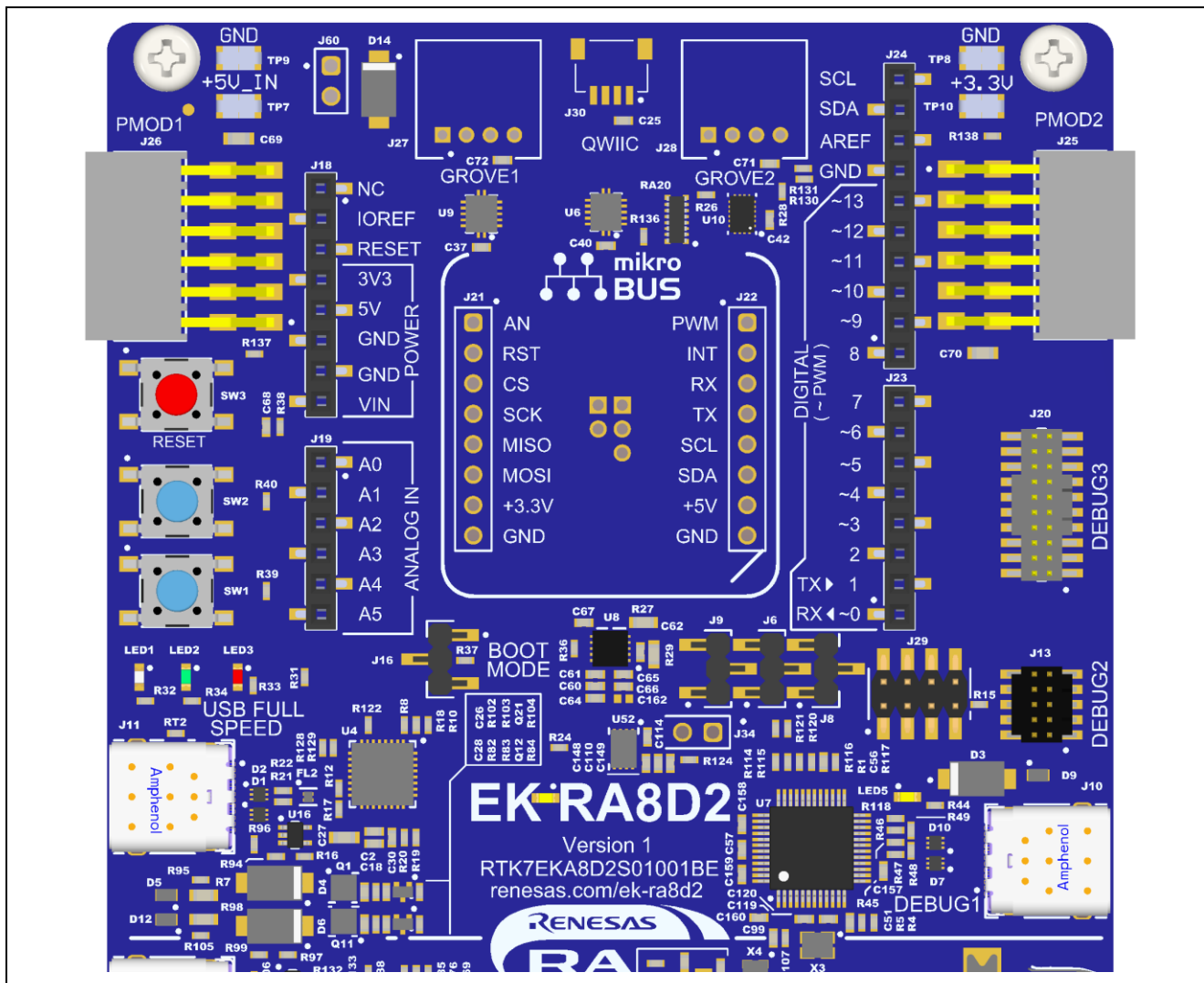
図 7. System Control and Ecosystem Access エリア
