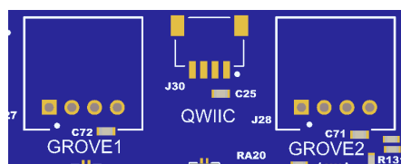
図 12. Seeed Grove®と SparkFun Qwiic®コネクタフットプリント
