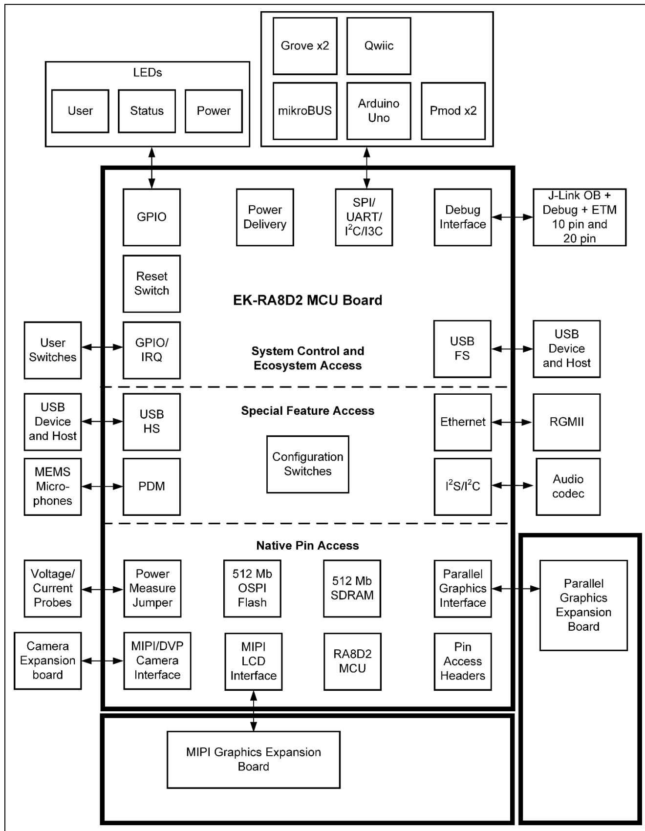
図 5. EK-RA8D2 ボードのブロック図
