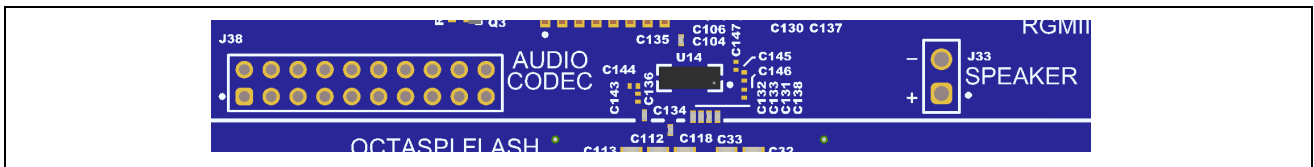
図 30. Audio CODEC(U14)、スピーカコネクタ(J33)、ピンヘッダ(J38)
