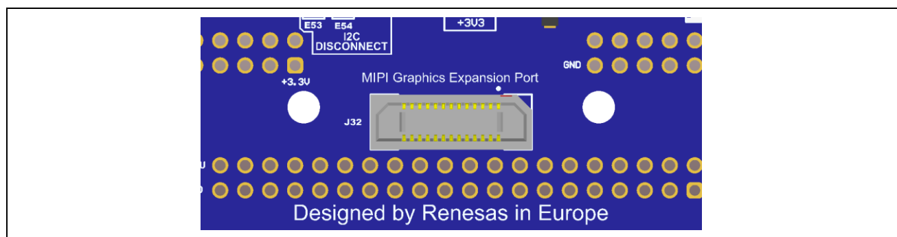
図 37. MIPI グラフィックス拡張ポート
