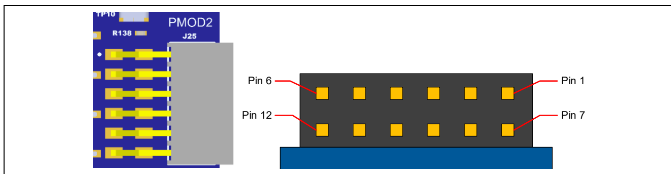
図 14. Pmod 2 コネクタ
