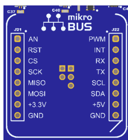
図 16. mikroBUS™コネクタ
