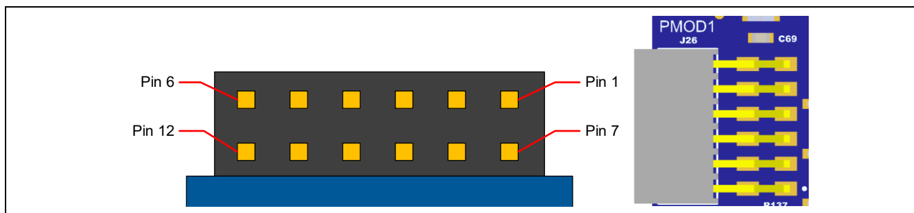
図 13. Pmod 1 コネクタ
