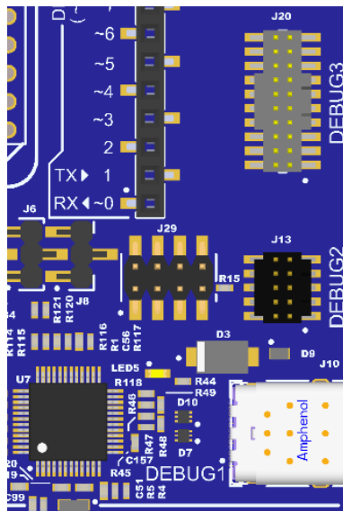
図 11. EK-RA8D2 デバッグインタフェース
