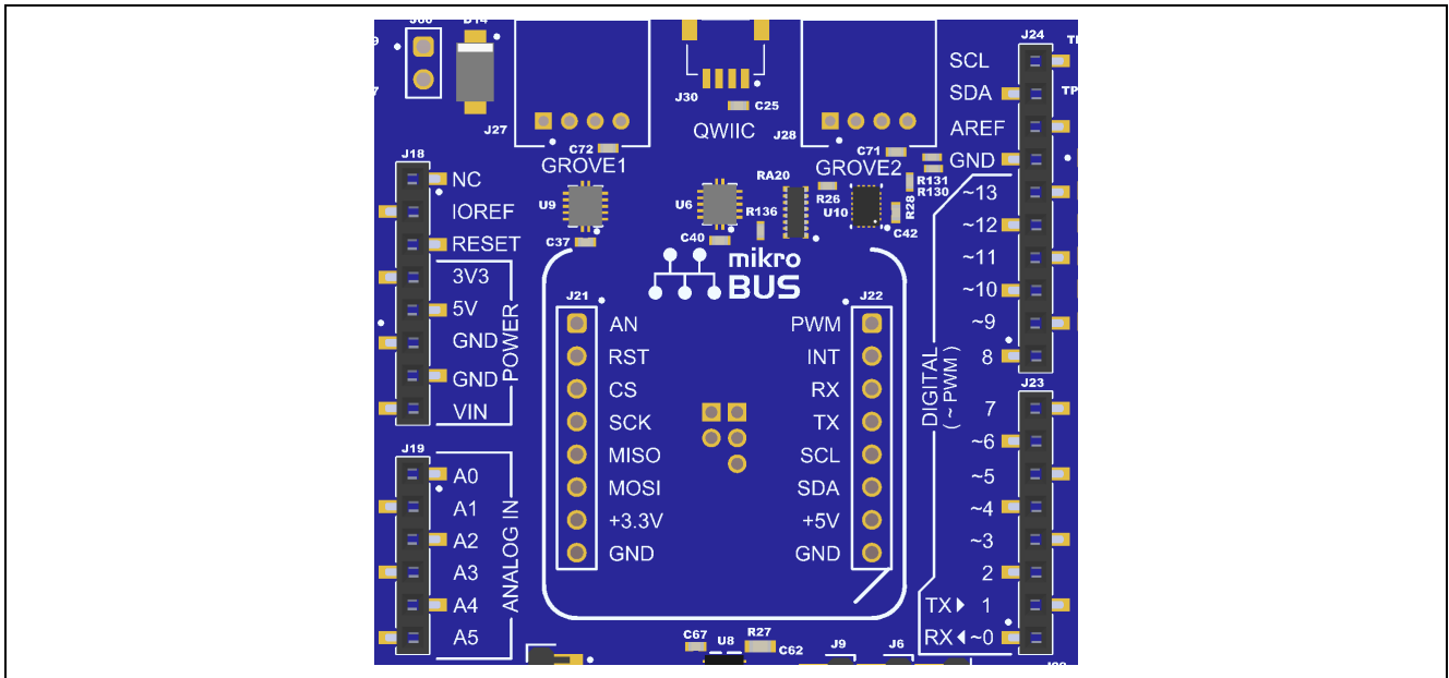
図 15. Arduino UNO コネクタ
