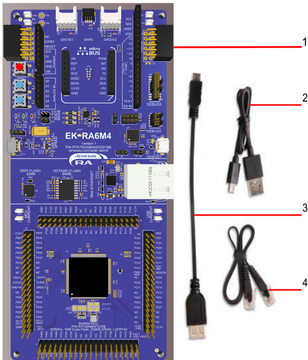
図3 EK-RA6M4 v1 評価キット構成
