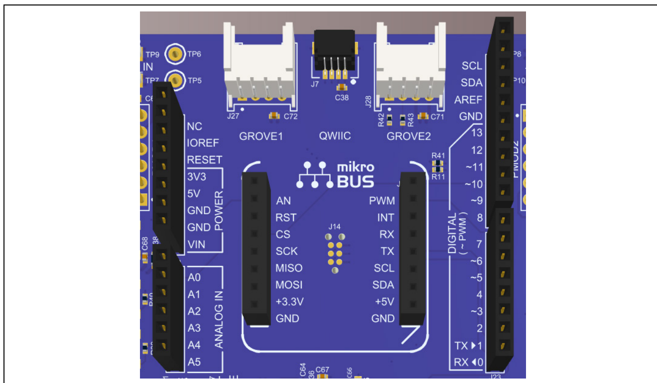
図 14 Arduino Uno コネクタ
