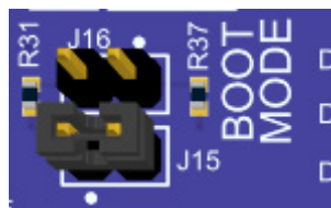
図 20 ブートモード
