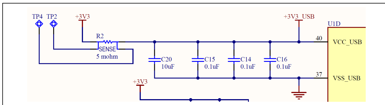
図 26 RA USB 電流測定回路
