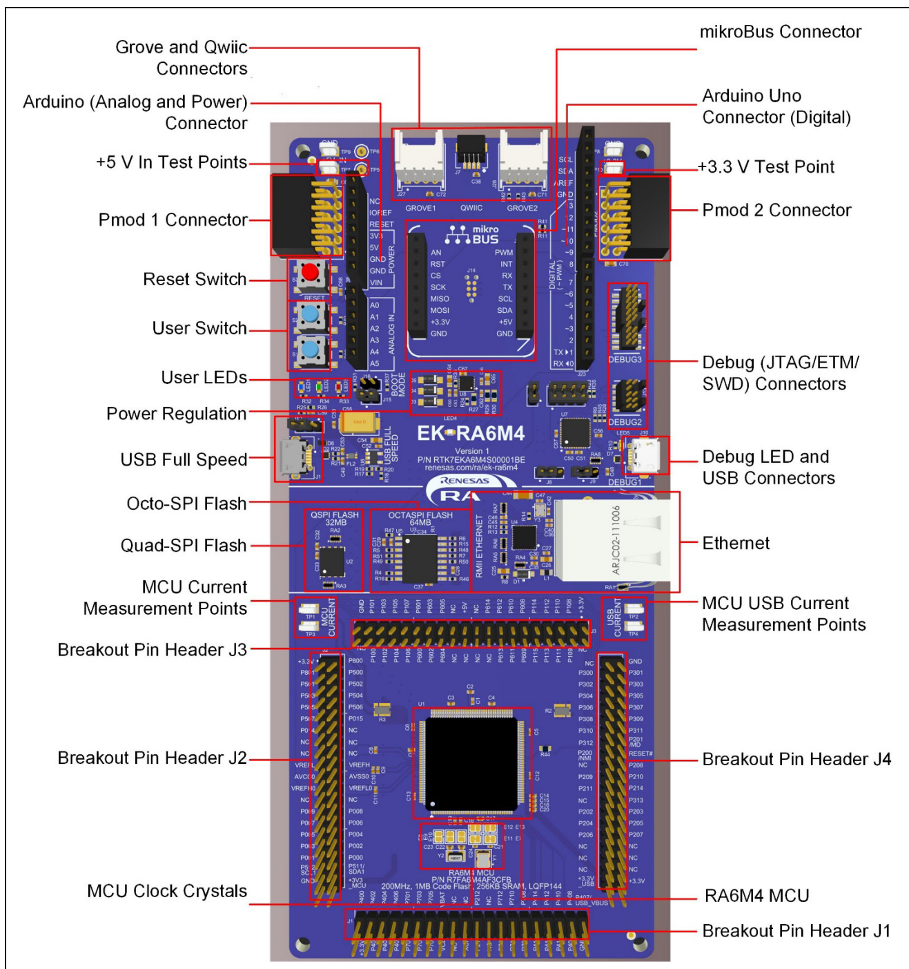
図 1 EK-RA6M4 ボード (上面)
