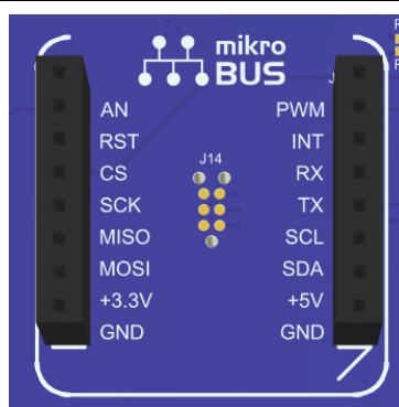
図 15 mikroBUS コネクタ
