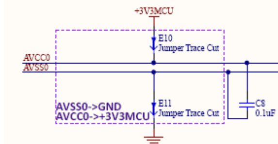
図 29 AVCC0/AVSS0 回路
