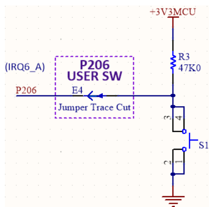
図 16 ユーザスイッチ回路
