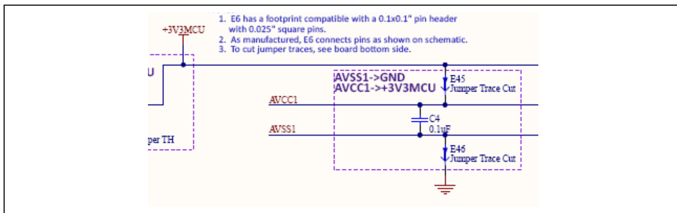
図 30 AVCC1/AVSS1 回路
