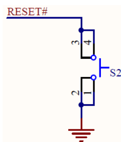
図 18 リセットスイッチ回路
