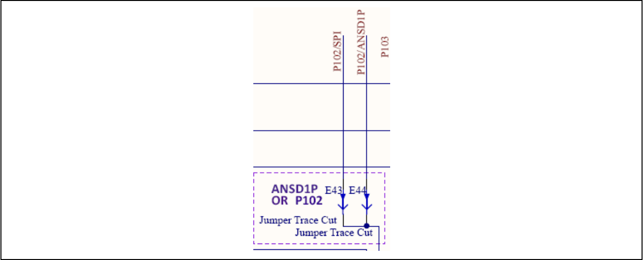
図 35 P102/SPI/ANSD1P 回路
