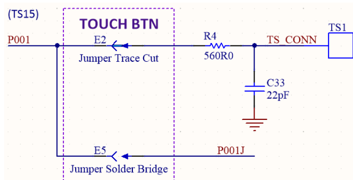
図 20 静電容量式タッチボタン回路
