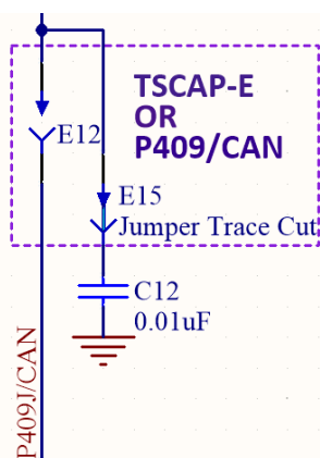
図 21 静電容量式タッチ TSCAP 回路
