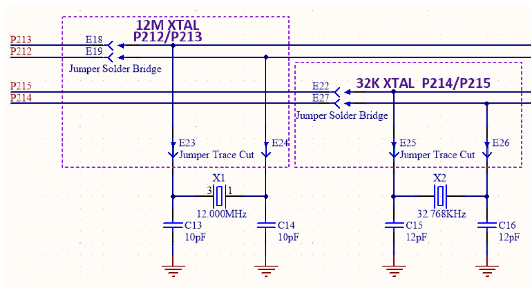
図 25 水晶クロックソース
