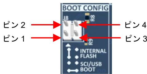
図 28 ブート設定ジャンパ J8
