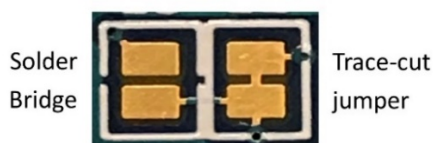
図4 はんだジャンパ
