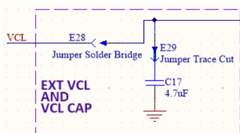
図 31 外部コンデンサと VCL 回路の接続
