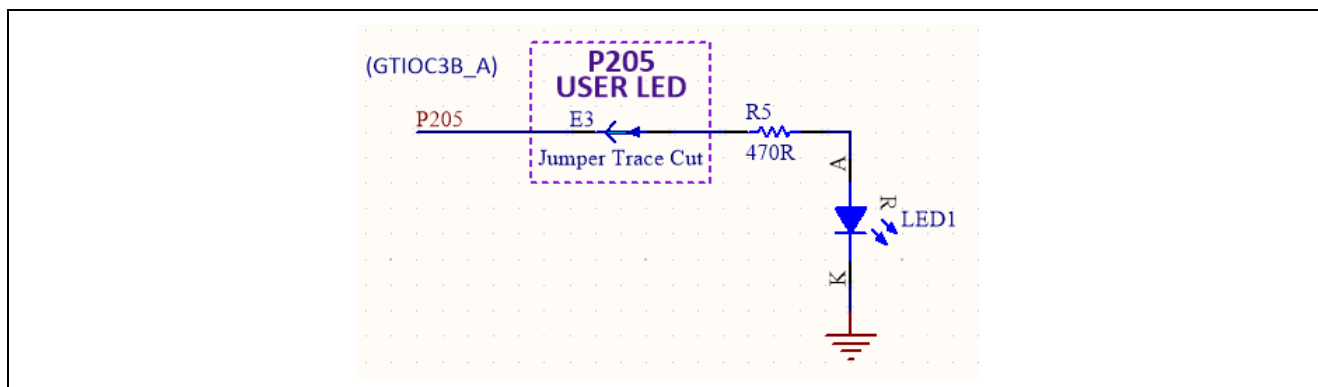
図 15 LED1 制御回路
