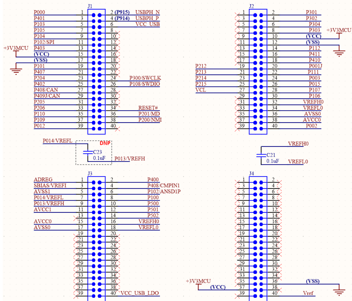
図 24 EK-RA2A1 ピンヘッダ回路
