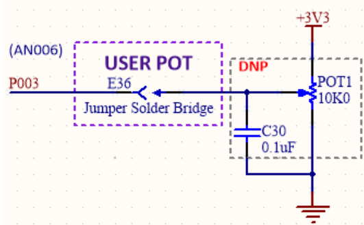
図 26 ユーザポテンショメータ回路
