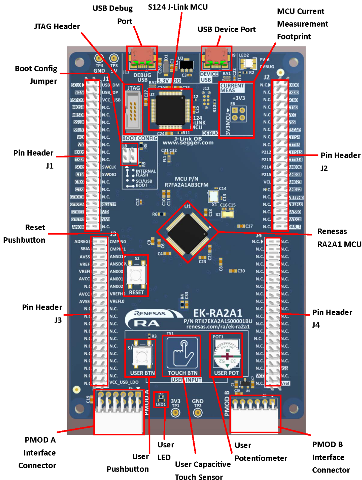
図 1 メインボード（上面）
