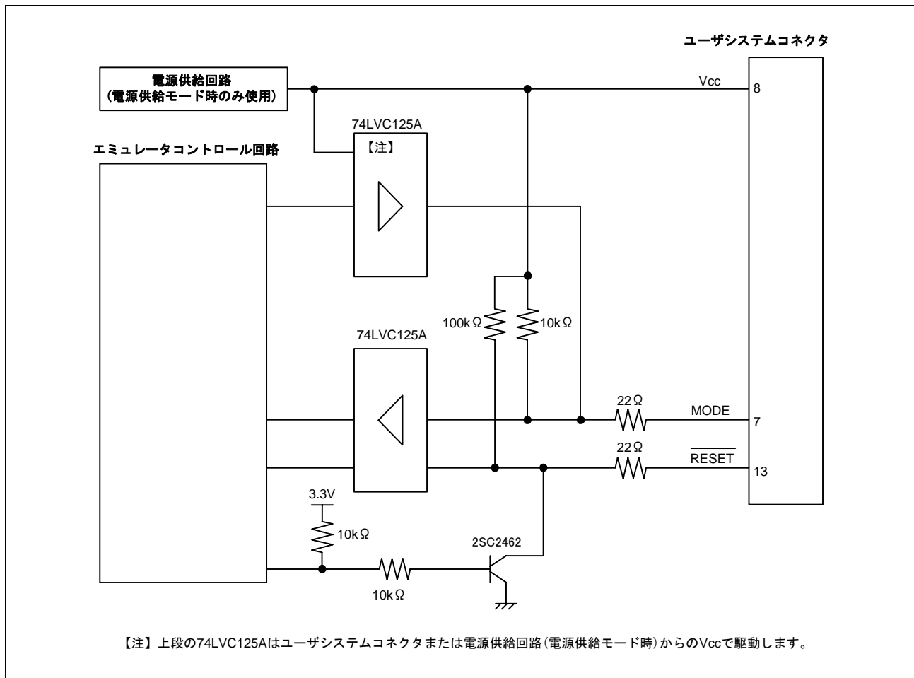
図 5.4 E8 エミュレータ内インタフェース回路 (参考)
