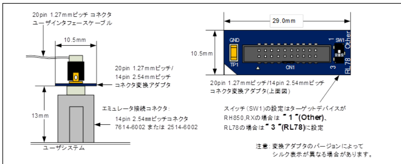
図 2-2 エミュレータ接続コネクタへの接続
