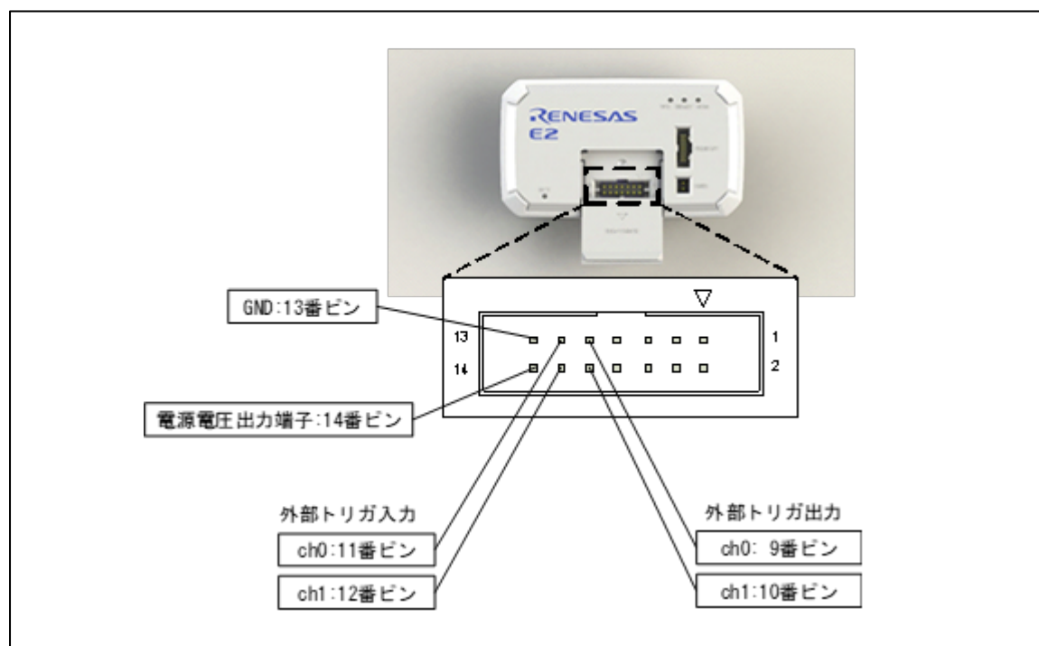
図 2-9 E2 エミュレータ拡張インタフェース
