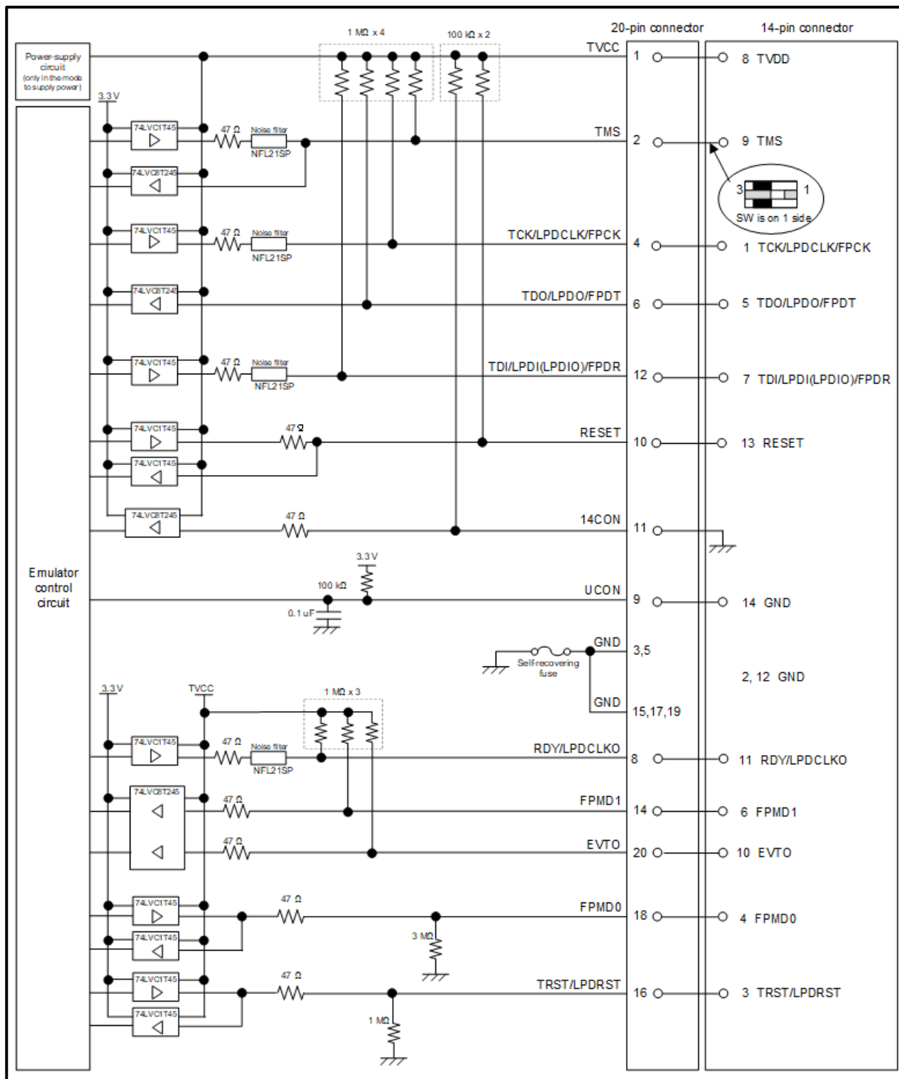
図 6-1 E2 エミュレータ(Rev.C)内インターフェース回路(LP4pin、JTAG、2wireUART、CSI)
