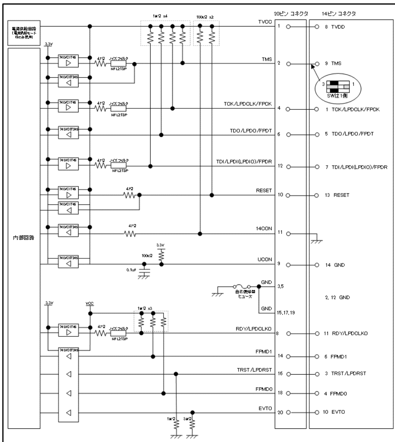
図 6-1 E2 エミュレータ (Rev. C) 内インタフェース回路 (LPD 4pin、JTAG、2wireUART、CSI)
