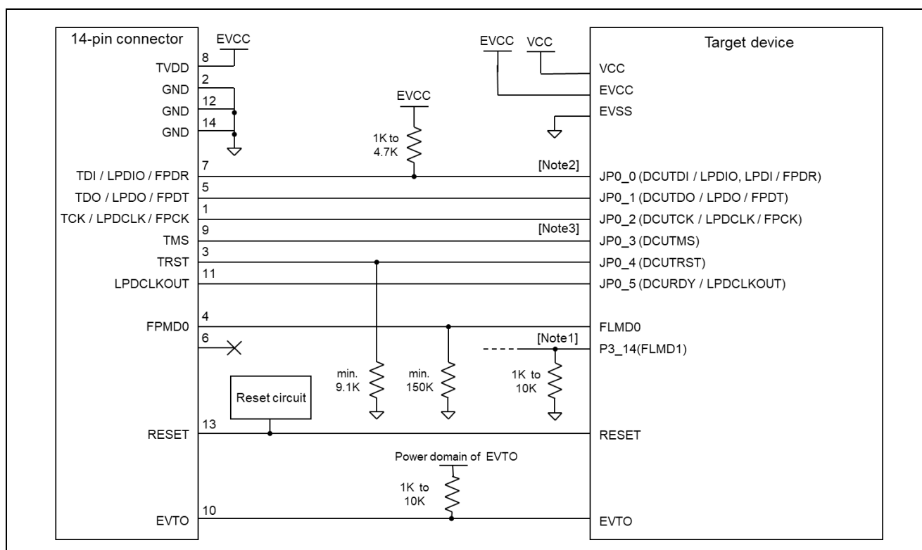
図 2-4 接続例
