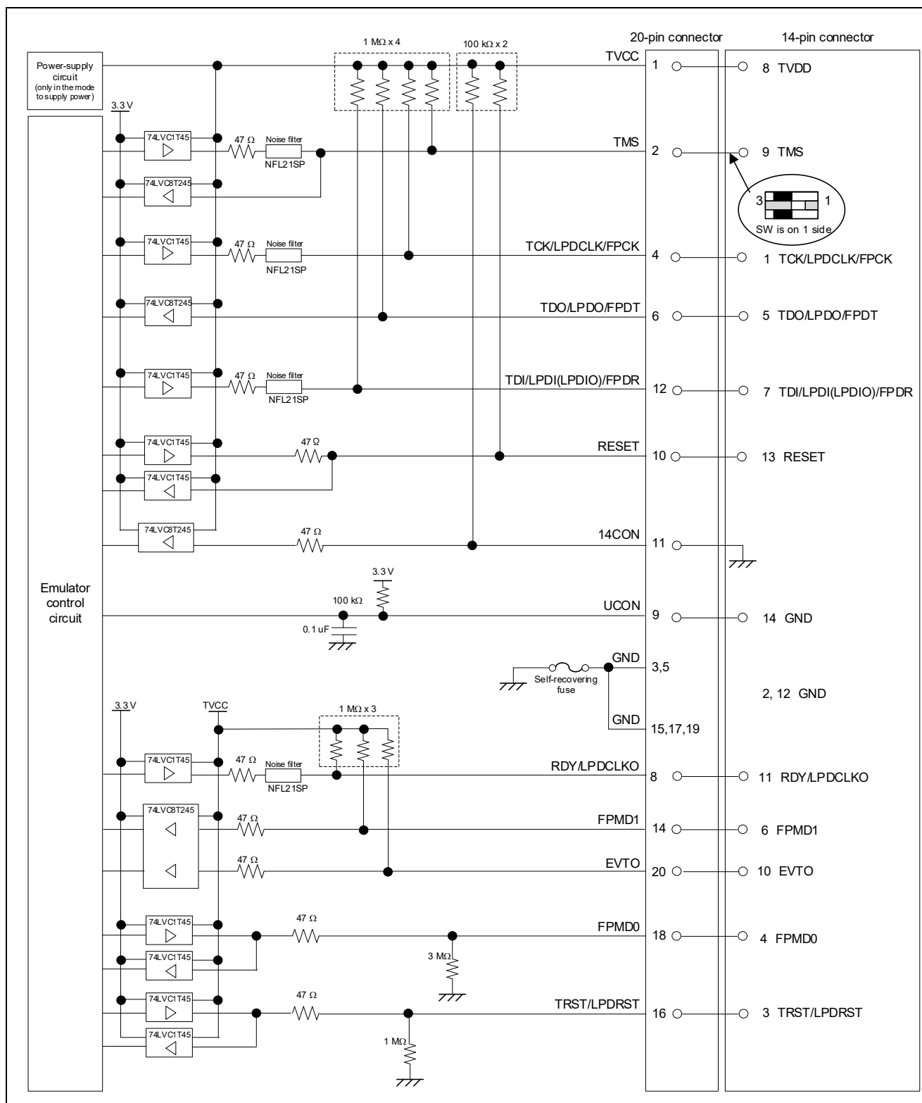
図 5-3 E2 エミュレータ (Rev.C) 内インタフェース回路 (LPD 1Pin、LPD 4pin、JTAG、1wireUART、2wireUART、CSI)
