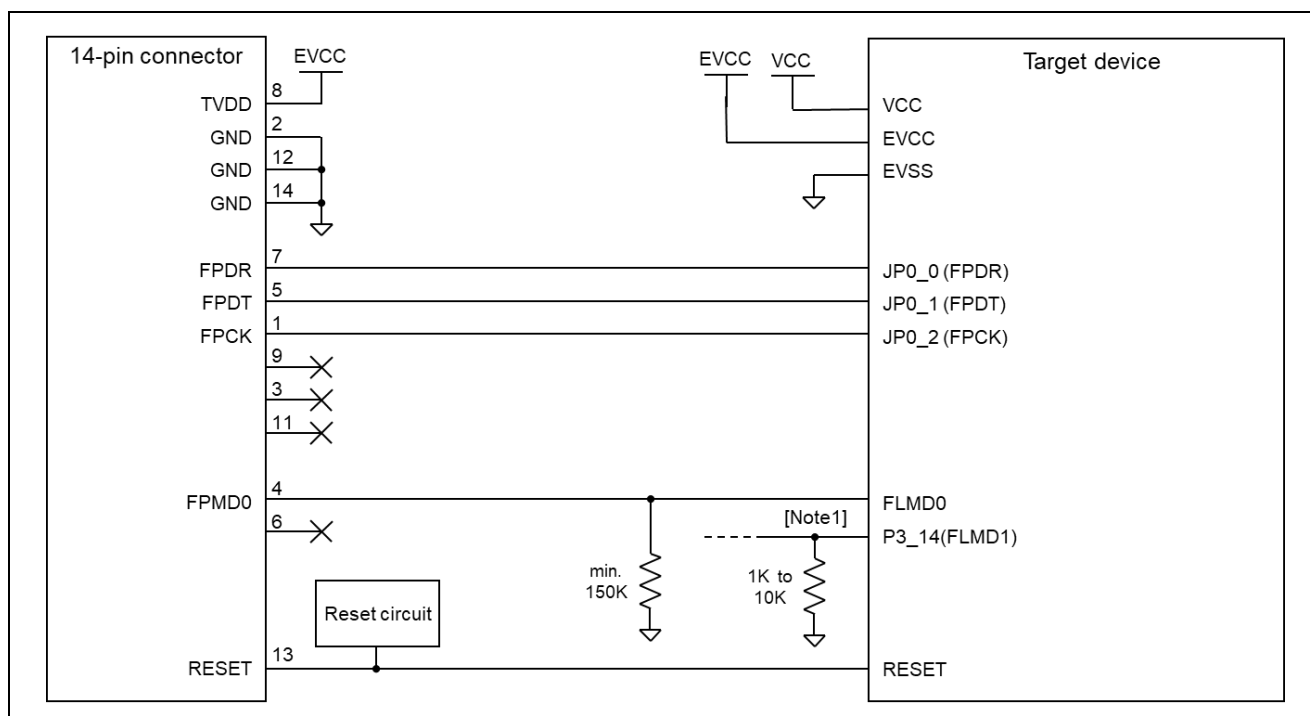
図 2-7 接続例
