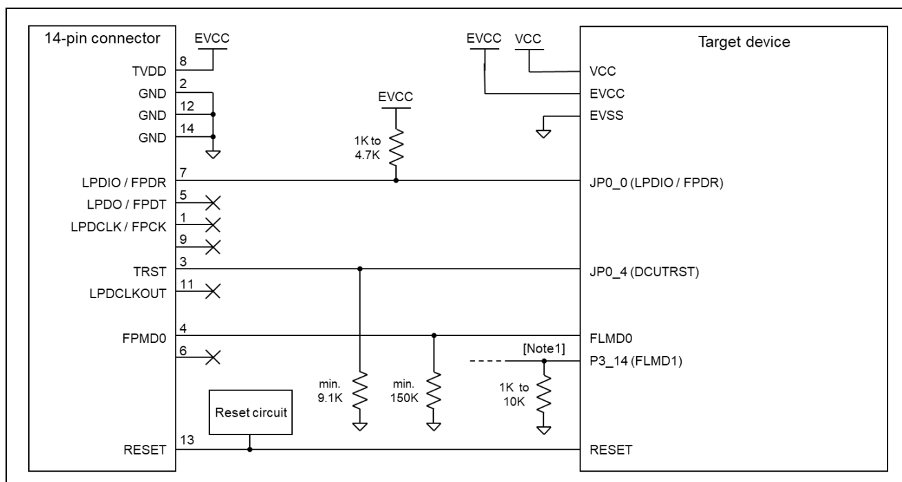
図 2-5 接続例
