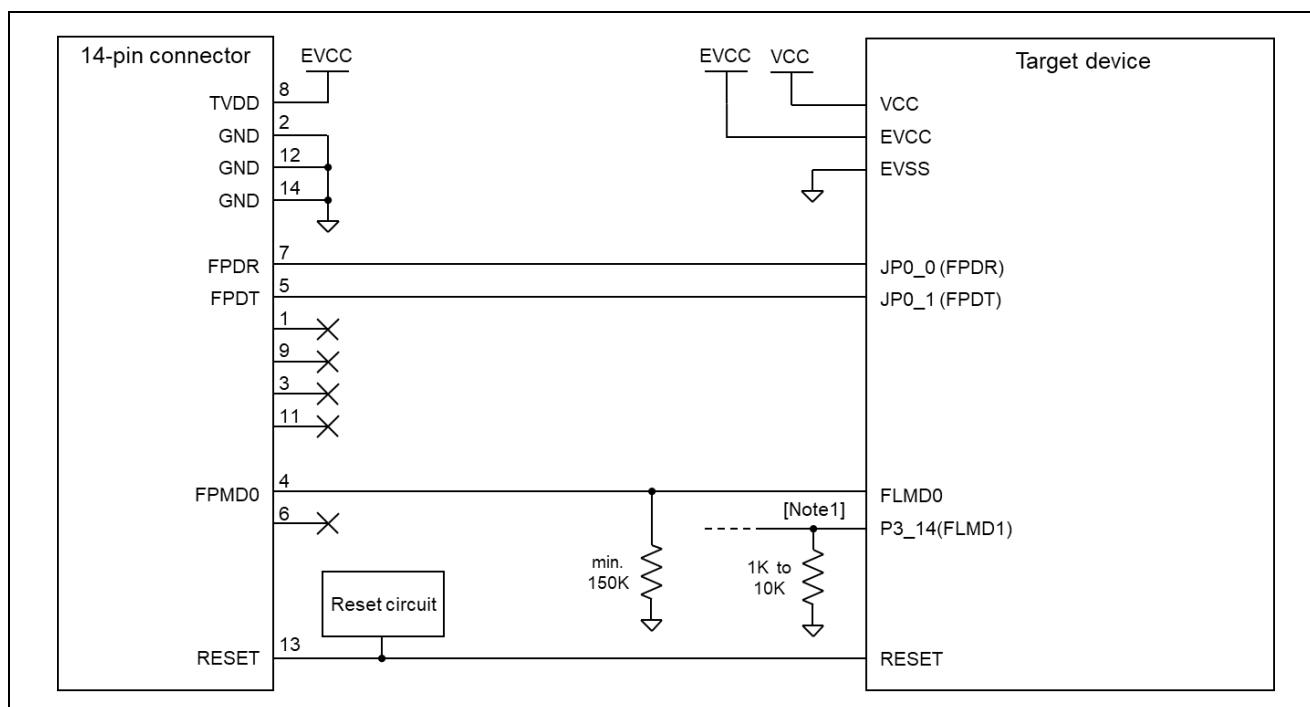
図 2-6 接続例
