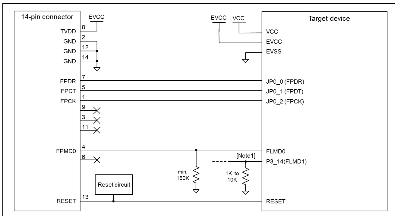
図 2-7 接続例
