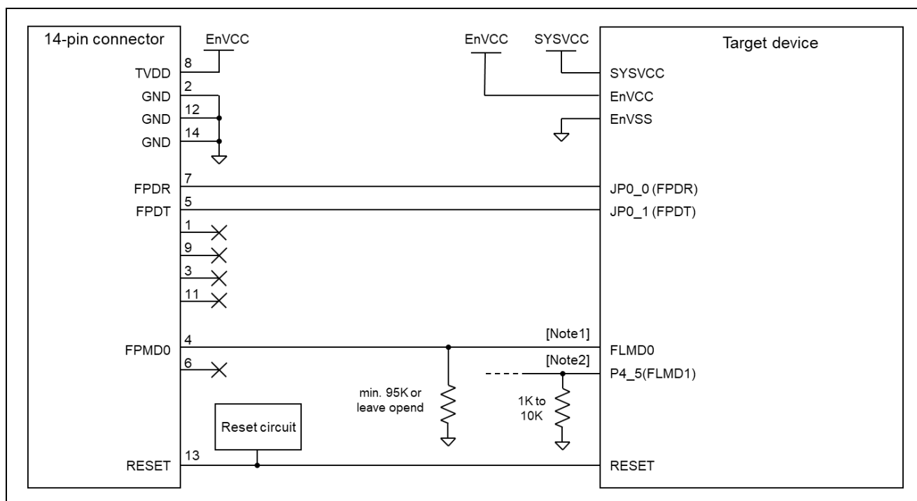
図 2-5 接続例
