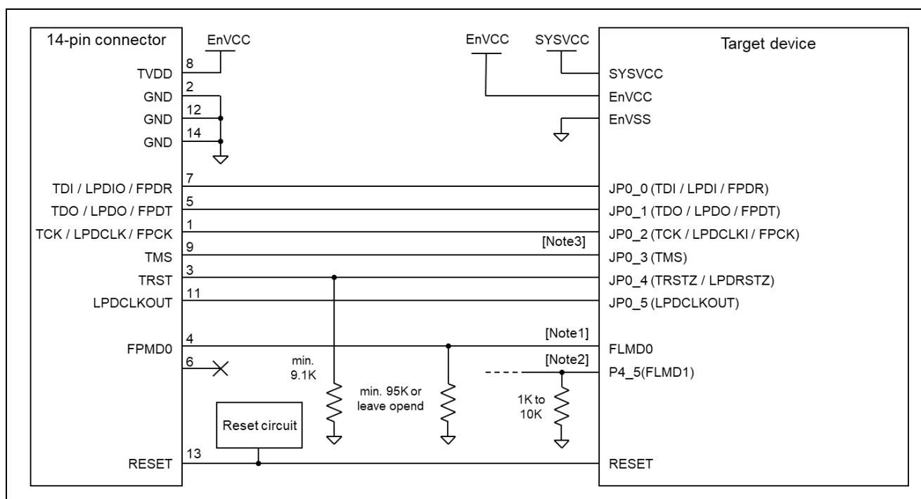
図 2-4 接続例
