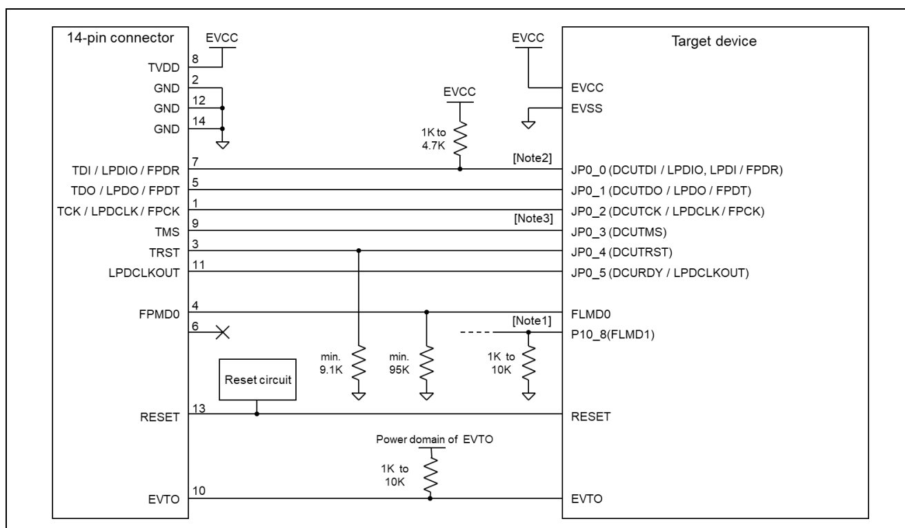
図 2-4 接続例
