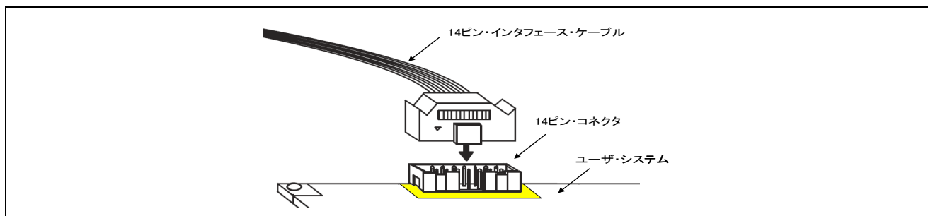
図 2-2 E1 エミュレータでの 14 ピンコネクタへのユーザインタフェースケーブル接続
