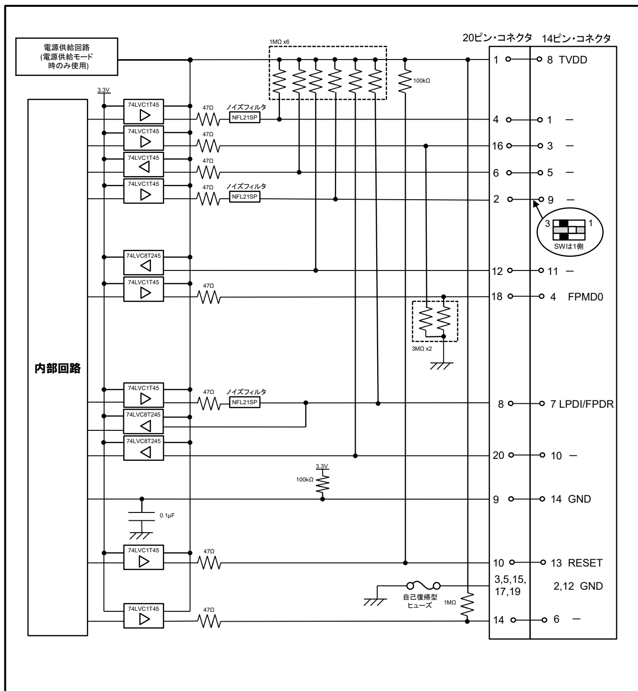
参考図 C E2 エミュレータ内インタフェース回路 (LPD1pin、1wireUART)
