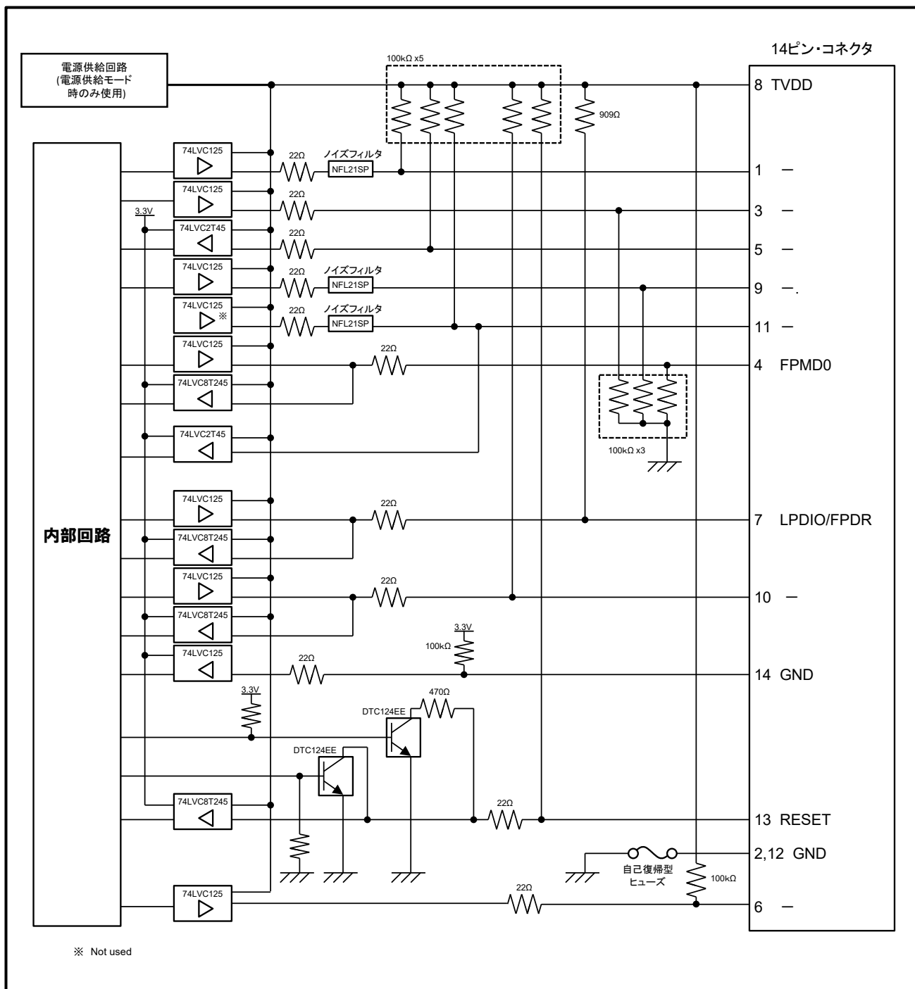
参考図 A E1/E20 エミュレータ内インタフェース回路 (LPD1pin、1wireUART)
