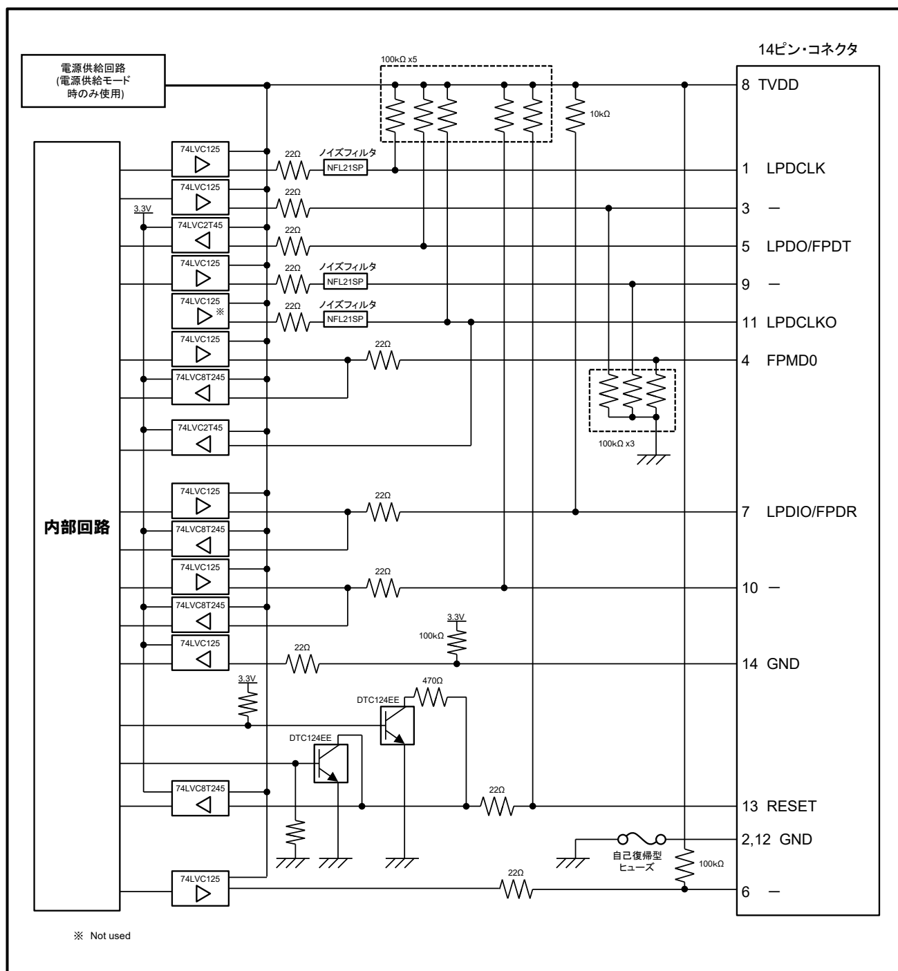
参考図 B E1/E20 エミュレータ内インタフェース回路 (LPD4pin、2wireUART)
