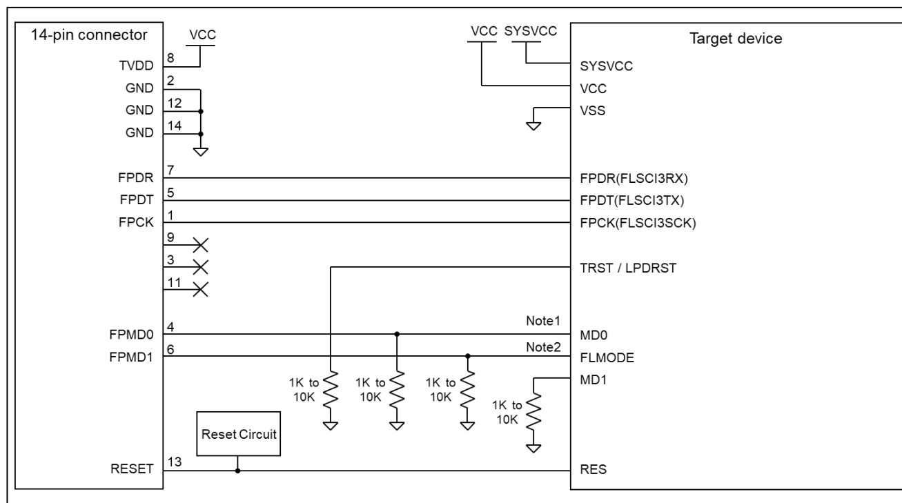
図 2-6 接続例
