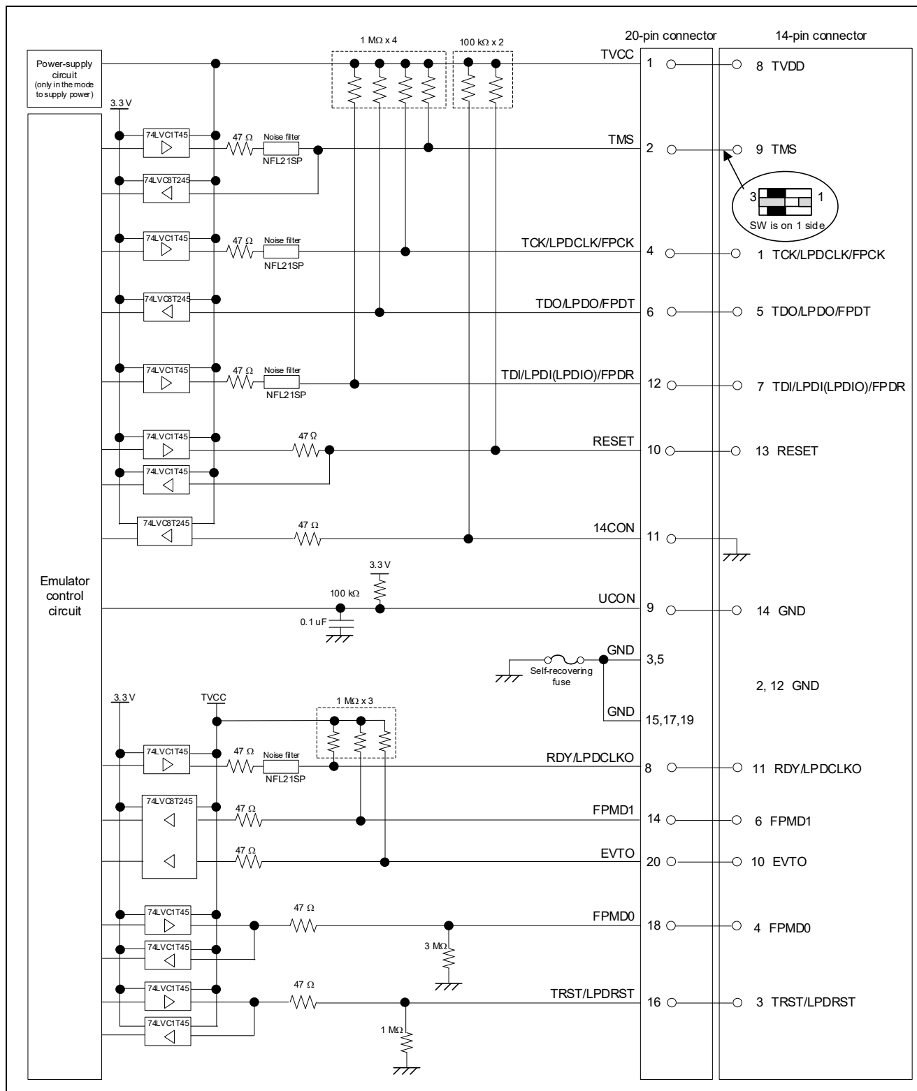
図 5-2 E2 エミュレータ(Rev.C)内インタフェース回路(LPD 4pin、JTAG、2wireUART、CSI)
