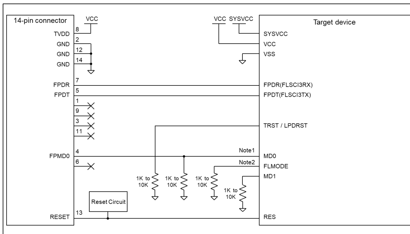
図 2-5 接続例
