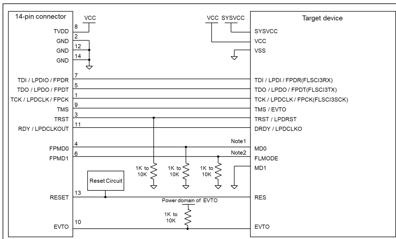
図 2-4 接続例
