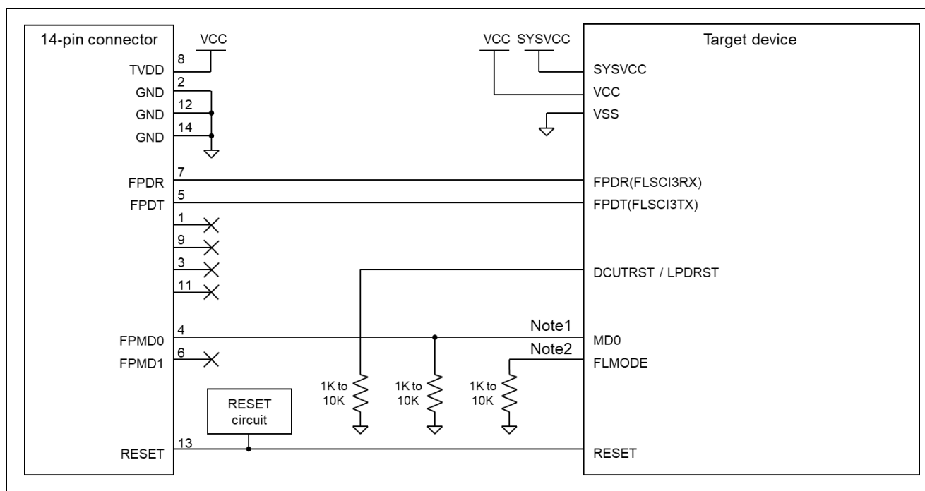
図 2-5 接続例
