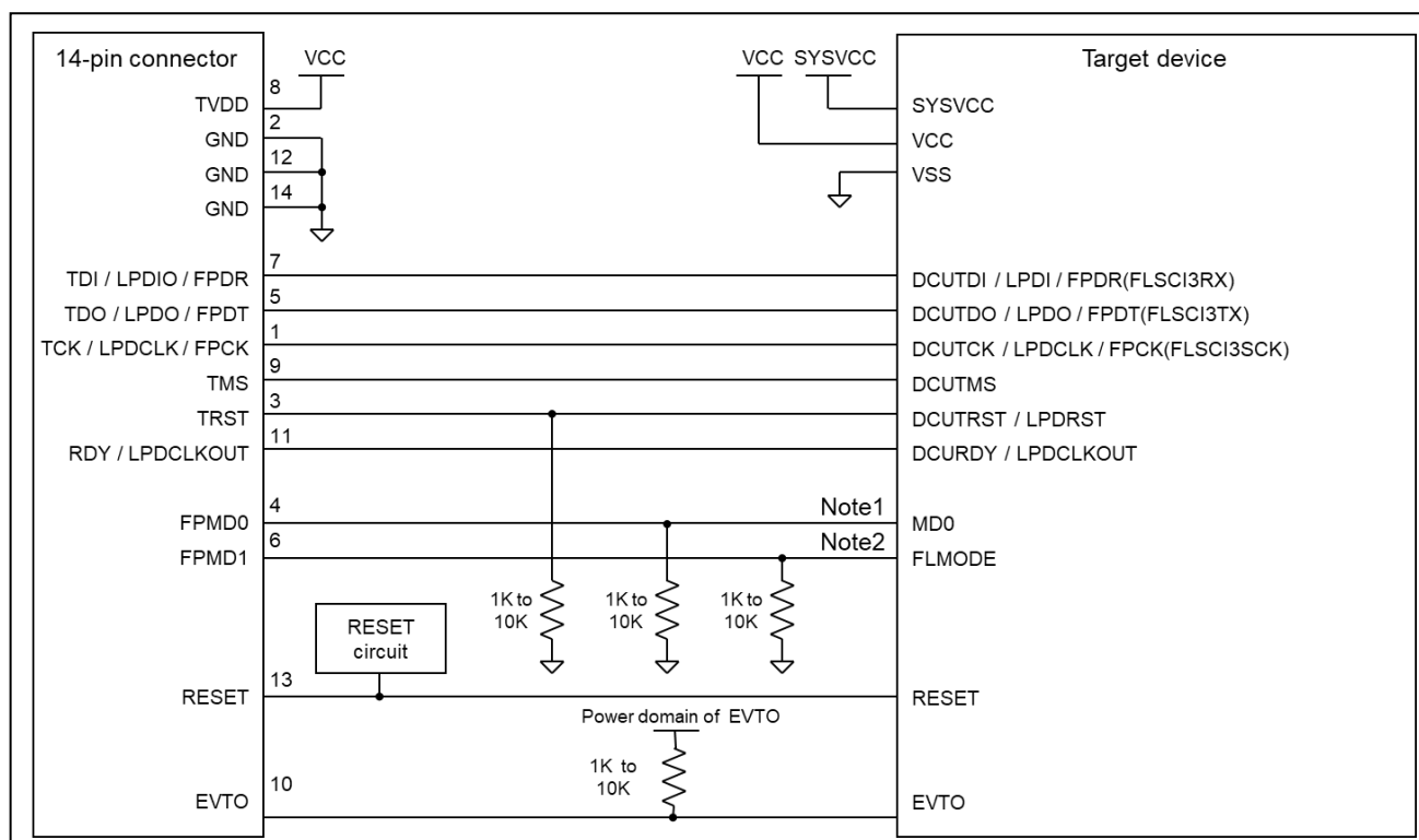
図 2-4 接続例
