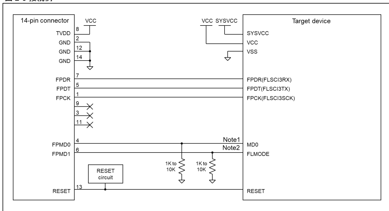
図 2-6 接続例
