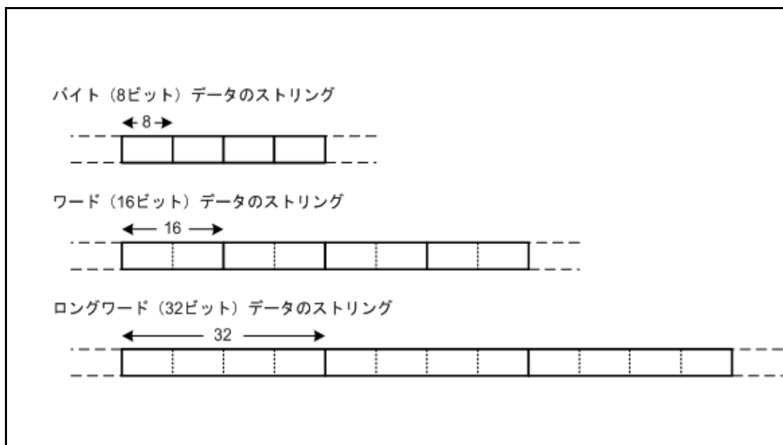
図 4—6 スtringデータ
