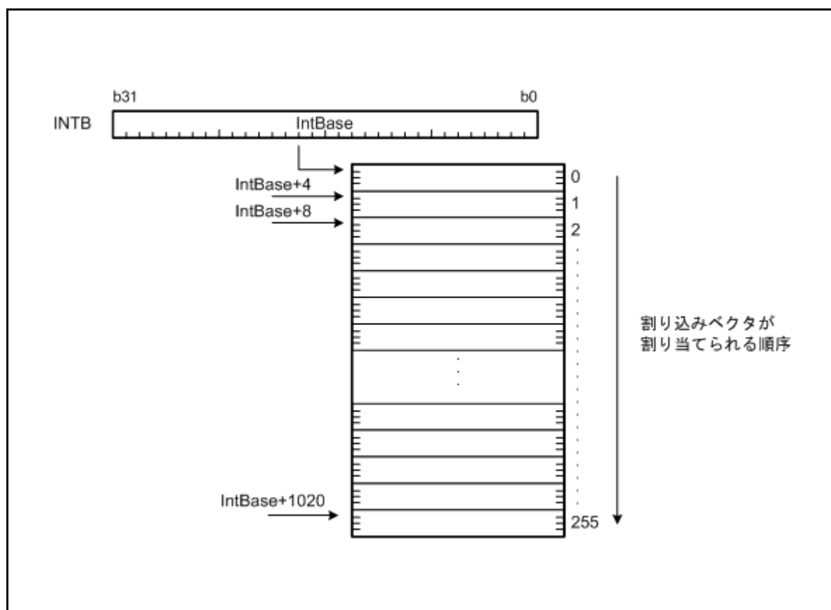
図 4—10 可変ベクタテーブル
