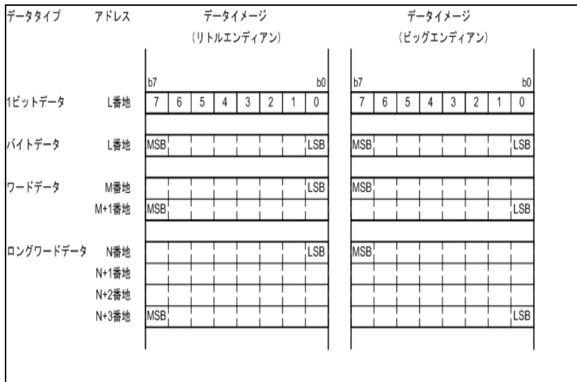
図 4—8 メモリ上のデータ配置
