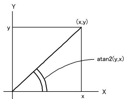
図 6—1 atan2 関数の意味
