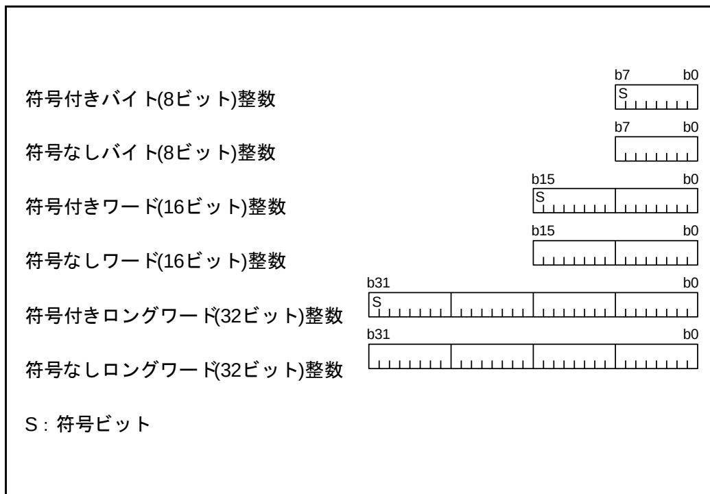
図 4—3 整数データ
