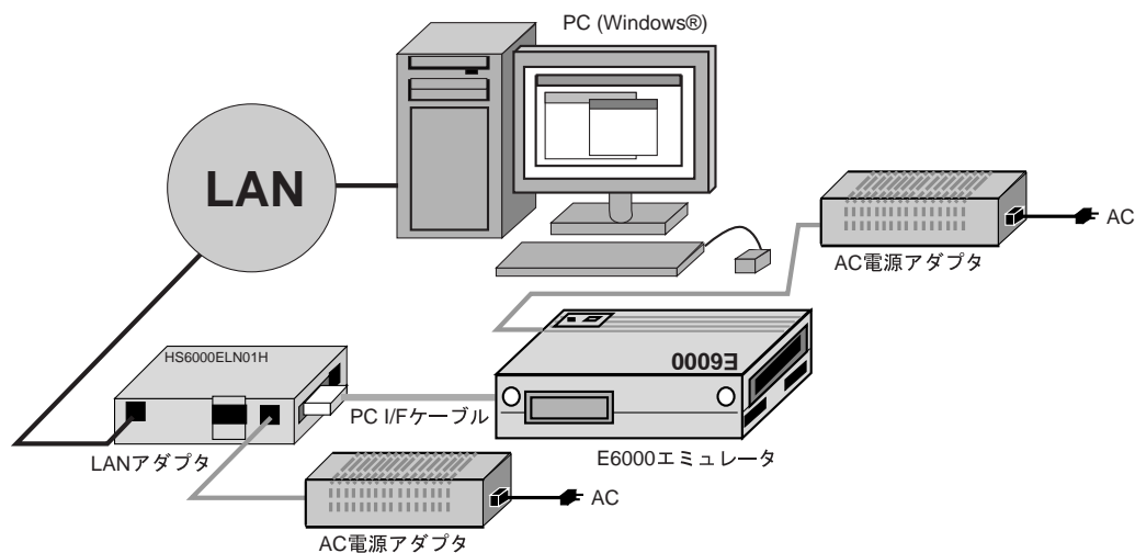
図 1.1 E6000 エミュレータ接続時のシステム構成図
