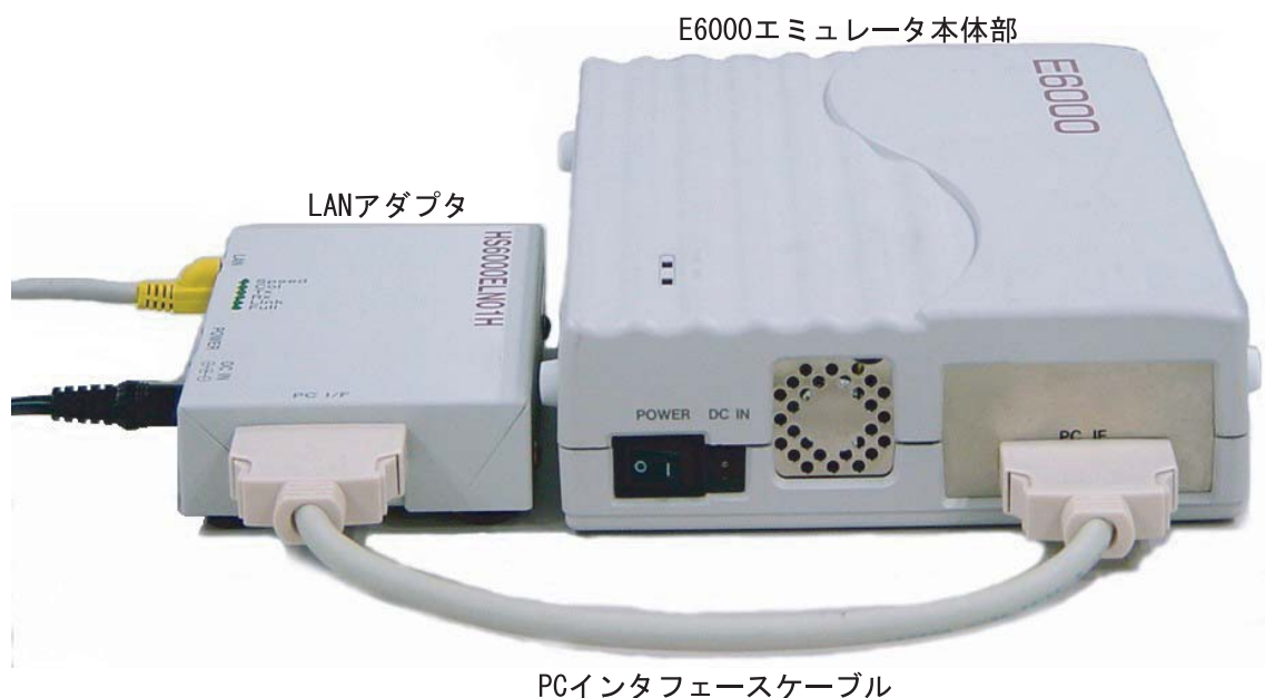
図 3.3 E6000 エミュレータと LAN アダプタとの接続
