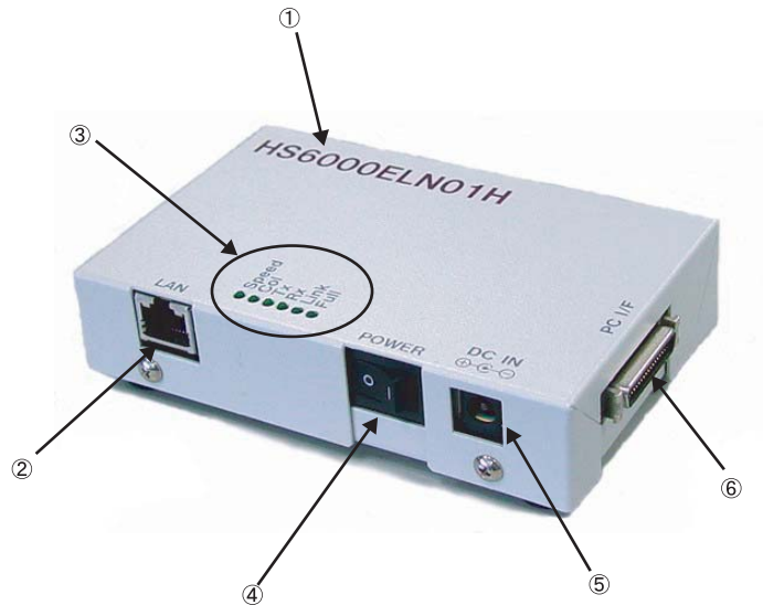
図 2.1 LAN アダプタ
