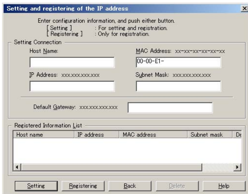
図 4.3 IP アドレスの設定と登録ダイアログ
