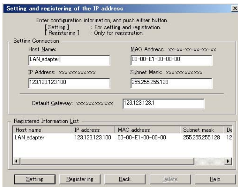
図 4.4 IP アドレスの設定と登録ダイアログ実行画面
