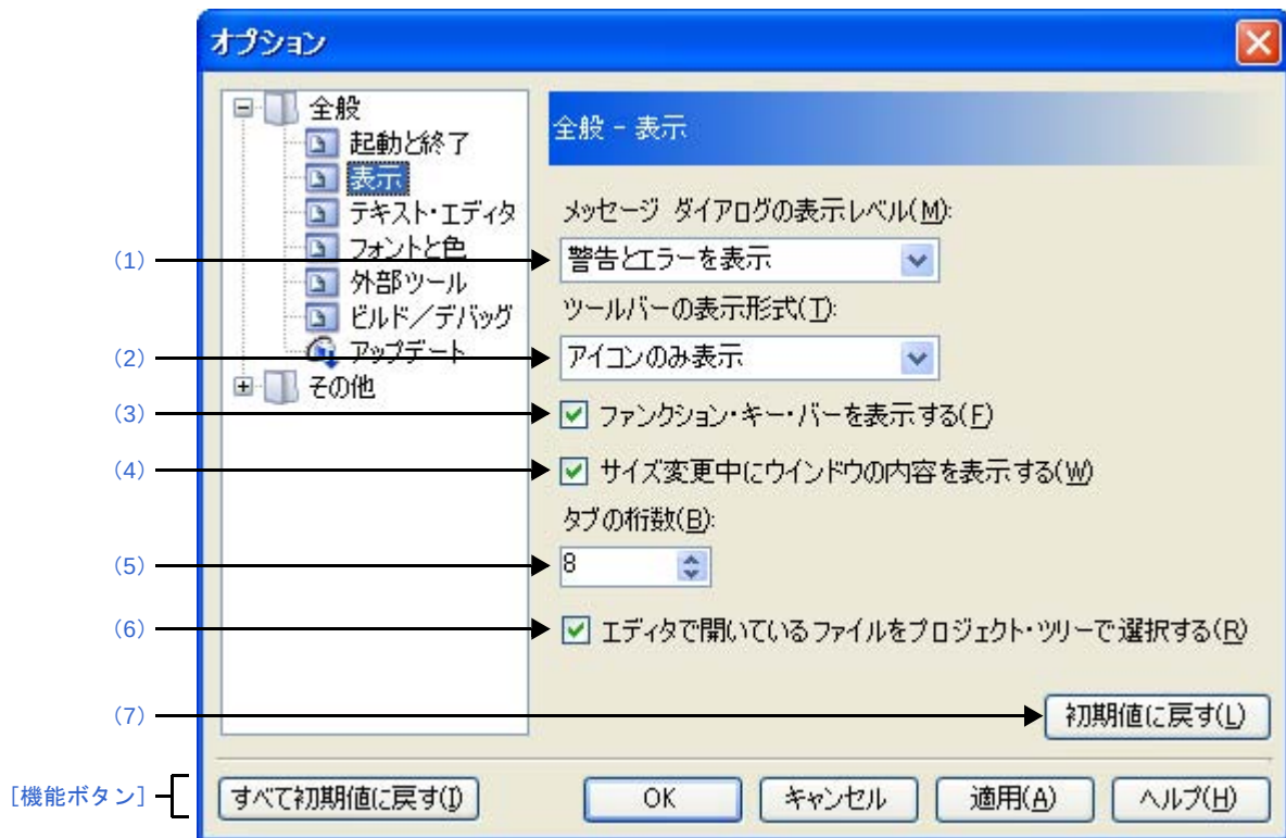
図 A—48 オプション ダイアログ ([全般 - 表示] カテゴリ)
