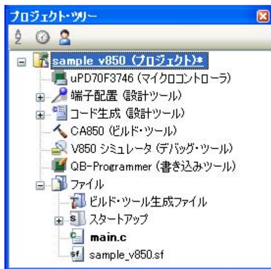
図 2—72 プロジェクト・ツリー パネル (セクション・ファイル生成後)
