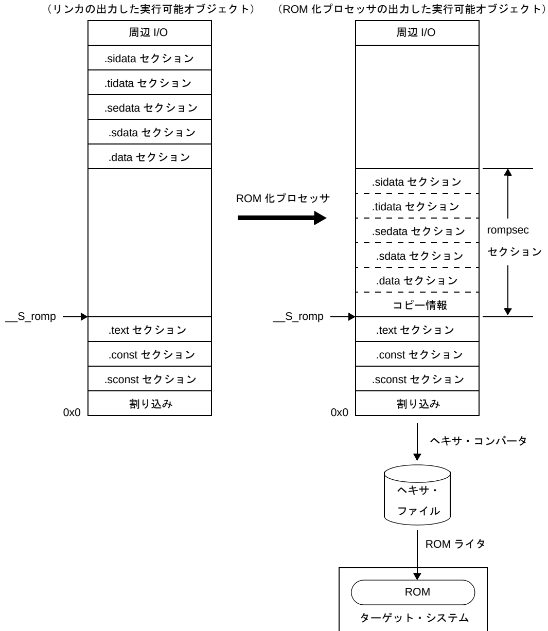
図 B—30 ROM 化のイメージ 1
