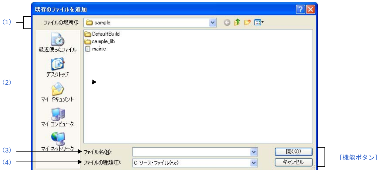
図 A—67 既存のファイルを追加 ダイアログ
