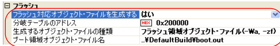
図 B—23 フラッシュ領域側の [フラッシュ] カテゴリ
