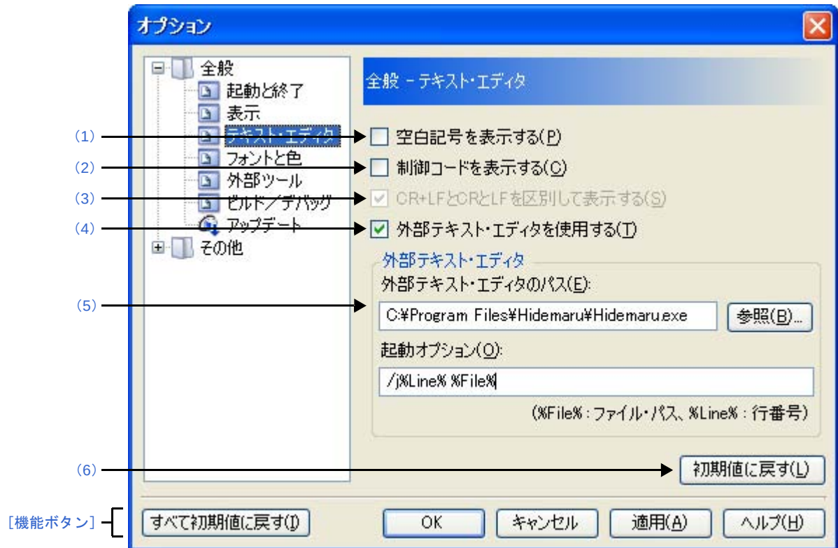
図 A—49 オプション ダイアログ ([全般 - テキスト・エディタ] カテゴリ)
