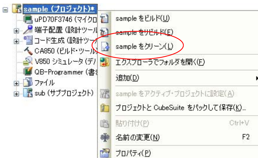
図 2—112 「アクティブ・プロジェクトをクリーン」項目
