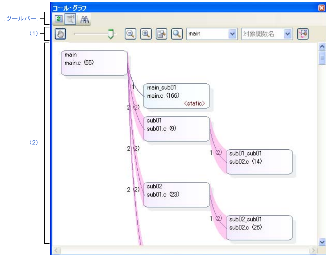
図 A—18 コール・グラフパネル (全体表示)
