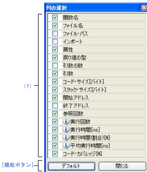
図 A—45 列の選択 ダイアログ（関数一覧パネル用）
