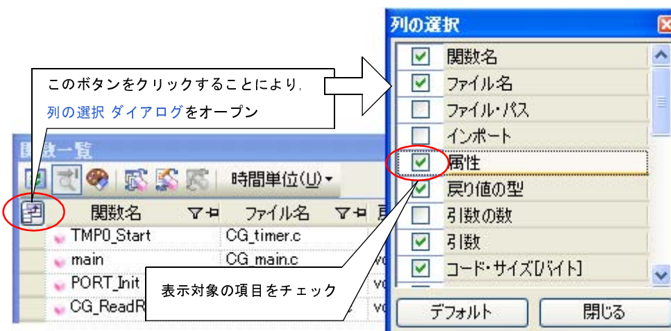
図 2—11 表示項目の追加（列の選択 ダイアログのチェック・ボックスでの操作）
