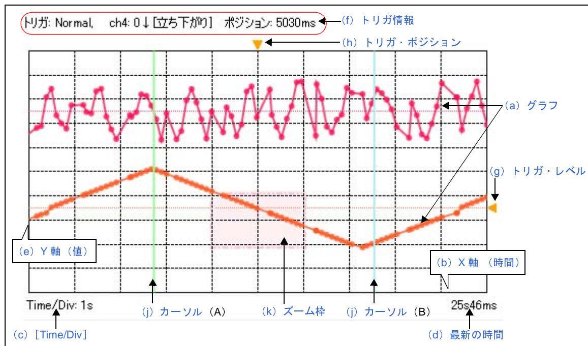
図 A—13 グラフ表示エリア
