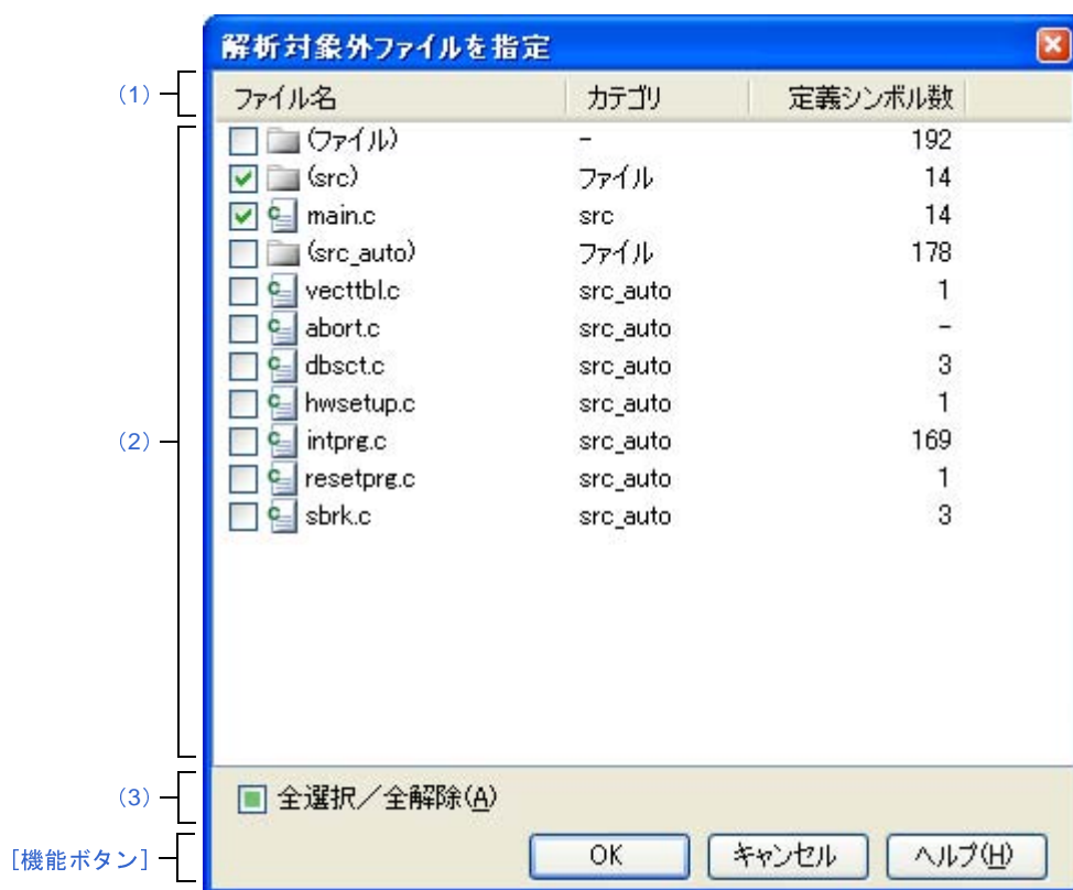
図 A—41 解析対象外ファイルを指定 ダイアログ
