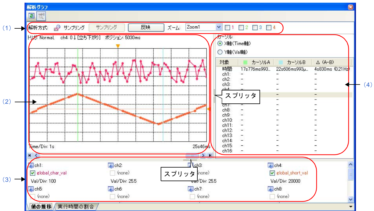
図 A—11 解析グラフパネル：[値の推移] タブ
