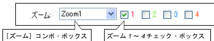
図 2—34 ズーム表示
