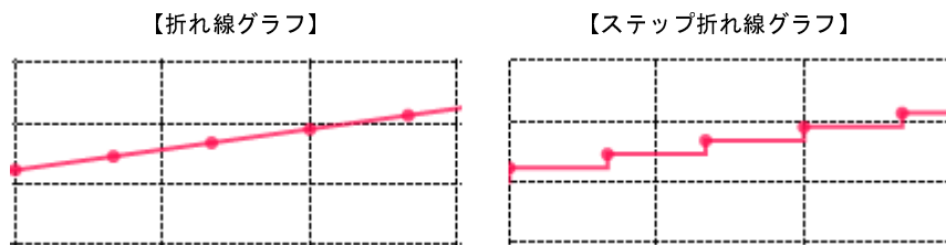
図 2—32 グラフ形式
