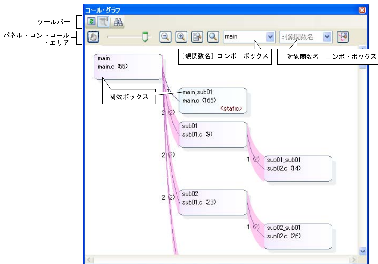
図 2—3 関数間の呼び出し関係の表示（コール・グラフパネル：全体表示）
