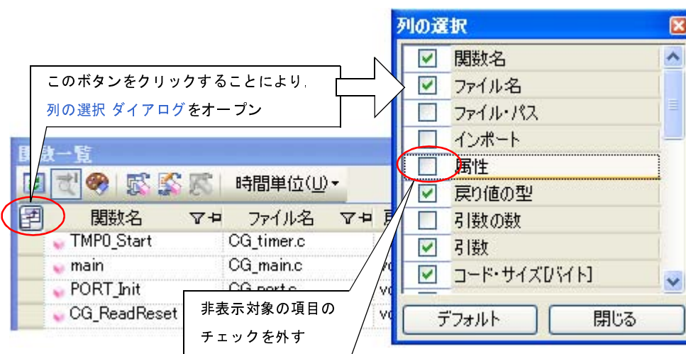
図 2—10 表示項目の限定（列の選択 ダイアログによる操作）
