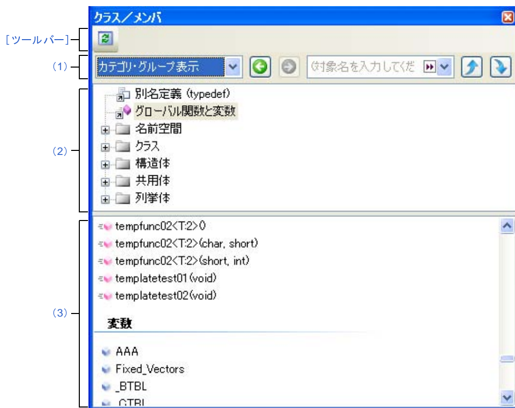
図 A—24 クラス／メンバパネル
