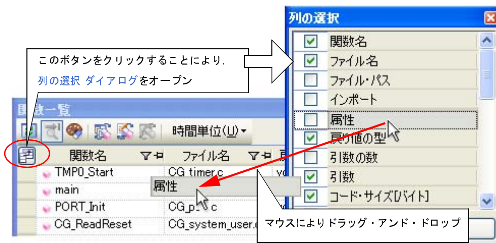
図 2—12 表示項目の追加 (列の選択 ダイアログからのドラッグ・アンド・ドロップ操作)
