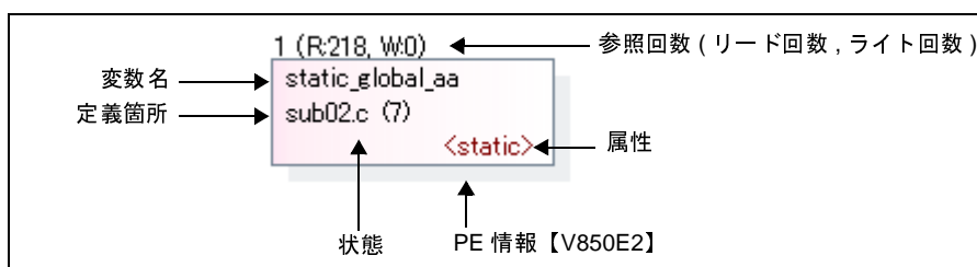
図 A—22 変数ボックスの情報
