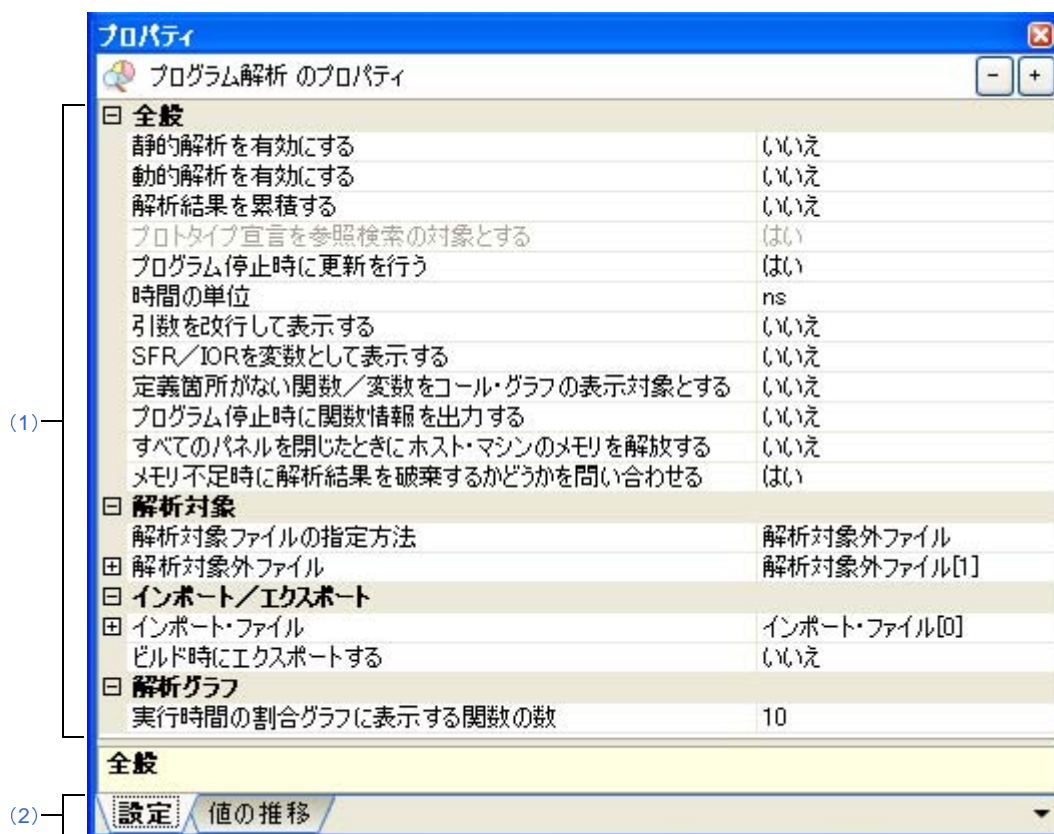
図 A—3 プロパティ パネル ([V850] の例)
