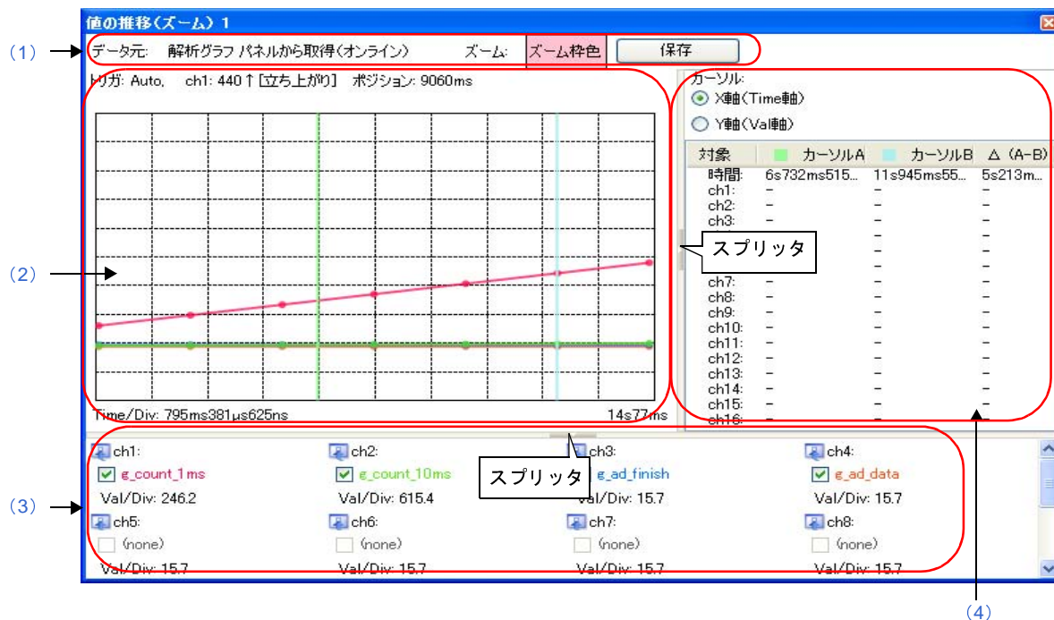
図 A—26 値の推移 (ズーム) パネル
