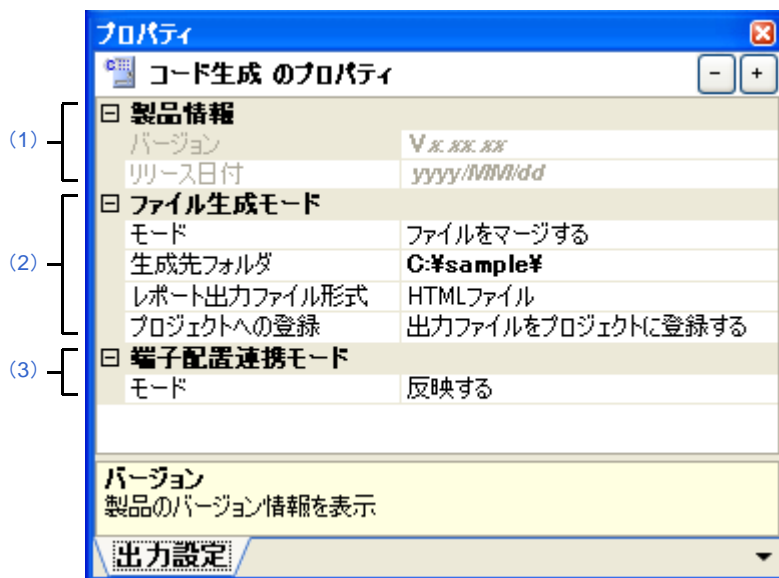
図 A-8 [出力設定] タブ
