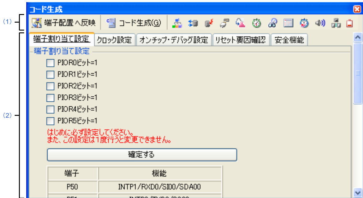
図 A—16 コード生成 パネル：[クロック発生回路]
