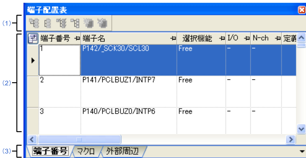
図 A—11 端子配置表 パネル
