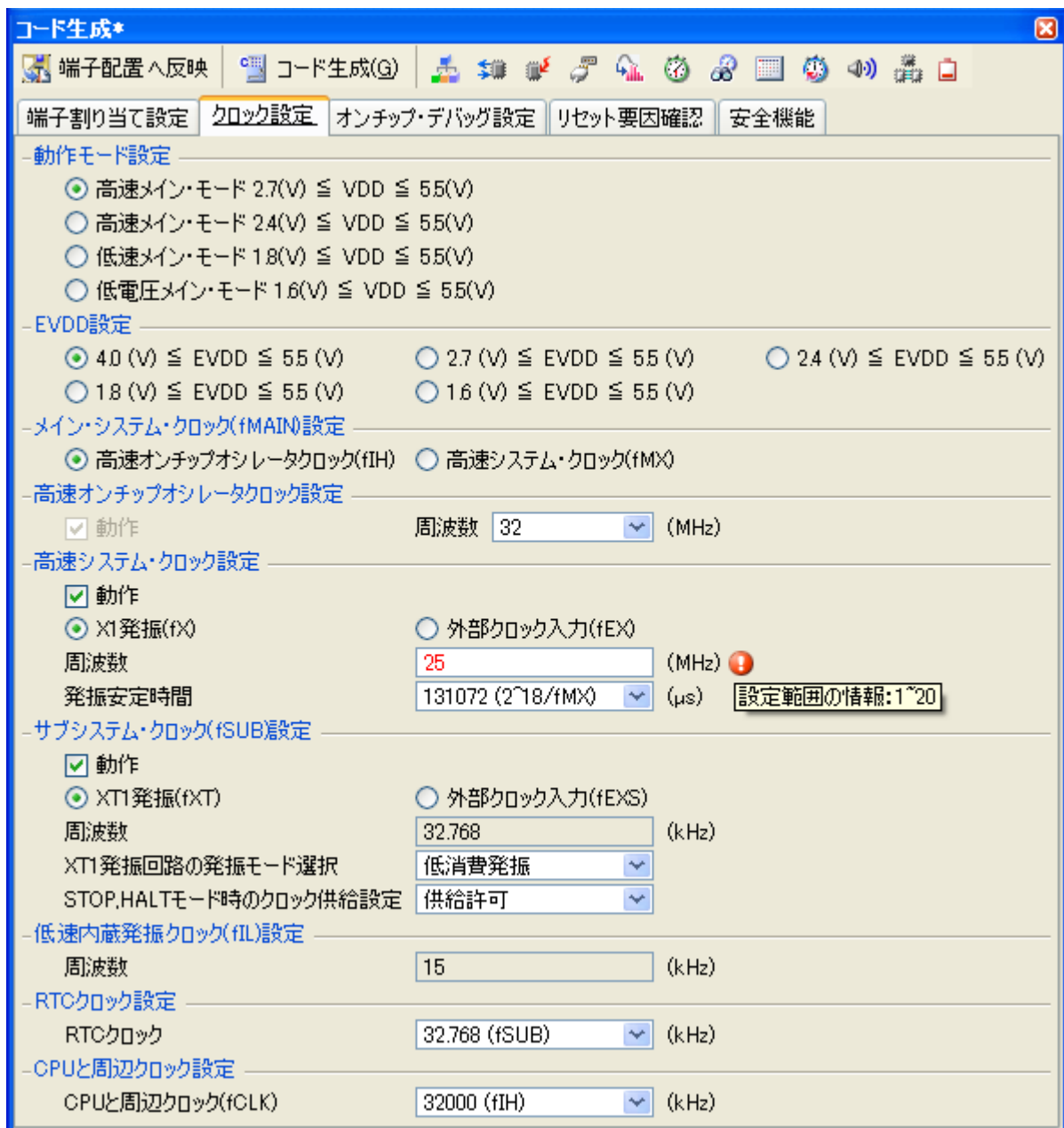
図 3—2 入力不備箇所に対するアイコン表示
