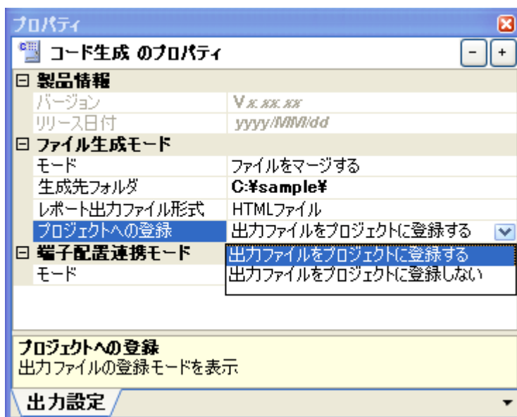
図 3—6 登録有無の設定
