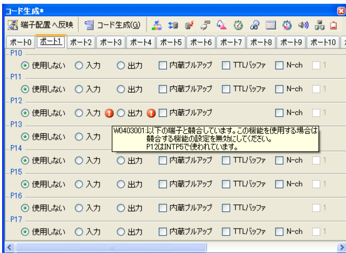
図 3—3 端子の競合に対するアイコン表示
