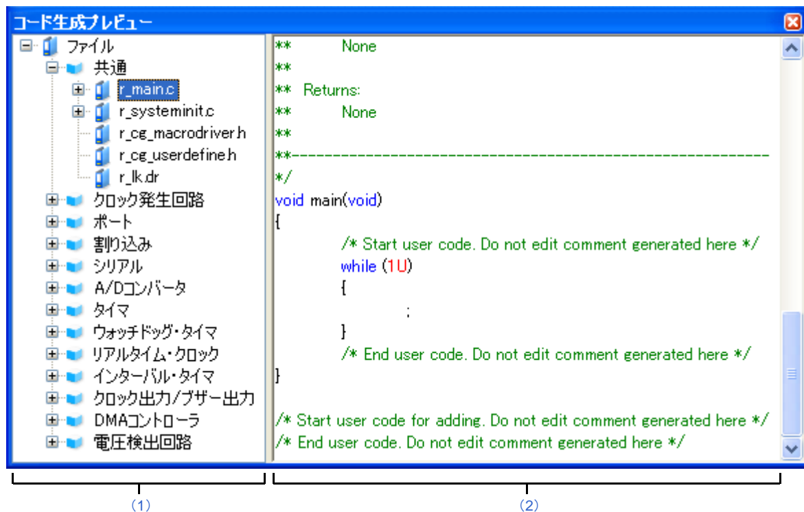
図 A—17 コード生成プレビュー パネル
