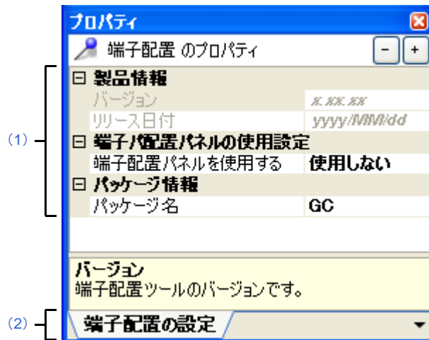
図 A—3 プロパティ パネル ([端子配置 (設計ツール)] 選択)
