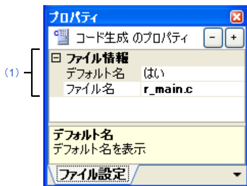
図 A—10 [ファイル設定] タブ
