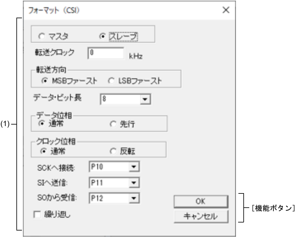
図 A.98 フォーマット（CSI）ダイアログ
