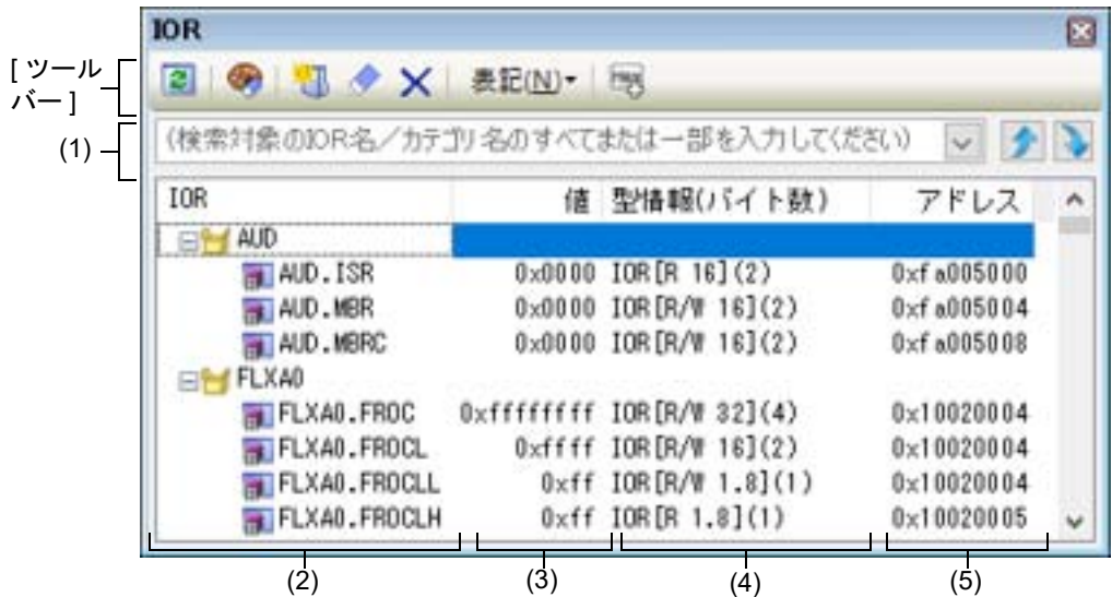
図 A.12 IOR パネル
