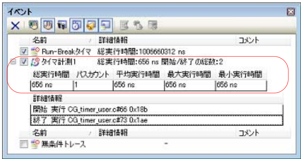
図 2.83 タイマ計測イベント（タイマ開始イベント／タイマ終了イベント）の測定結果例【シミュレータ】
