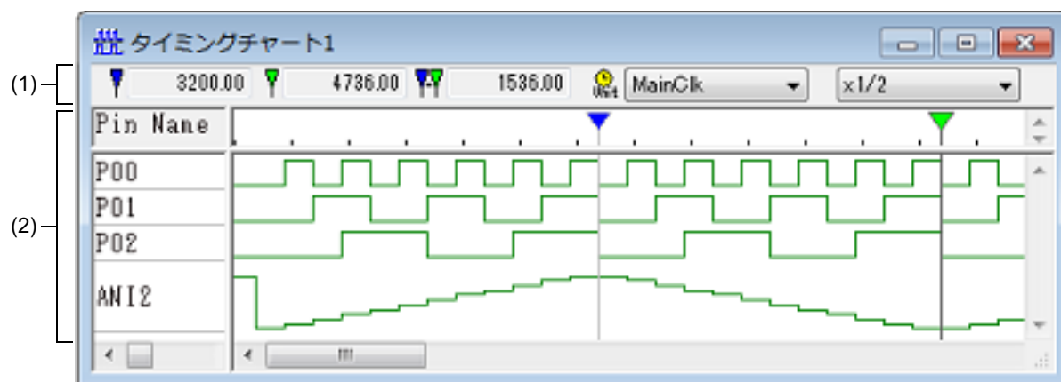
図 A.63 タイミングチャート ウィンドウ
