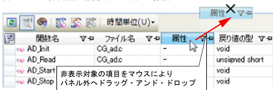
図 2.9 表示項目の限定（パネル内での操作）
