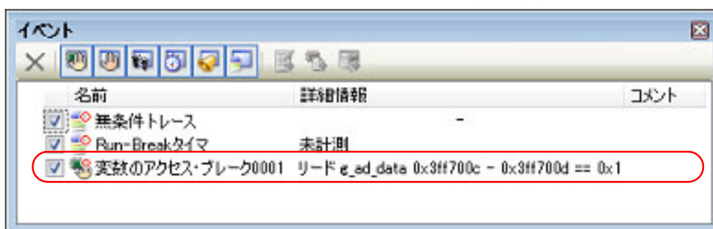
図 2.18 イベント パネルのブレーク・イベント（アクセス系）の設定例
