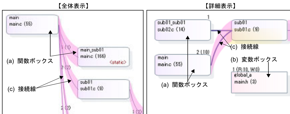
図 A.18 コール・グラフの構成要素
