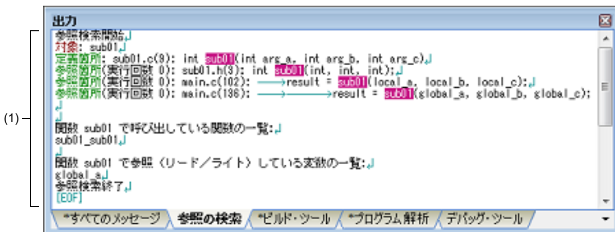
図 A.32 出力 パネル：「参照の検索」タブ
