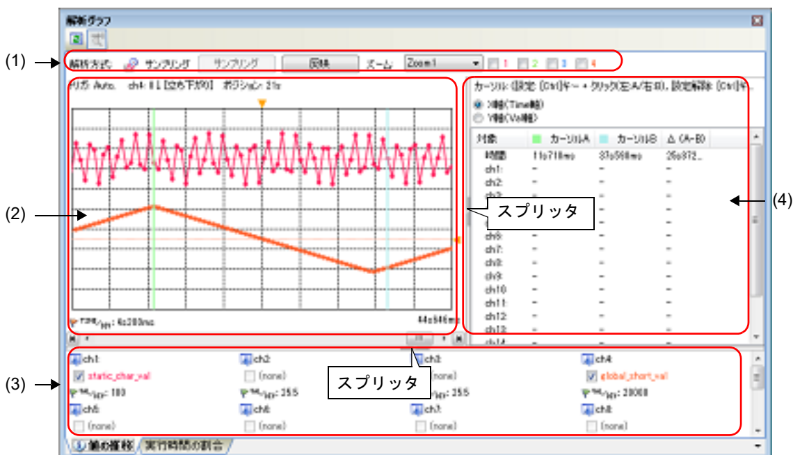
図 A.9 解析グラフ パネル：〔値の推移〕 タブ
