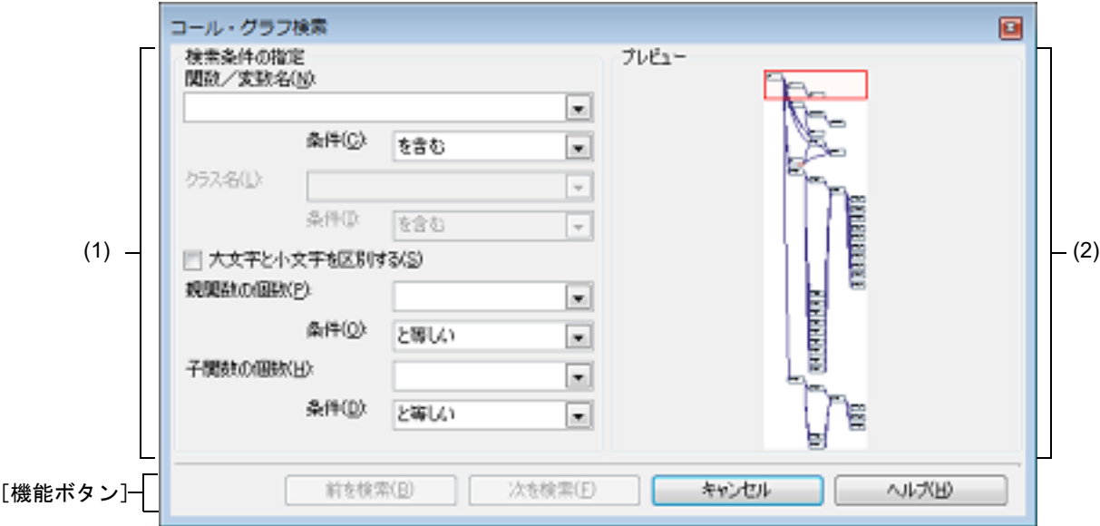
図 A.43 コール・グラフ検索 ダイアログ
