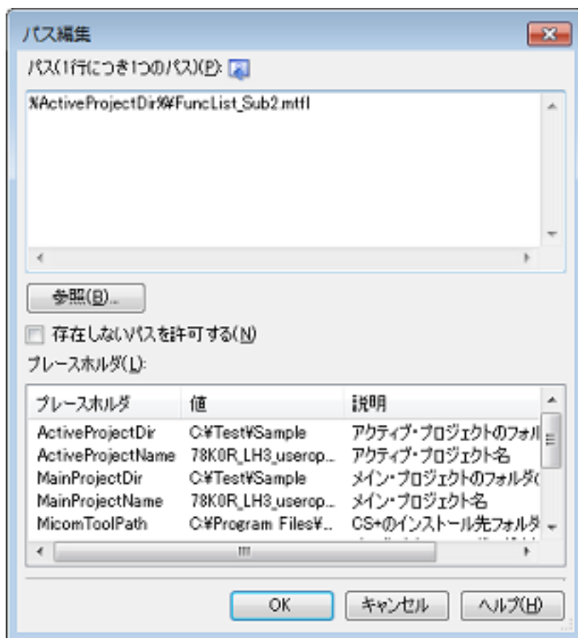
図 2.23 インポート・ファイル名の設定（パス編集 ダイアログ）
