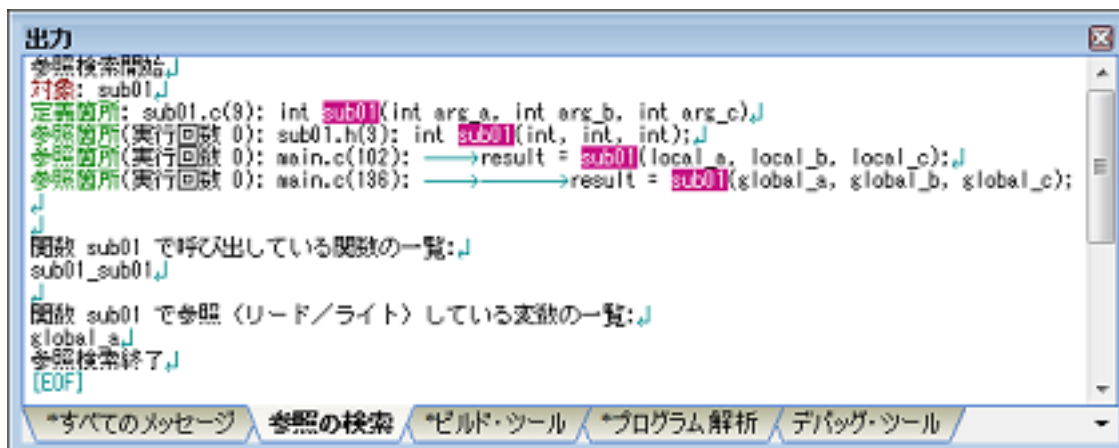
図 2.19 関数／変数の参照箇所一覧の出力例（出力パネル）
