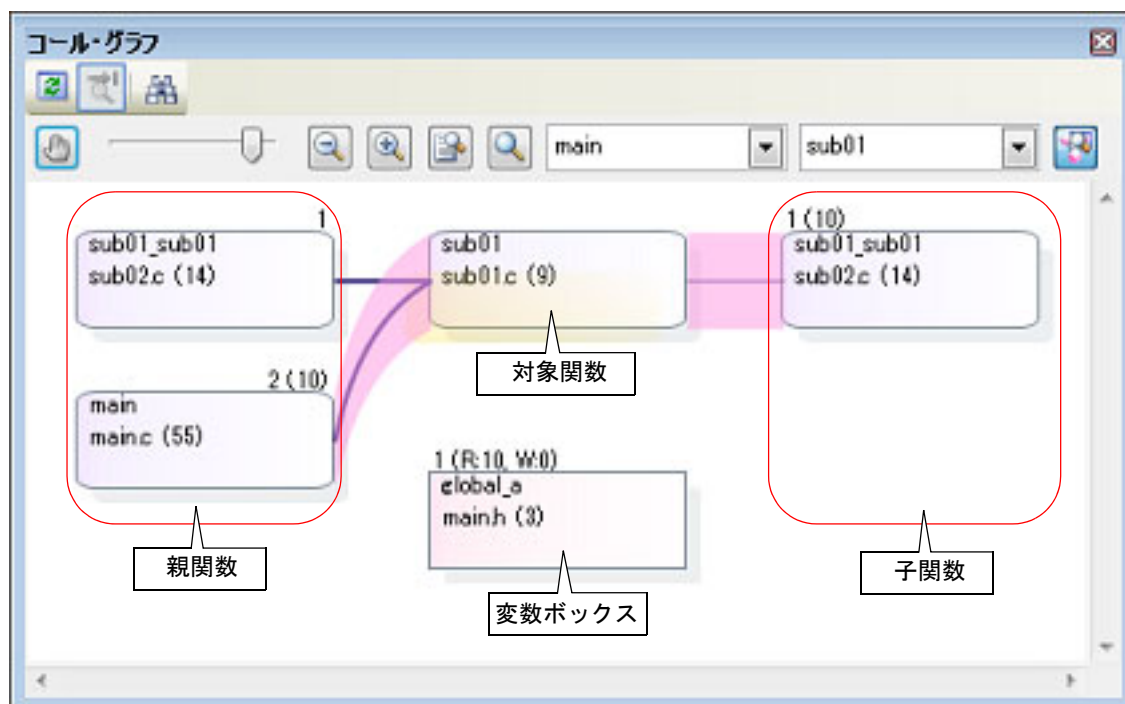
図 A.17 コール・グラフ パネル（詳細表示）
