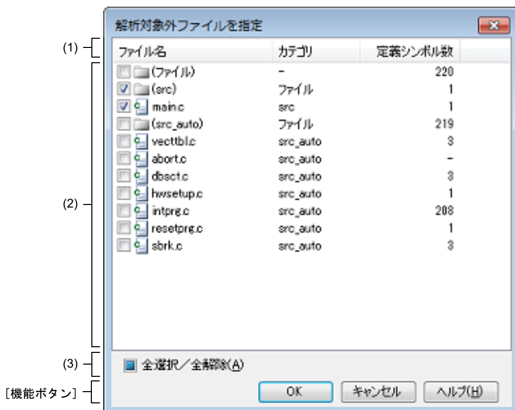
図 A.39 解析対象外ファイルを指定 ダイアログ
