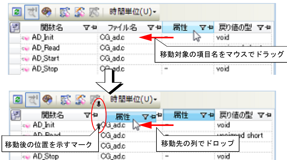
図 2.13 表示項目の並び替え（パネル内での操作）
