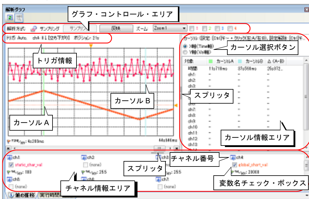
図 2.26 変数値の推移のグラフ化
