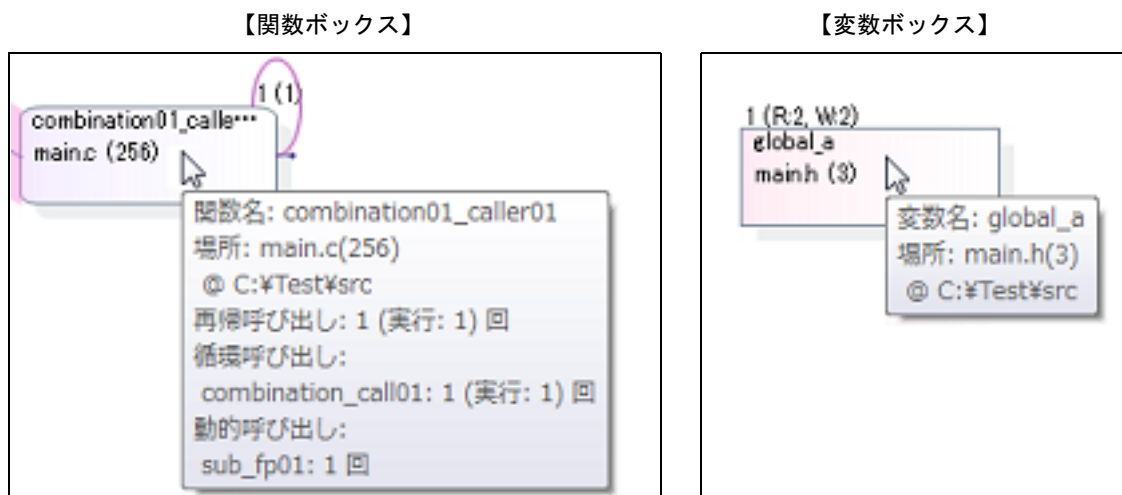
図 2.5 関数情報／変数情報のポップアップ表示例
