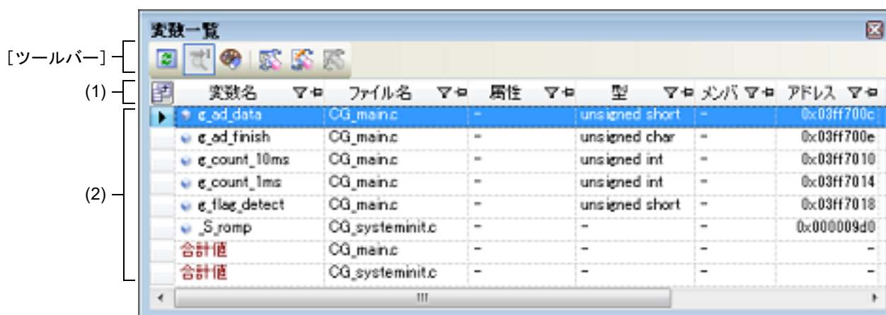
図 A.6 変数一覧 パネル
