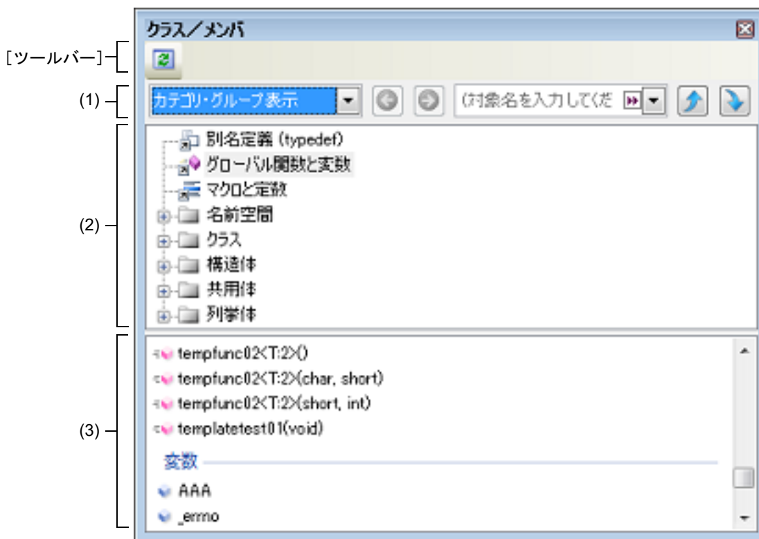
図 A.22 クラス／メンバパネル
