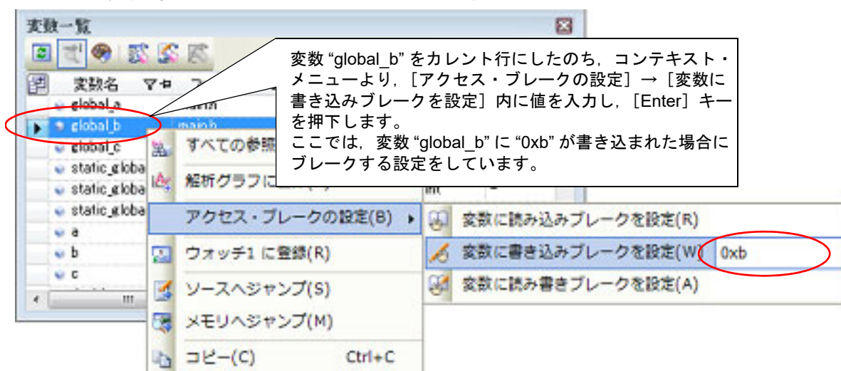
図 2.17 変数一覧 パネルにおけるブレーク・イベントの設定例
