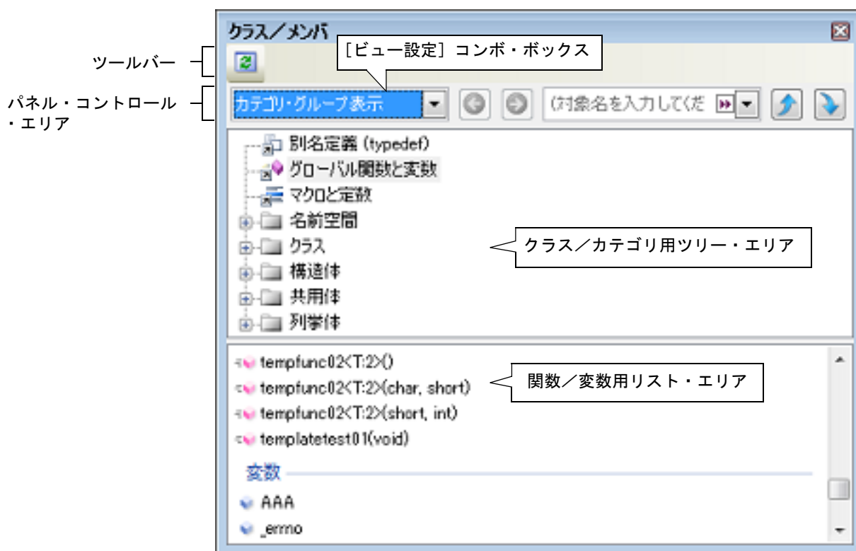
図 2.8 クラス情報の表示（クラス／メンバパネル）
