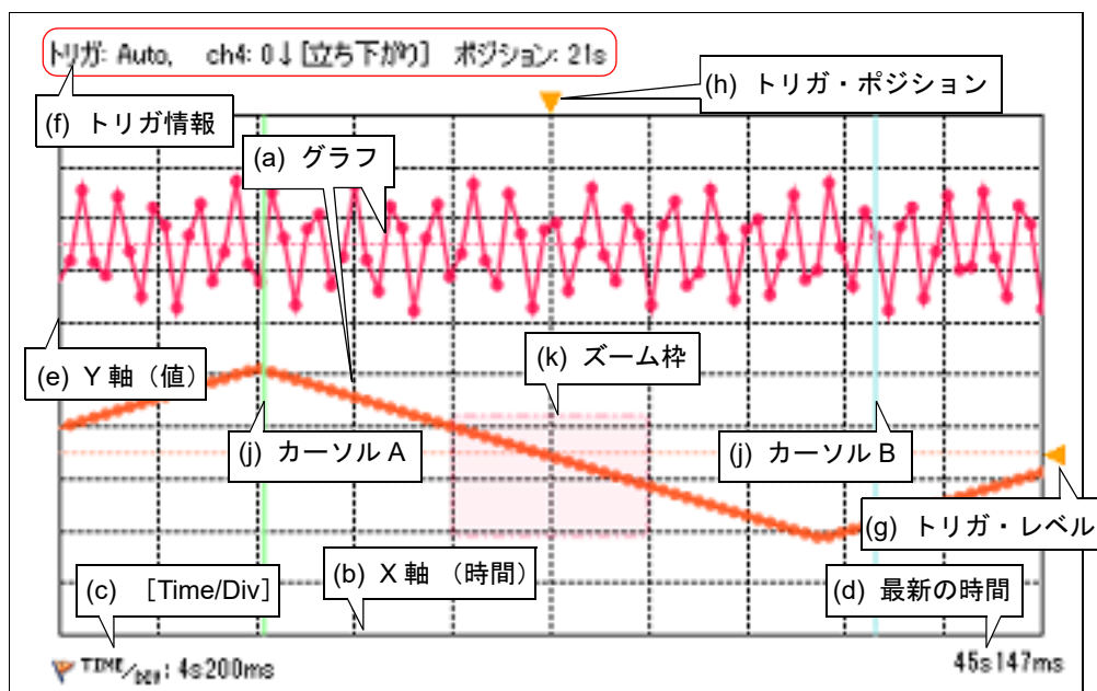
図 A.11 グラフ表示エリア
