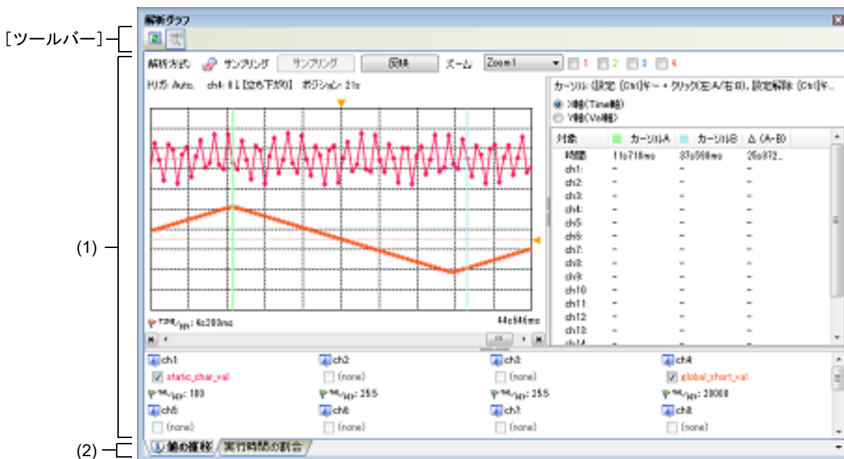
図 A.8 解析グラフ パネル
