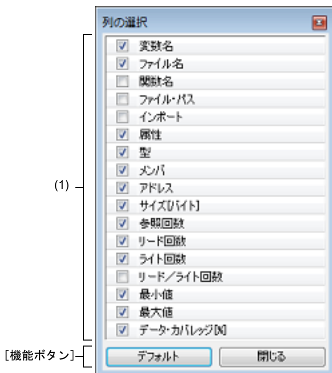
図 A.42 列の選択 ダイアログ（変数一覧 パネル用）
