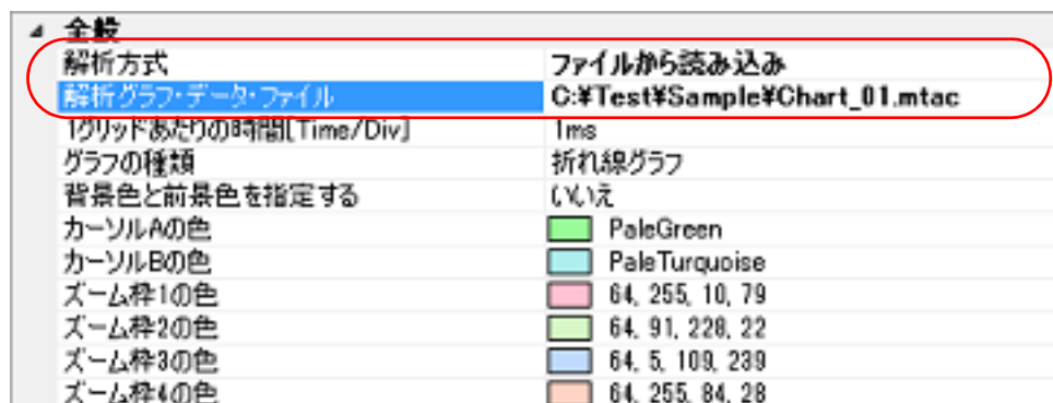
図 2.36 グラフ・データの読み込み（〔全般〕カテゴリ）
