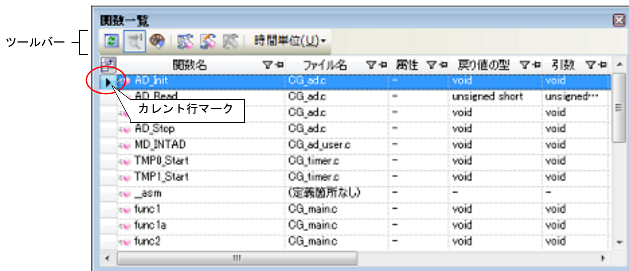
図 2.1 関数情報の表示（関数一覧パネル）
