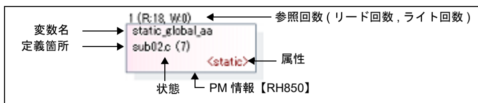
図 A.20 変数ボックスの情報
