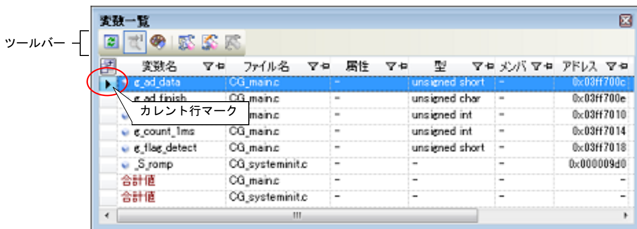
図 2.2 変数情報の表示（変数一覧パネル）
