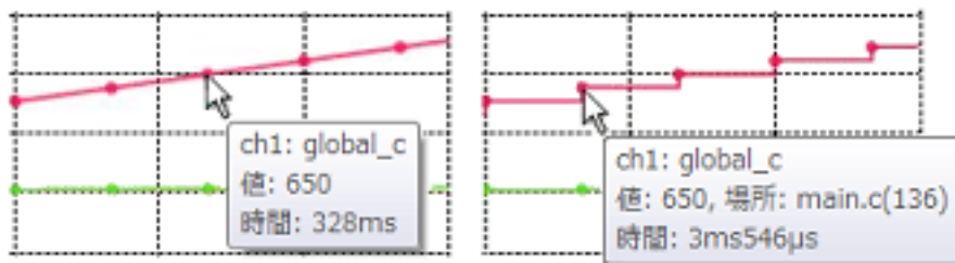
図 2.33 遷移箇所のポップアップ表示例
