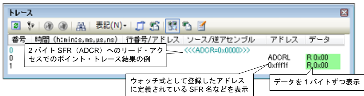
図 2.125 ポイント・トレース・イベントの結果表示例（16 ビット（2 バイト）変数/SFR の場合）【IECUBE】
