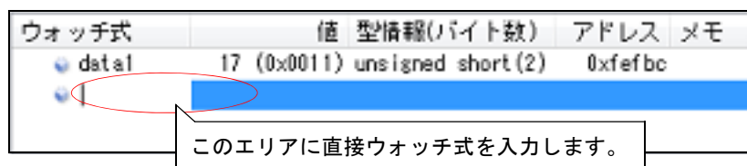
図 2.111 ウォッチ式のエン트리・ボックス
