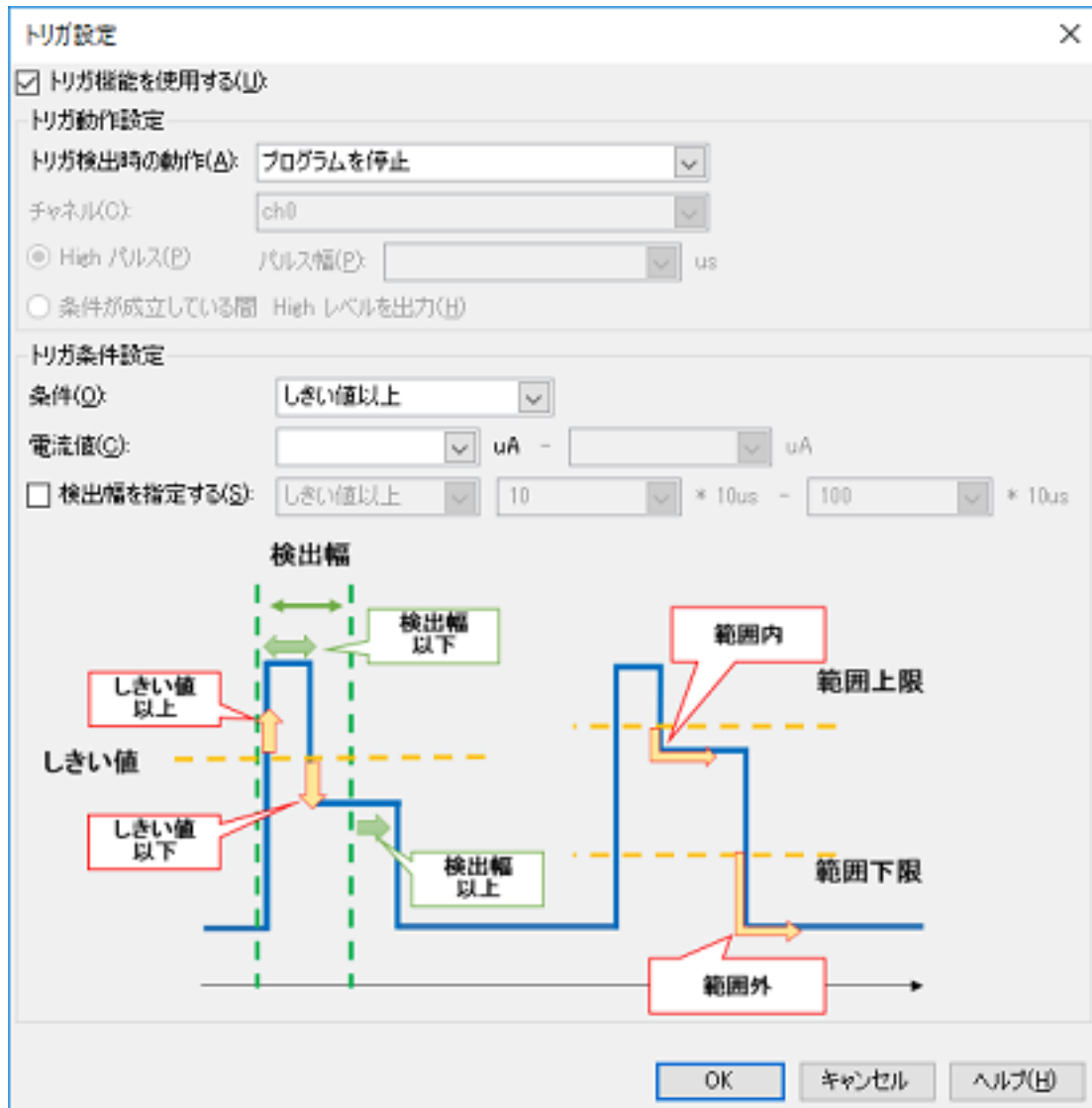
図 2.166 消費電流測定トリガ条件設定ダイアログ
