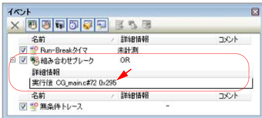
図 2.87 イベントパネルの組み合わせブレイク・イベント（実行系）の設定例【E1】【E20】
