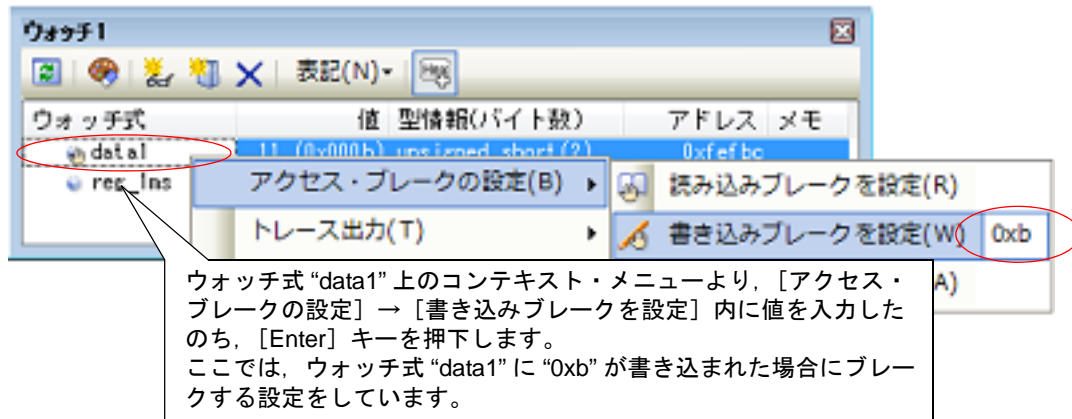
図 2.91 ウォッチ式に対する組み合わせブレーク・イベント（アクセス系）の設定例【E1】【E20】
