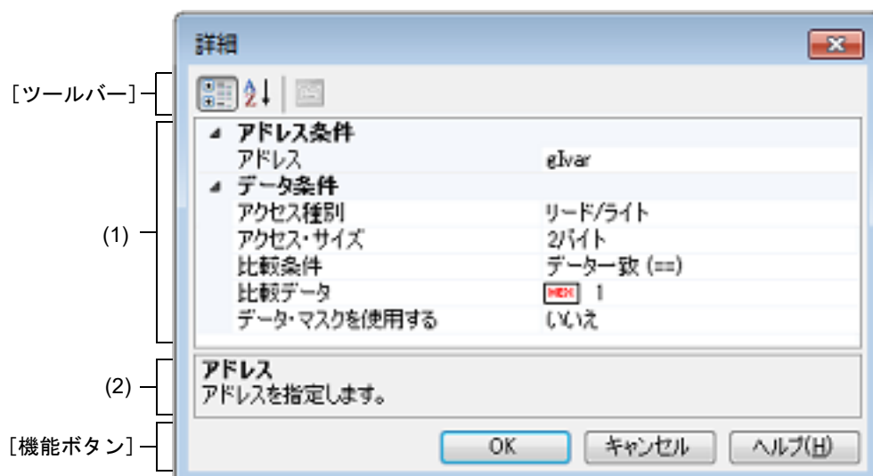
図 A.37 詳細 ダイアログ (アクセス・イベント)【E1】【E20】【EZ Emulator】
