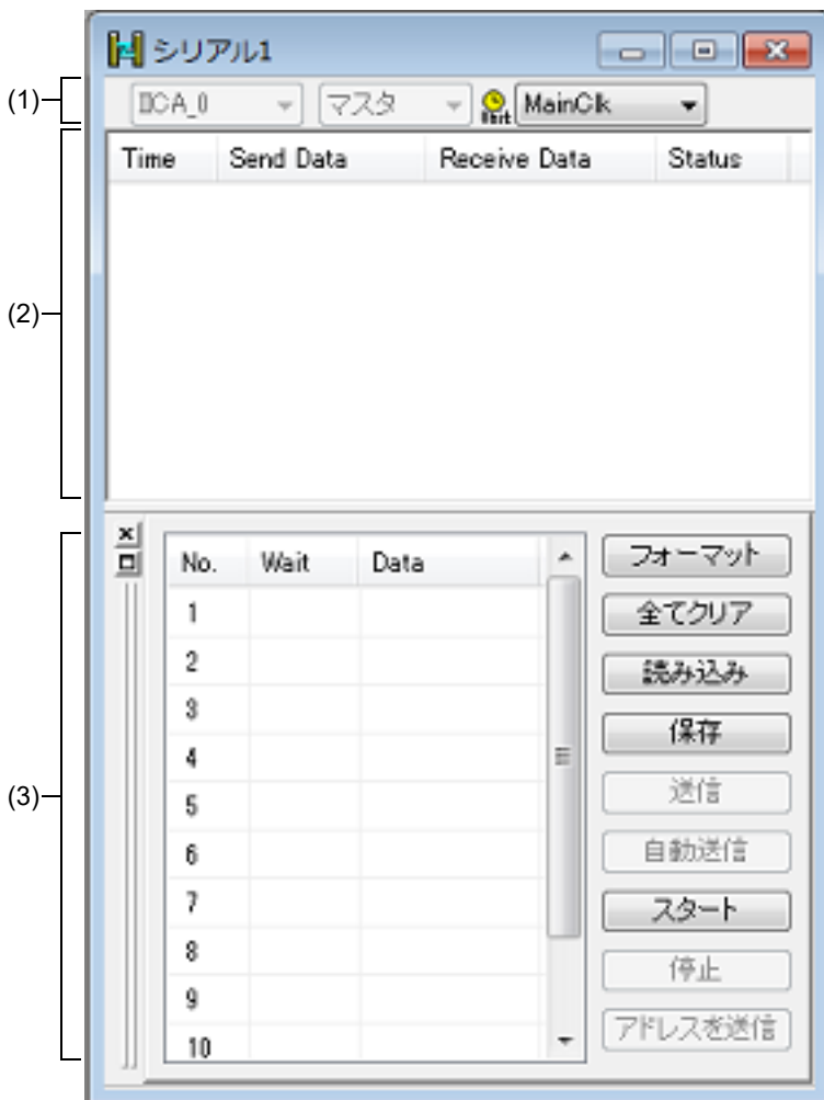
図 A.89 シリアル ウィンドウ
