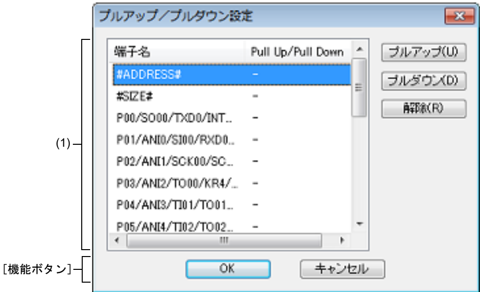
図 A.85 プルアップ／プルダウン設定 ダイアログ
