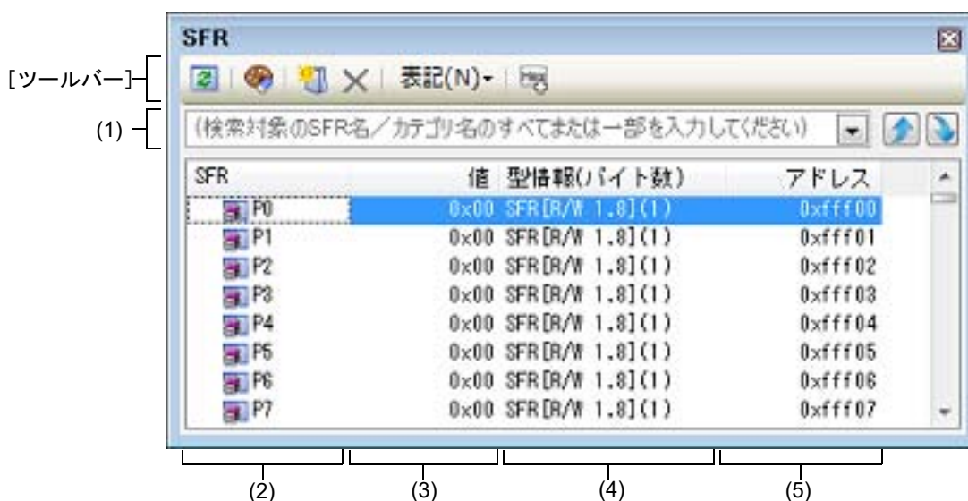
図 A.11 SFR パネル
