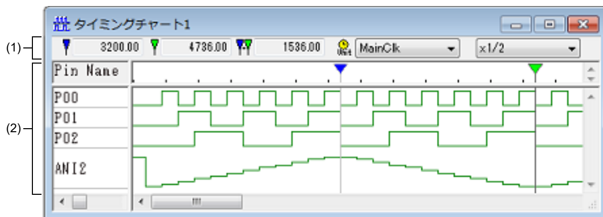
図 A.57 タイミングチャート ウィンドウ
