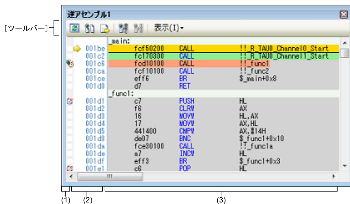
図 A.8 逆アセンブル パネル（コード・カバレージ測定結果を表示した場合）
