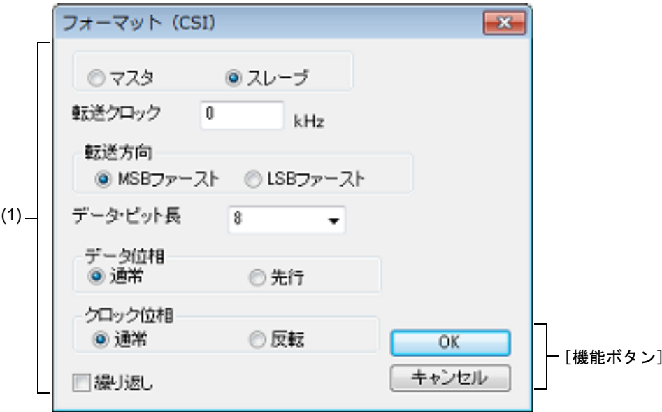
図 A.91 フォーマット（CSI）ダイアログ
