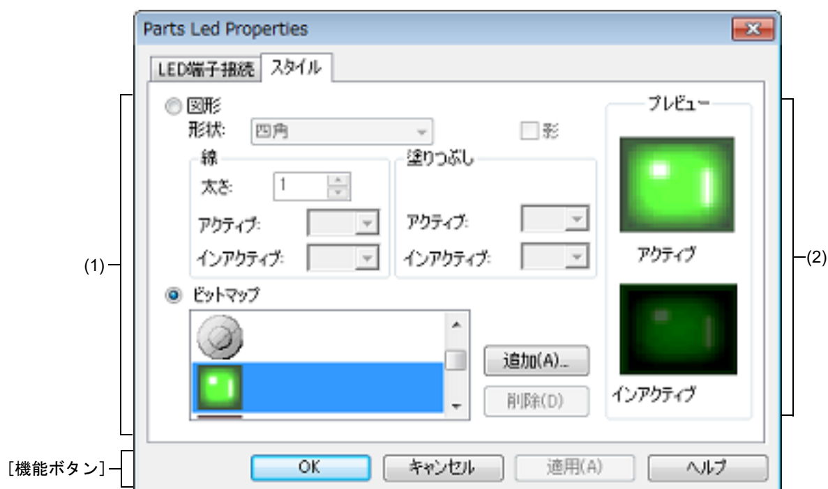
図 A.74 Parts Led Properties ダイアログ : [スタイル] タブ
