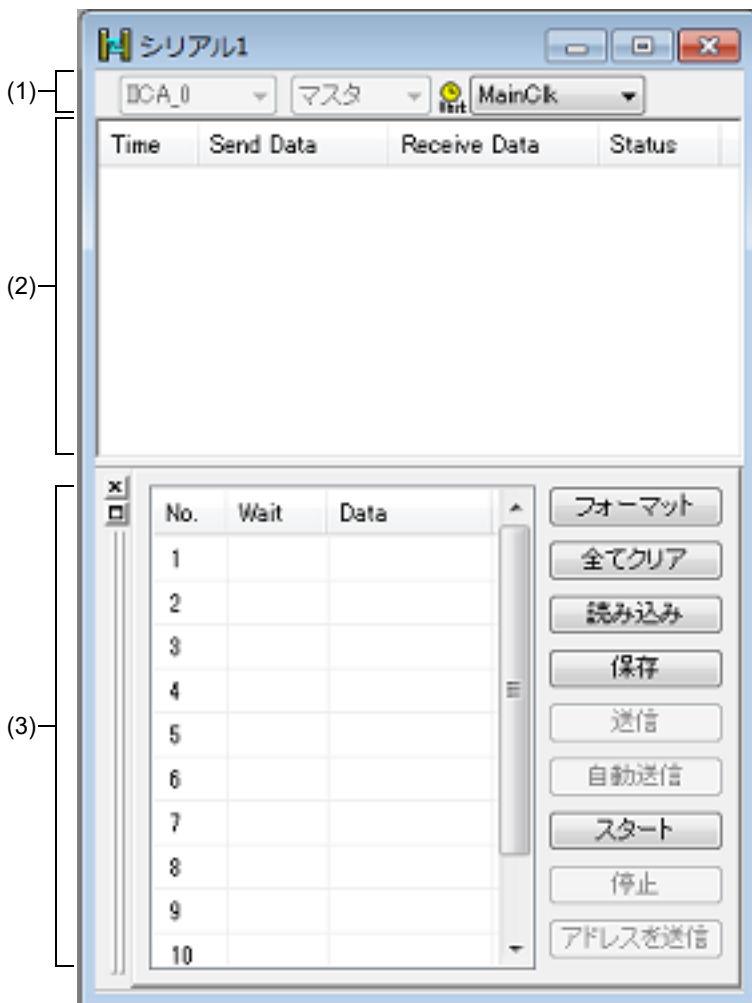
図 A.99 シリアル ウィンドウ
