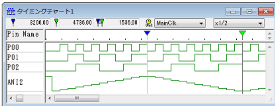
図 2.176 マイコンの入出力波形の確認（タイミングチャート ウィンドウ）
