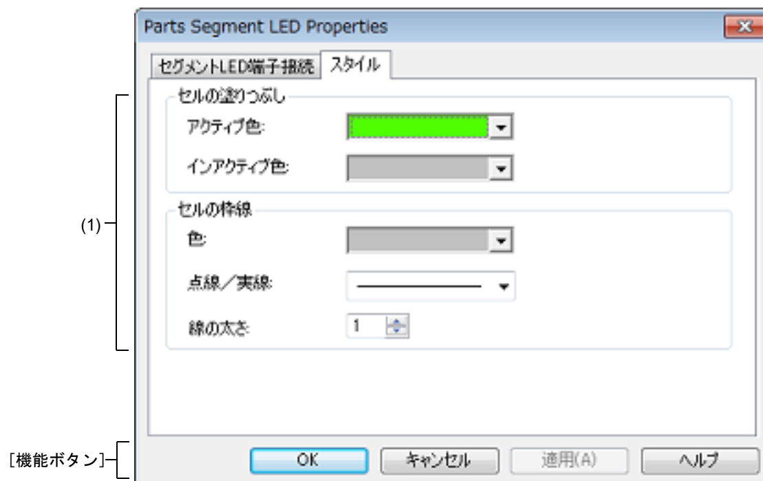
図 A.87 Parts Segment LED Properties ダイアログ : [スタイル] タブ
