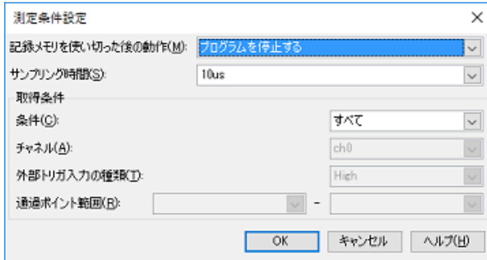
図 2.165 消費電流測定条件設定 ダイアログ
