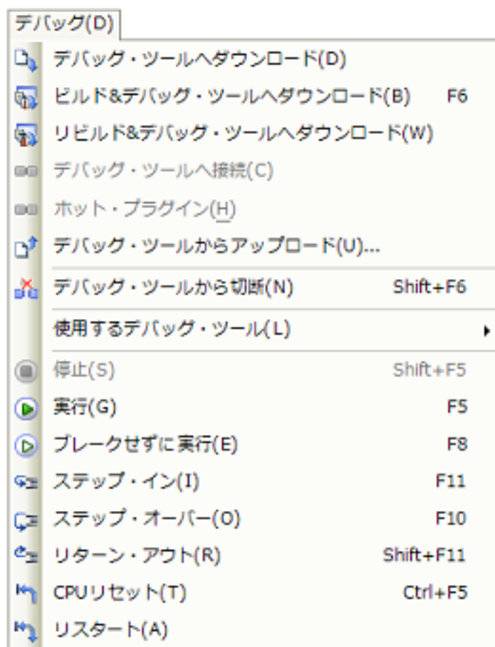
図 2.79 「デバッグ」メニュー
