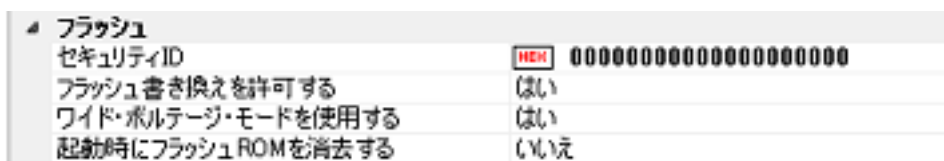
図 2.40 [フラッシュ] カテゴリ
