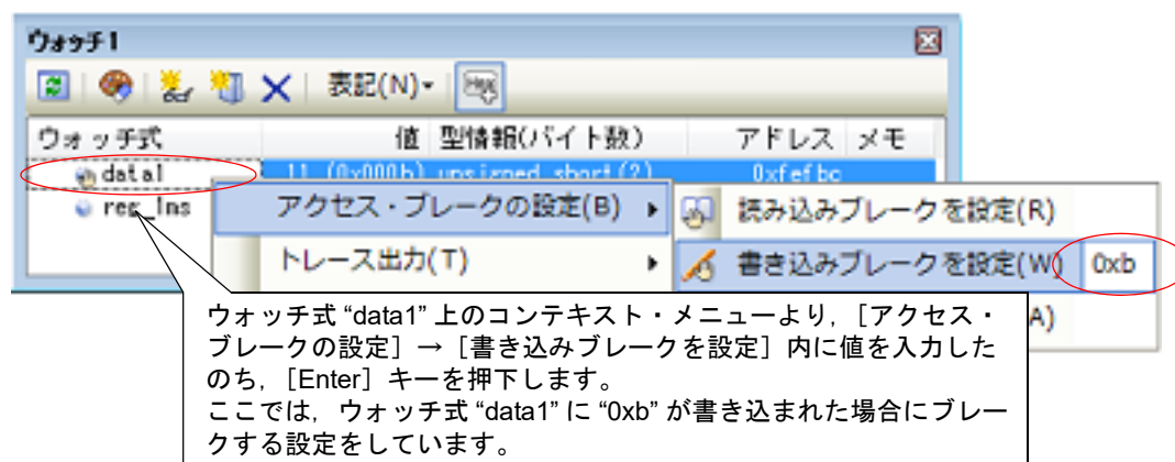
図 2.90 ウォッチ式に対するハードウェア・ブレーク・イベント（アクセス系）の設定例
