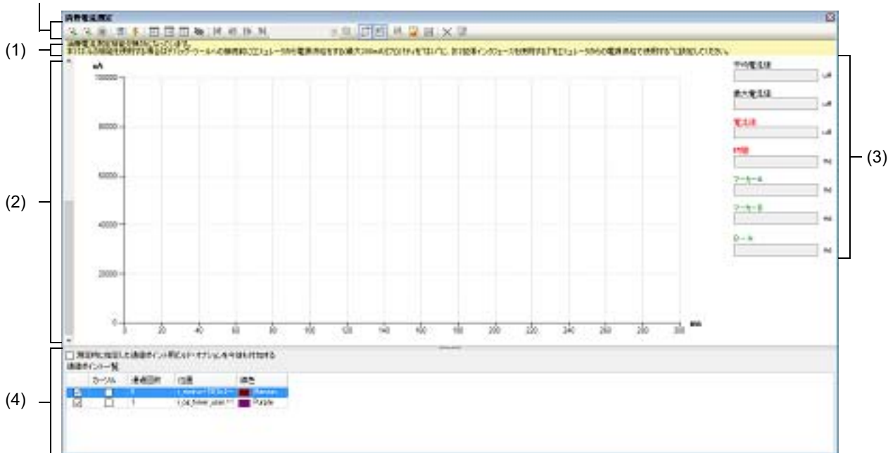
図 A.54 消費電流測定 パネル
