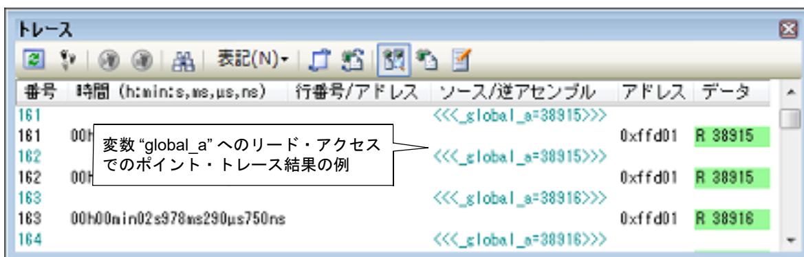
図 2.125 ポイント・トレース・イベントの結果表示例（16 ビット（2 バイト）変数 /SFR の場合）【IECUBE】
