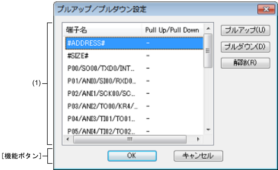
図 A.95 プルアップ／プルダウン設定 ダイアログ
