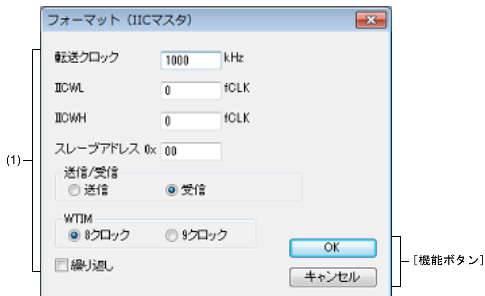
図 A.102 フォーマット（IIC マスタ）ダイアログ
