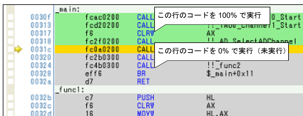
図 2.143 コード・カバレッジ測定結果の表示例（逆アセンブル パネル）
