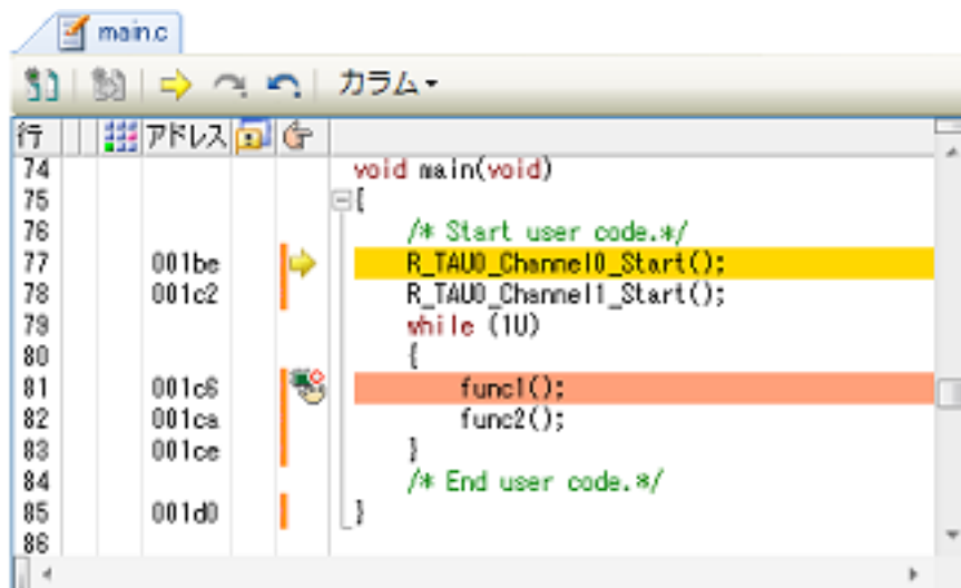
図 2.71 ソース・ファイルの表示（エディタ パネル）
