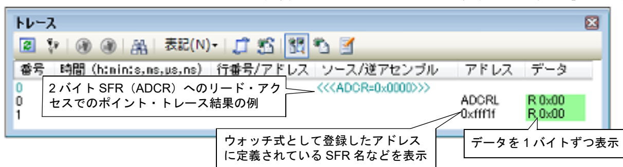
図 2.125 ポイント・トレース・イベントの結果表示例（16 ビット（2 バイト）変数 /SFR の場合）【IECUBE】
