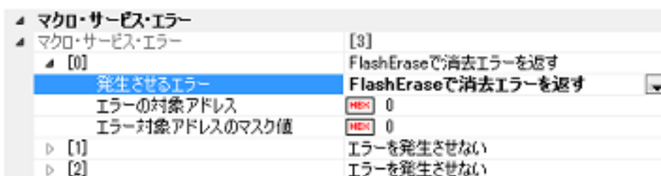
図 2.18 [マクロ・サービス・エラー] カテゴリ
