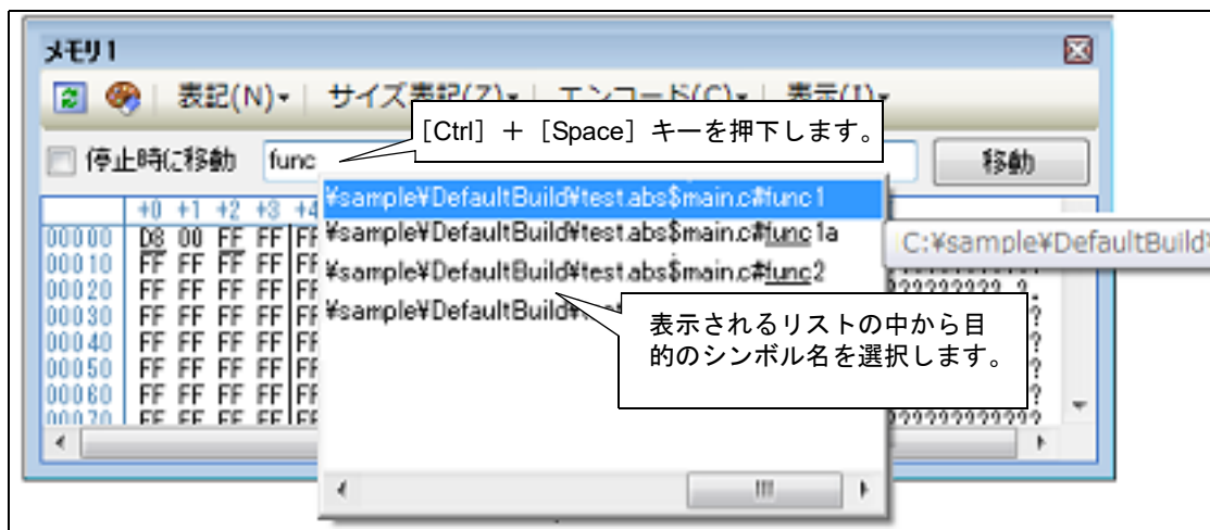
図 2.180 シンボル名の入力補完機能
