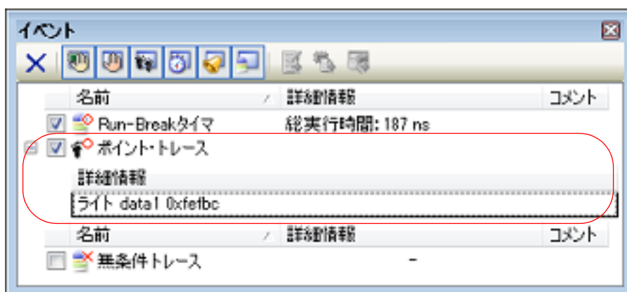
図 2.123 イベントパネルのポイント・トレース・イベントの設定例
