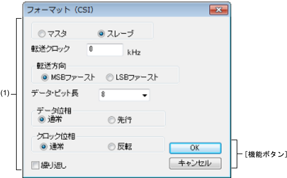
図 A.101 フォーマット（CSI）ダイアログ
