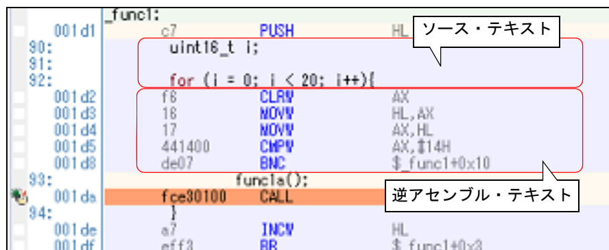
図 2.73 混合表示モード（逆アセンブル パネル）
