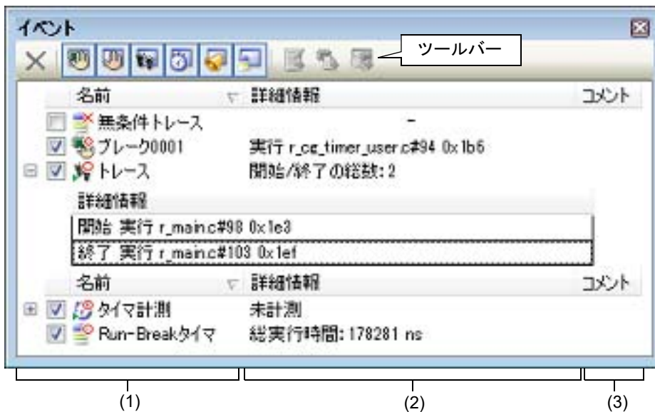
図 2.146 設定したイベントの表示（イベントパネル）
