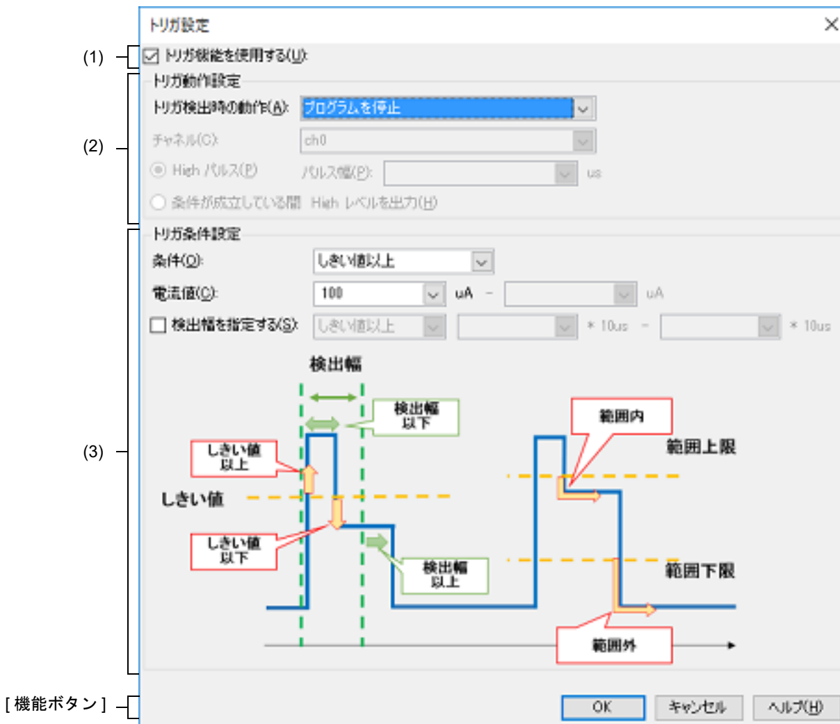
図 A.57 消費電流測定トリガ条件設定 ダイアログ
