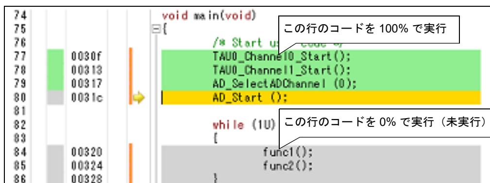
図 2.143 コード・カバレッジ測定結果の表示例（逆アセンブル パネル）
