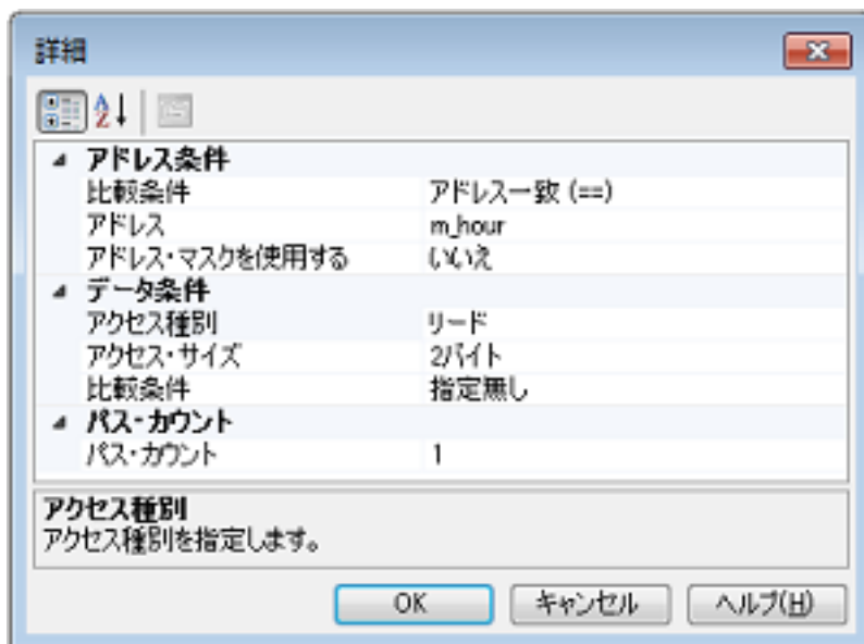
図 2.153 詳細 ダイアログ（アクセス・イベント）の例【シミュレータ】
