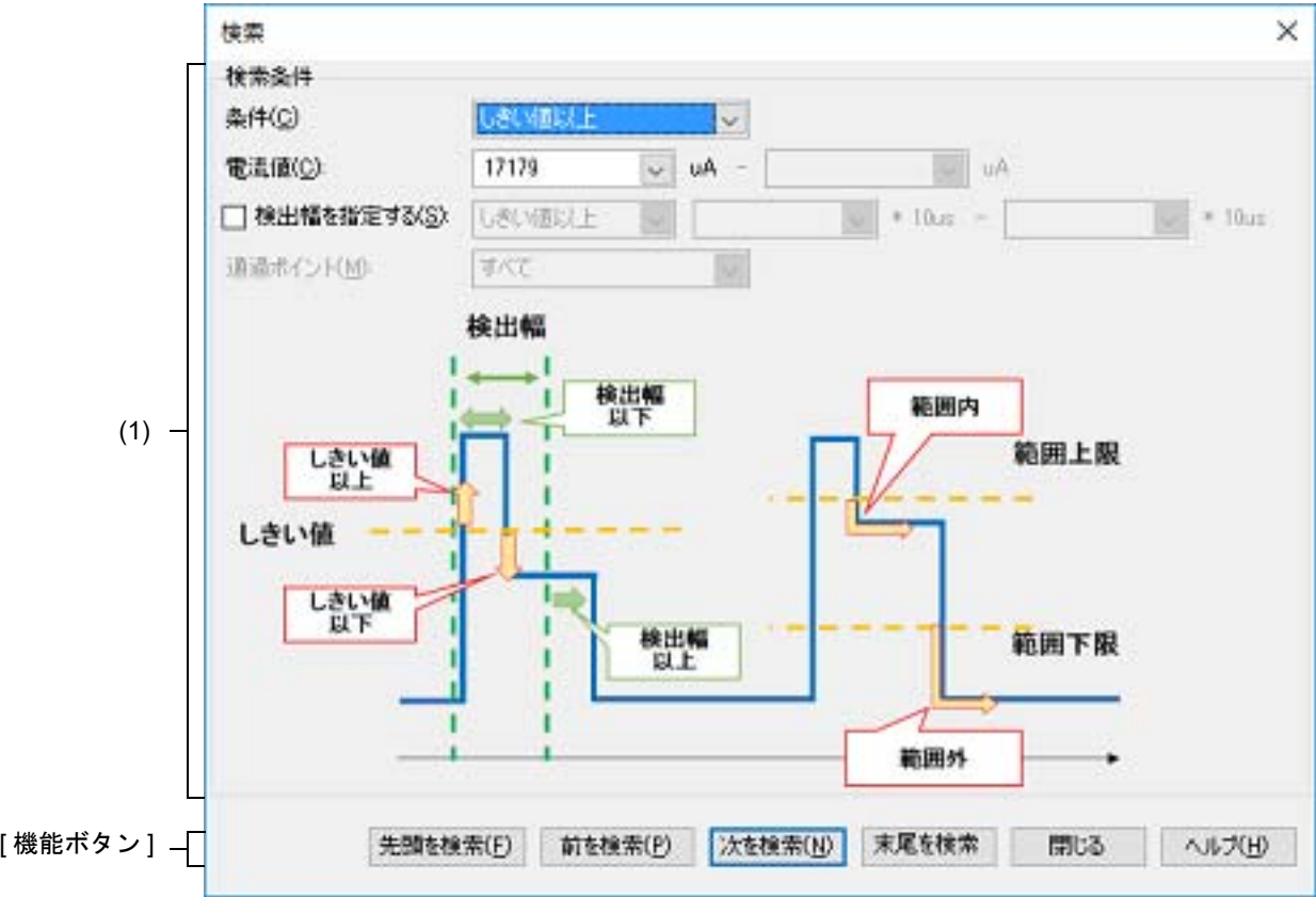
図 A.58 消費電流測定検索 ダイアログ
