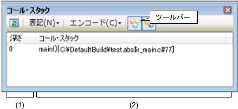
図 2.115 コール・スタック情報の表示（コール・スタック パネル）
