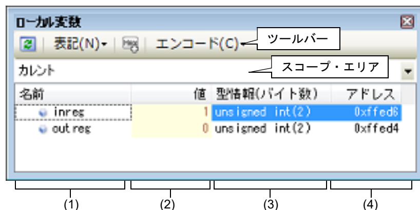
図 2.107 ローカル変数の内容の表示（ローカル変数 パネル）
