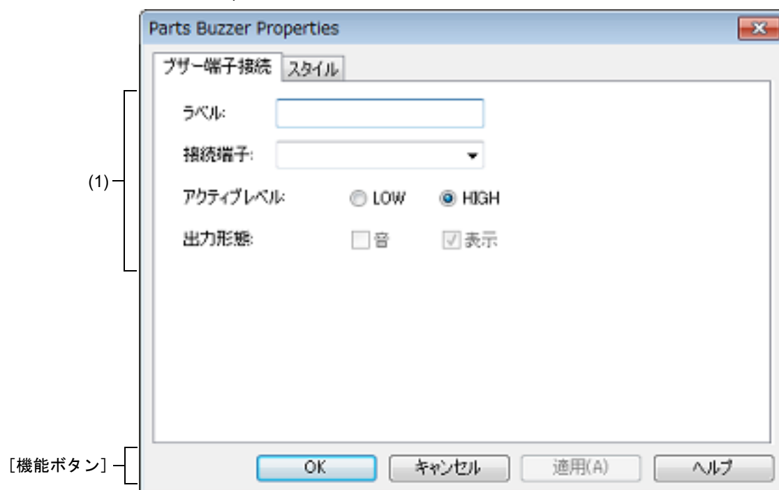
図 A.92 Parts Buzzer Properties ダイアログ : [ブザー端子接続] タブ
