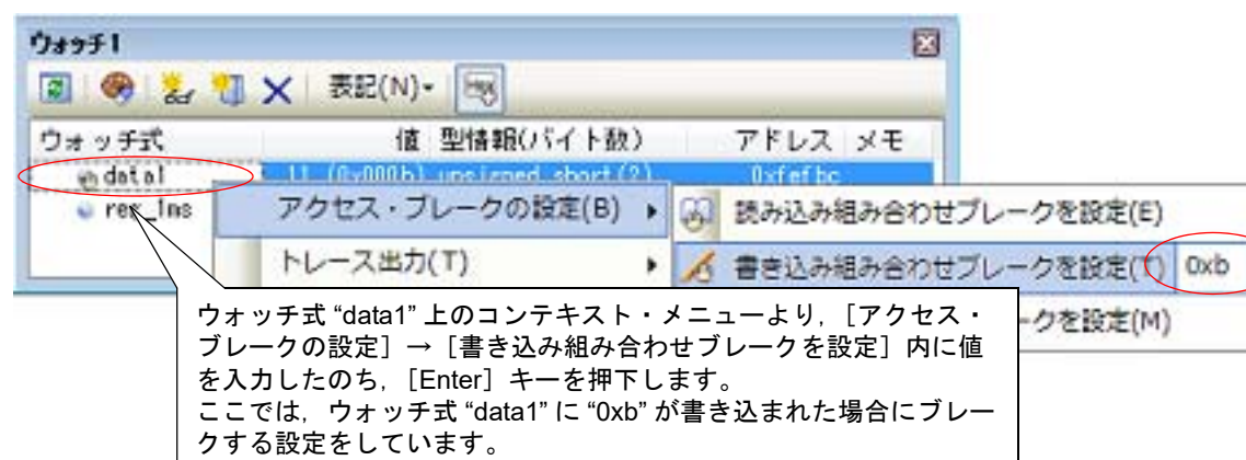
図 2.91 ウォッチ式に対する組み合わせブレーク・イベント（アクセス系）の設定例【E1】【E20】
