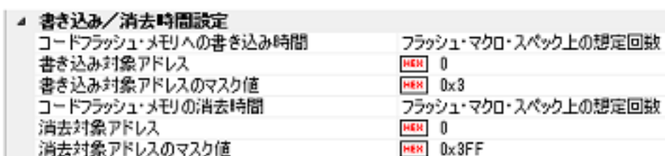
図 2.17 [書き込み／消去時間設定] カテゴリ
