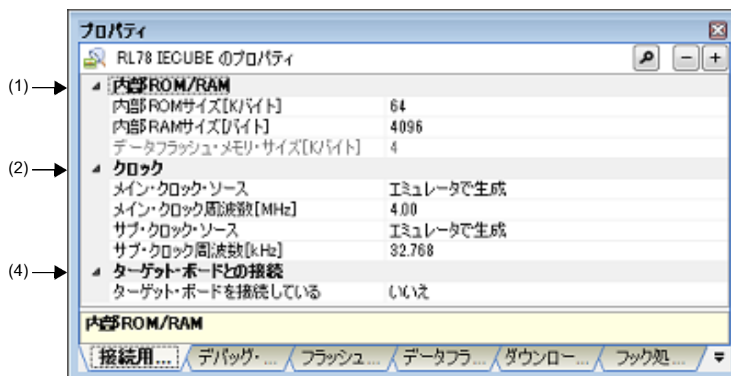
図 A.5 プロパティ パネル：〔接続用設定〕 タブ【IECUBE】
