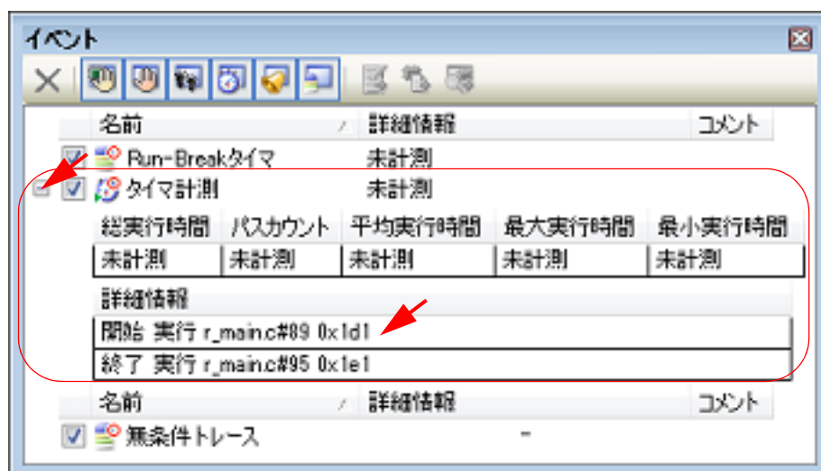
図 2.138 イベント パネルのタイマ開始イベント／タイマ終了イベント（実行系）の設定例
