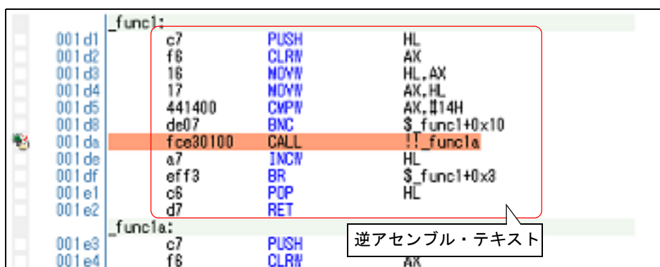
図 2.74 逆アセンブル表示モード（逆アセンブル パネル）
