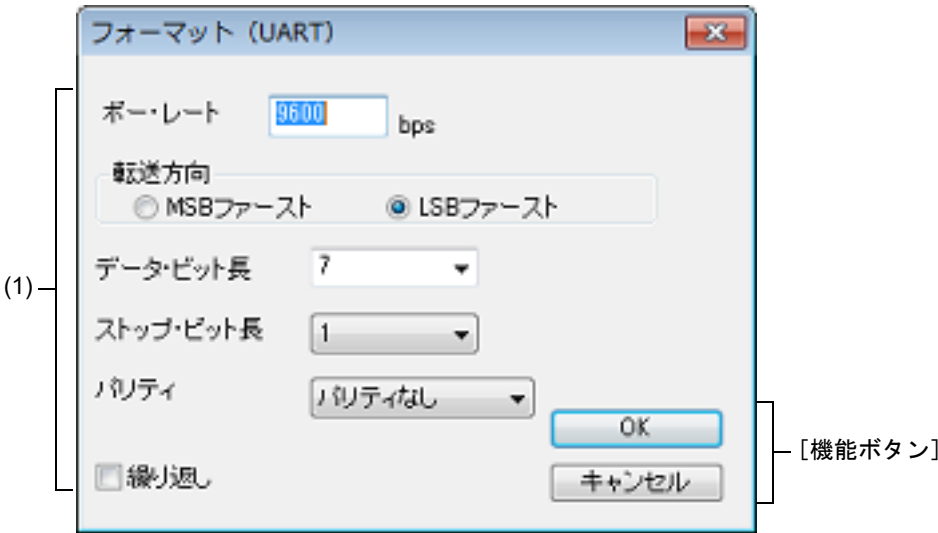
図 A.100 フォーマット（UART）ダイアログ
