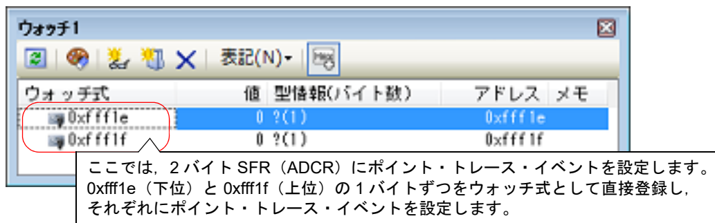
図 2.122 16 ビット (2 バイト) 変数 /SFR へのポイント・トレース・イベントの設定方法【IECUBE】
