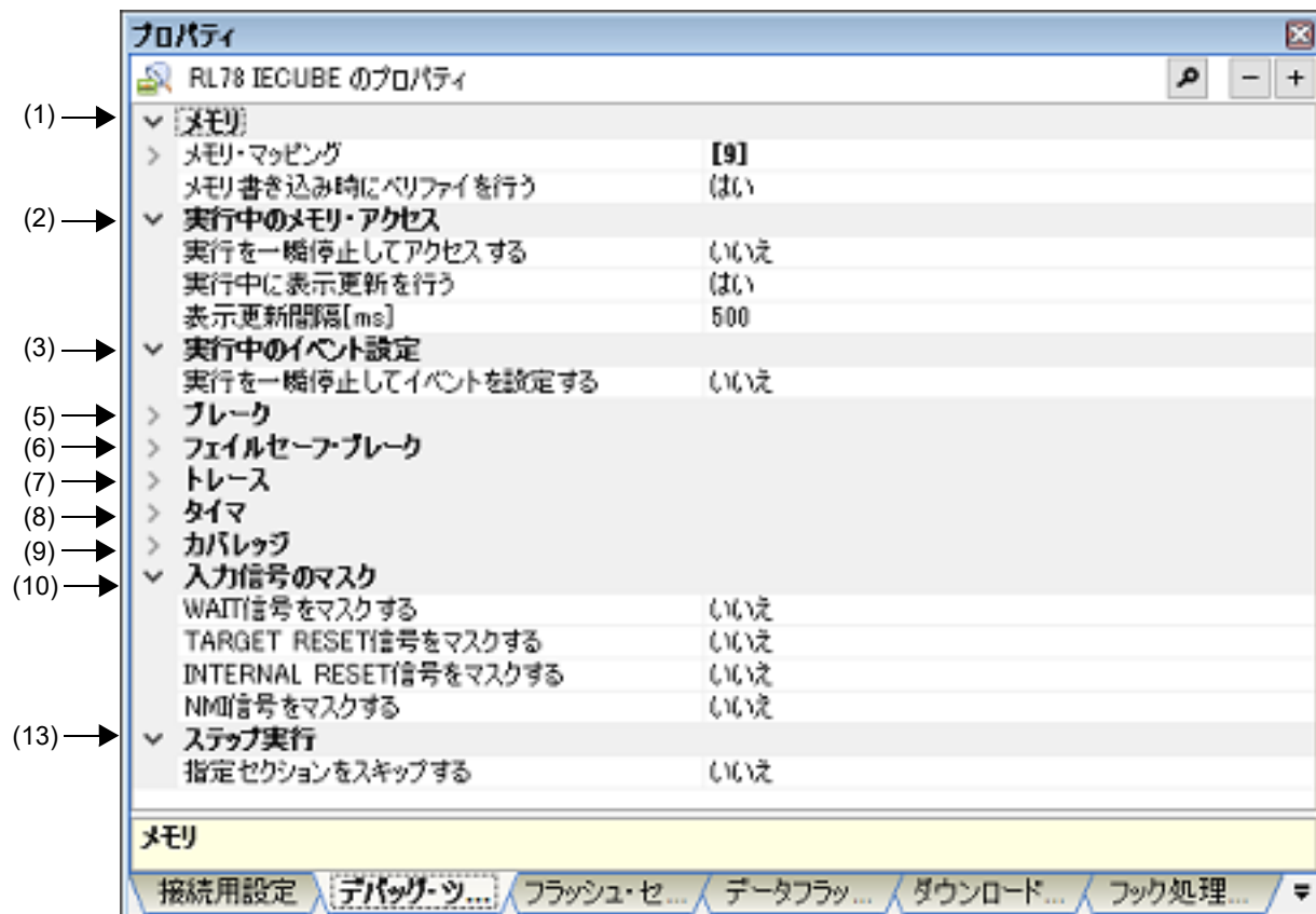
図 A.8 プロパティ パネル : [デバッグ・ツール設定] タブ【IECUBE】
