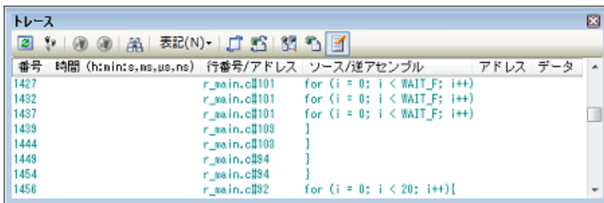
図 2.127 ソース表示モードの例（トレース パネル）
