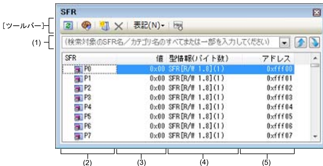
図 A.21 SFR パネル
