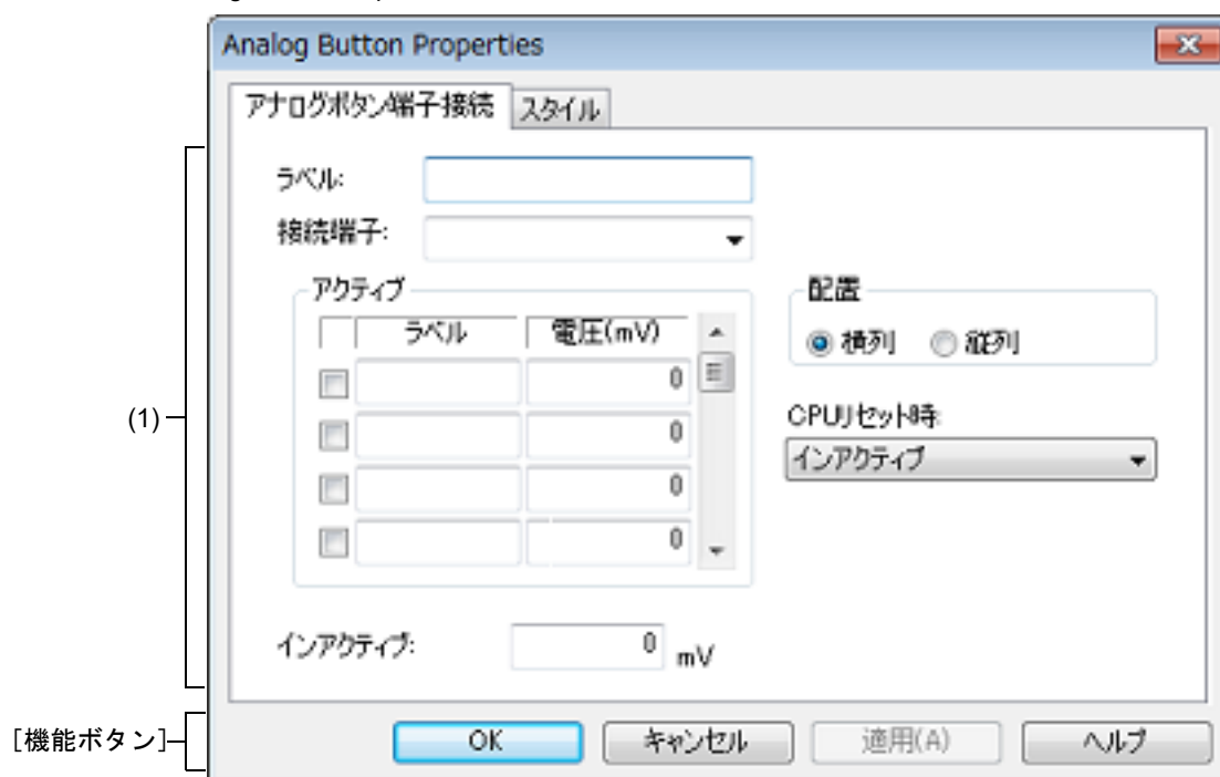
図 A.74 Analog Button Properties ダイアログ : [アナログボタン端子接続] タブ
