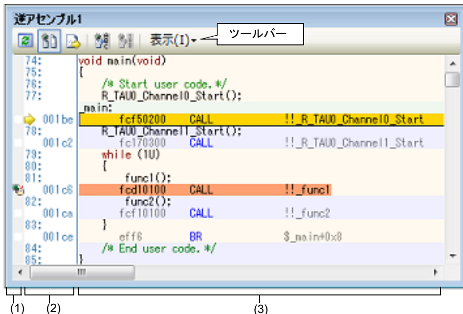
図 2.72 逆アセンブル結果の表示（逆アセンブル パネル）
