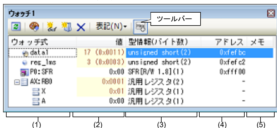
図 2.109 ウォッチ式の内容の表示（ウォッチパネル）
