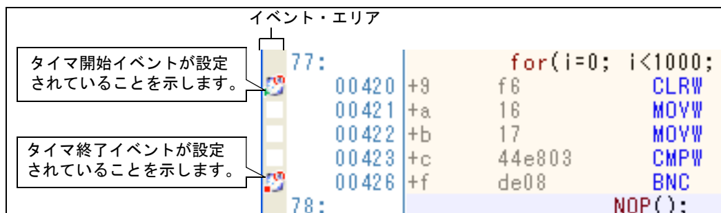
図 2.137 タイマ開始イベント／タイマ終了イベントの設定例（逆アセンブル パネルの場合）
