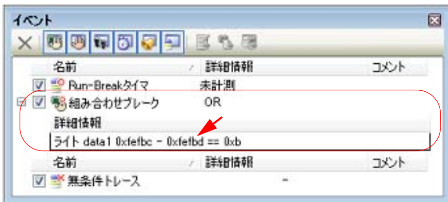
図 2.93 イベントパネルの組み合わせブレイク・イベント（アクセス系）の設定例【E1】【E20】
