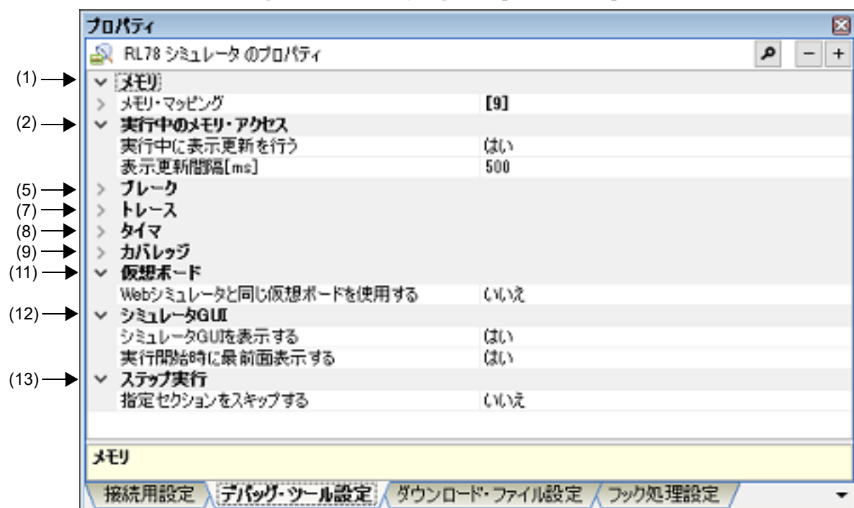
図 A.10 プロパティ パネル：[デバッグ・ツール設定] タブ【シミュレータ】
