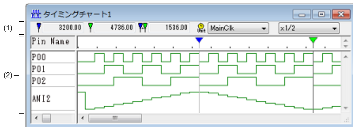
図 A.67 タイミングチャート ウィンドウ
