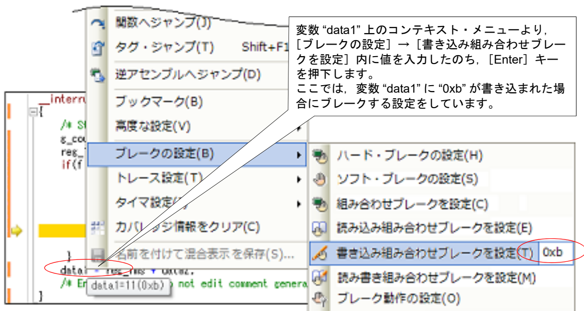
図 2.89 エディタ パネル上の変数に対する組み合わせブレーク・イベント（アクセス系）の設定例【E1】【E20】
