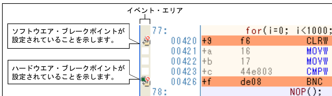
図 2.83 ブレークポイントの設定例（逆アセンブル パネルの場合）
