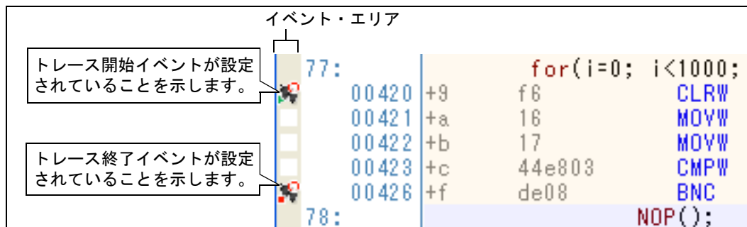
図 2.120 トレース開始イベント／トレース終了イベントの設定例（逆アセンブル パネルの場合）
