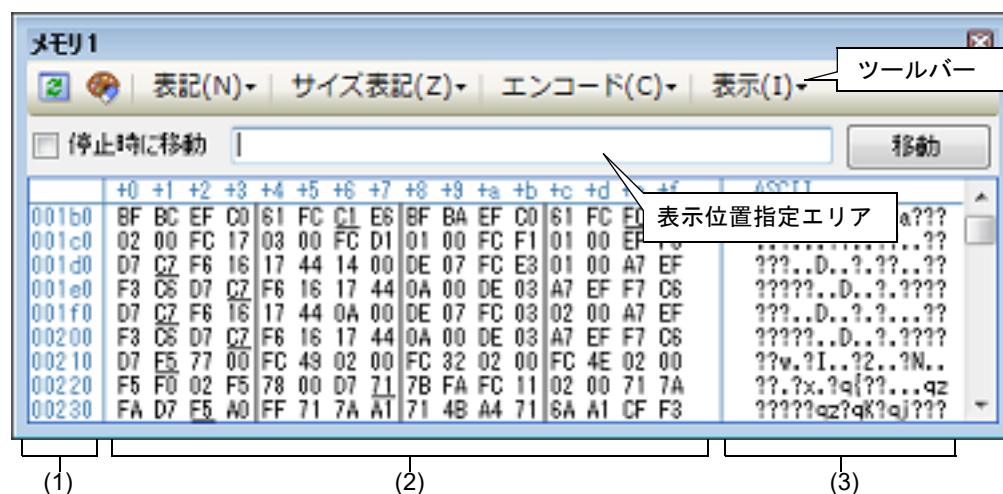
図 2.95 メモリの内容の表示（メモリ パネル）
