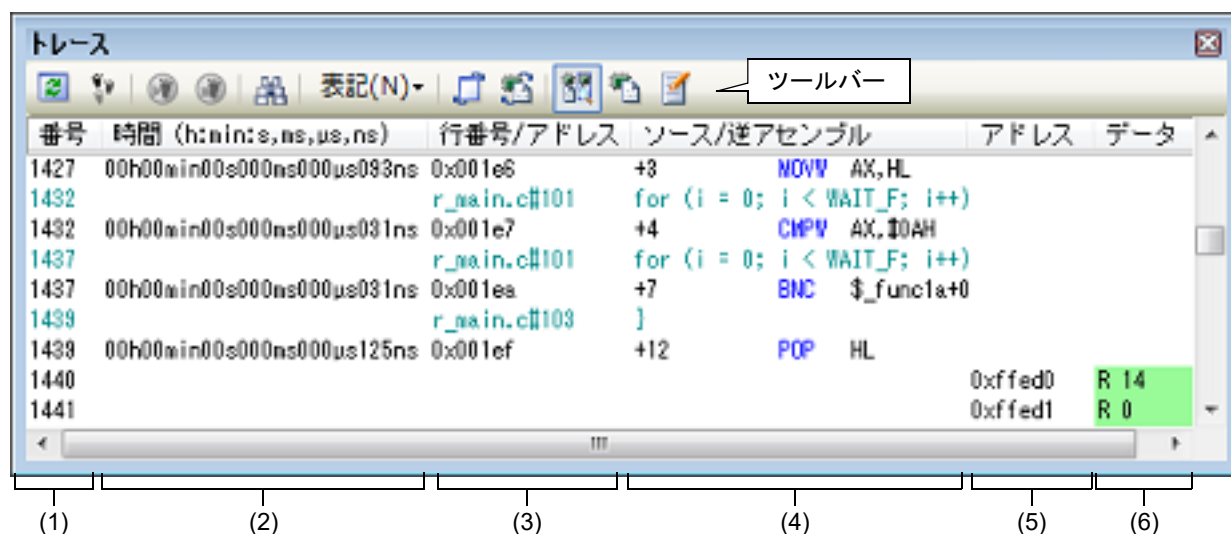
図 2.126 トレース・データの表示（トレース パネル）
