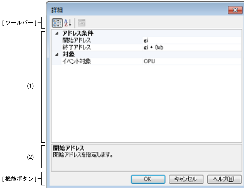
図 A.48 ポイント・トレース詳細設定ダイアログ【Full-spec emulator】【E1】【E20】
