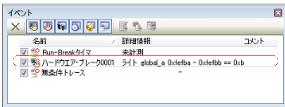
図 2.82 イベントパネルのハードウェア・ブレーク・イベント（アクセス系）の設定例
