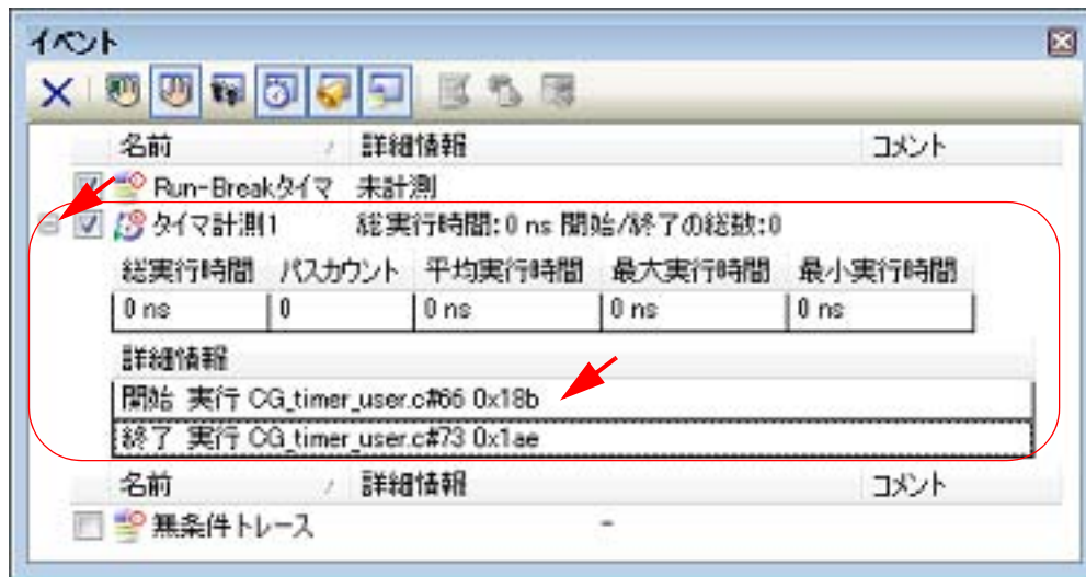
図 2.123 イベントパネルのタイマ開始イベント／タイマ終了イベント（実行系）の設定例【Full-spec emulator】 【E1】【E20】
