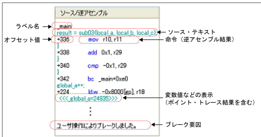
図 A.27 [ソース/逆アセンブル] エリアの表示内容 (デフォルト)
