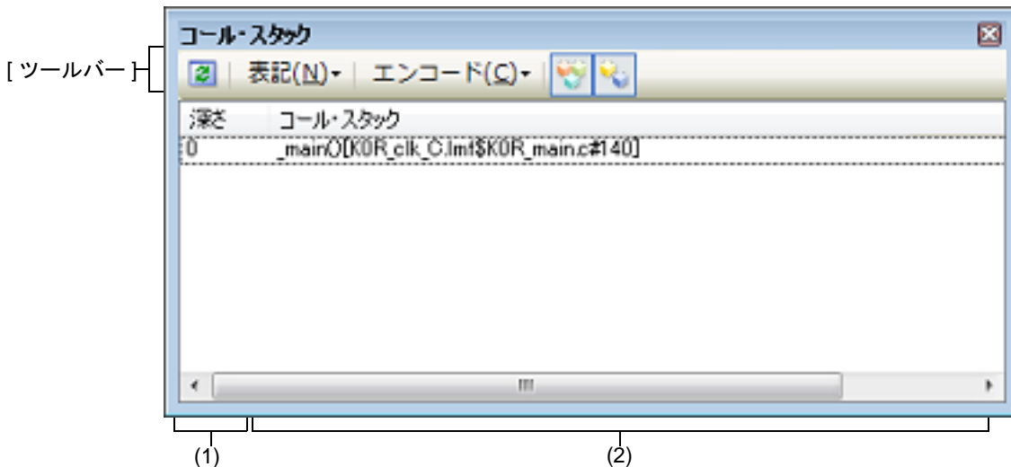
図 A.24 コール・スタック パネル
