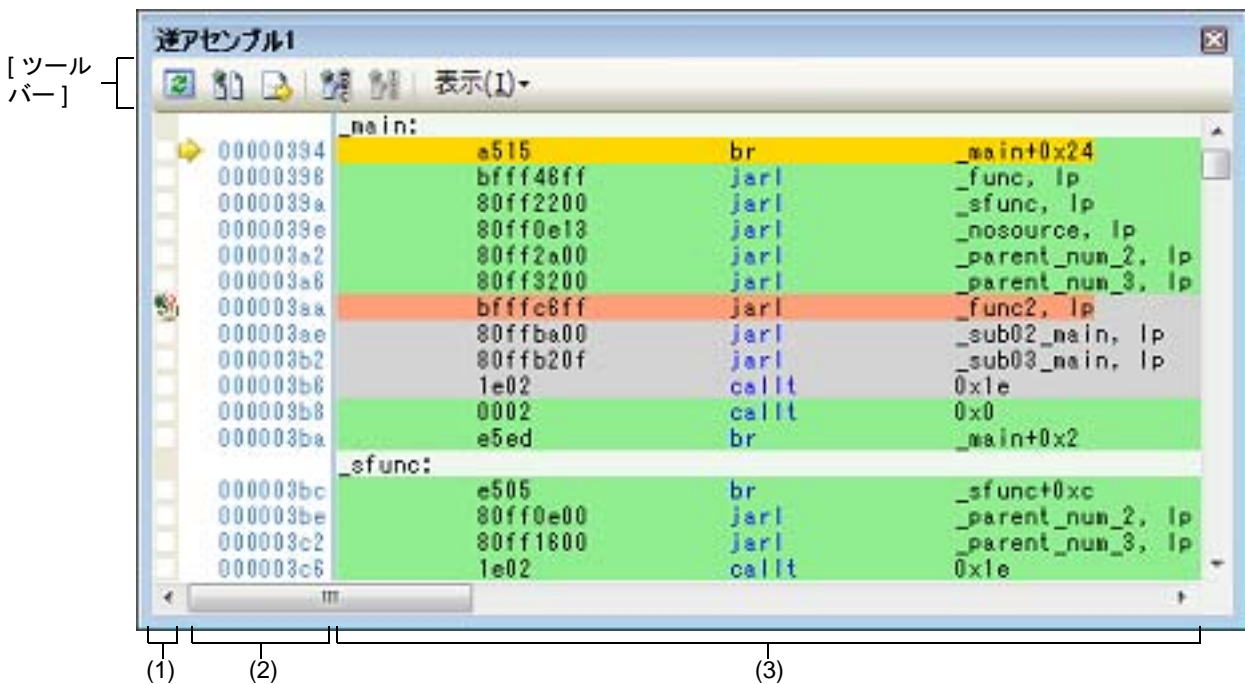
図 A.18 逆アセンブル パネル（コード・カバレッジ測定結果を表示した場合）【シミュレータ】
