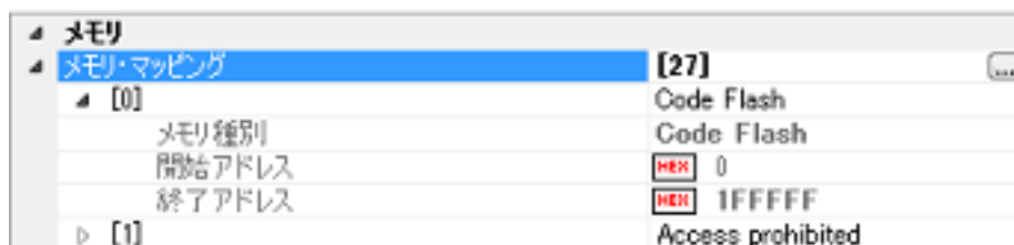
図 2.37 メモリ・マッピングの詳細表示
