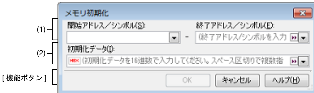
図 A.42 メモリ初期化 ダイアログ
