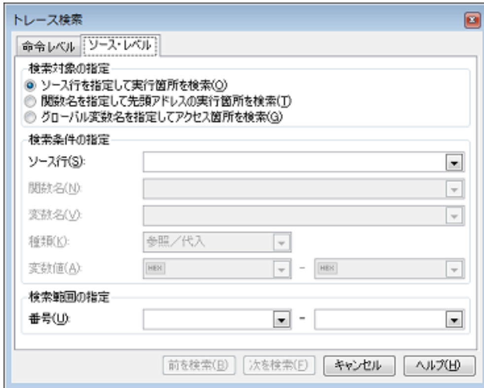
図 2.116 ソース・レベルでのトレース・データの検索
