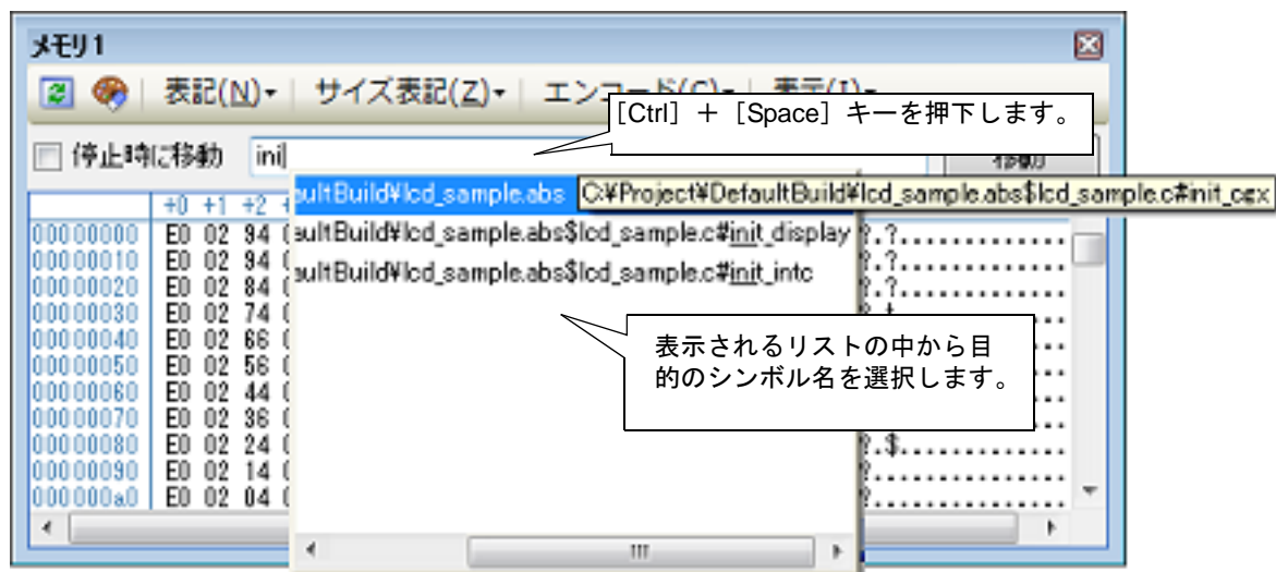
図 2.137 シンボル名の入力補完機能
