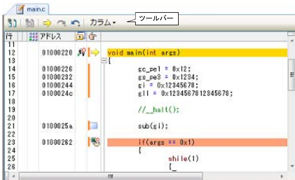
図 2.64 ソース・ファイルの表示（エディタ パネル）
