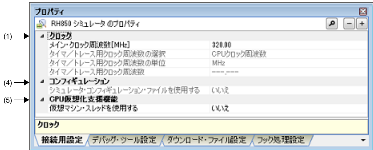
図 A.8 プロパティ パネル：[接続用設定] タブ【シミュレータ】
