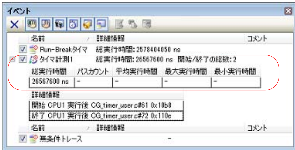
図 2.125 タイマ計測イベント（タイマ開始イベント／タイマ終了イベント）の測定結果例【Full-spec emulator】 【E1】【E20】
