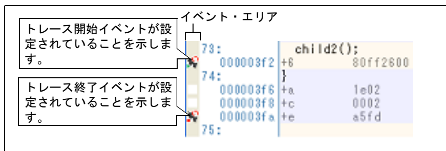
図 2.107 トレース開始イベント/トレース終了イベントの設定例（逆アセンブルパネルの場合）
