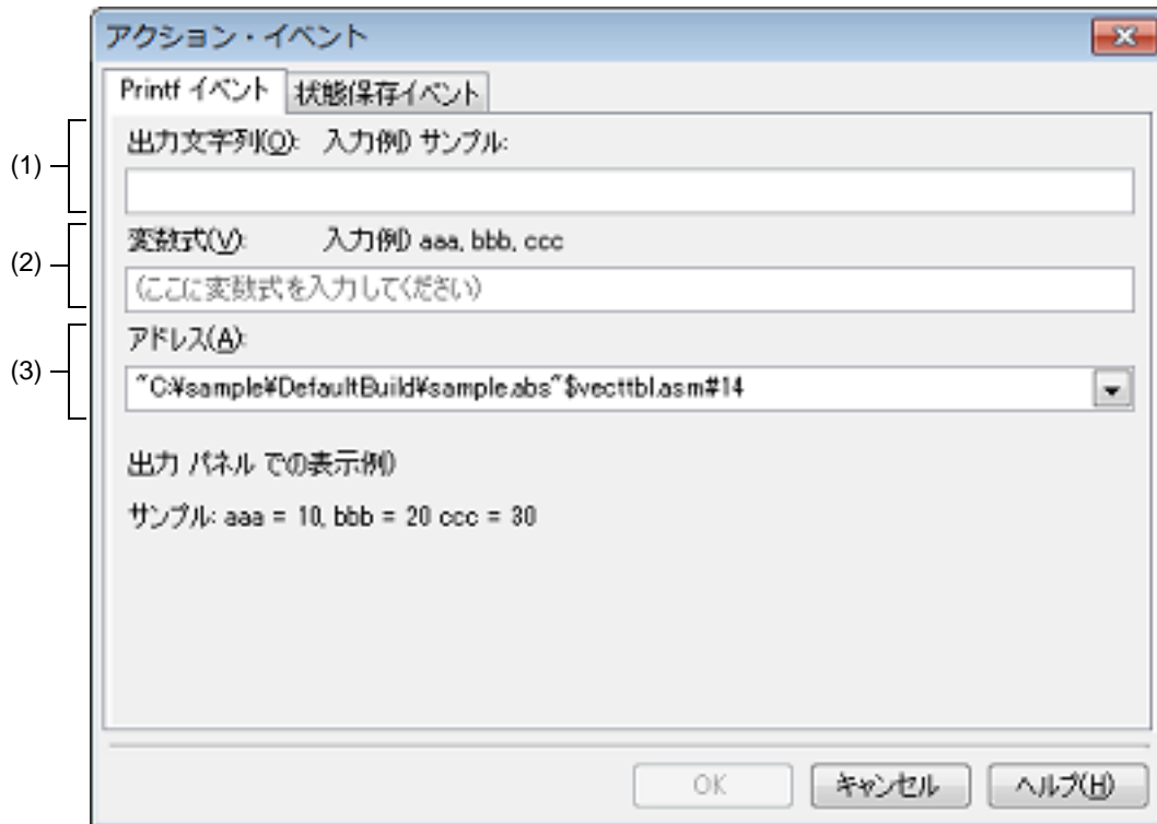
図 A.37 アクション・イベント ダイアログ : [Printf イベント] タブ
