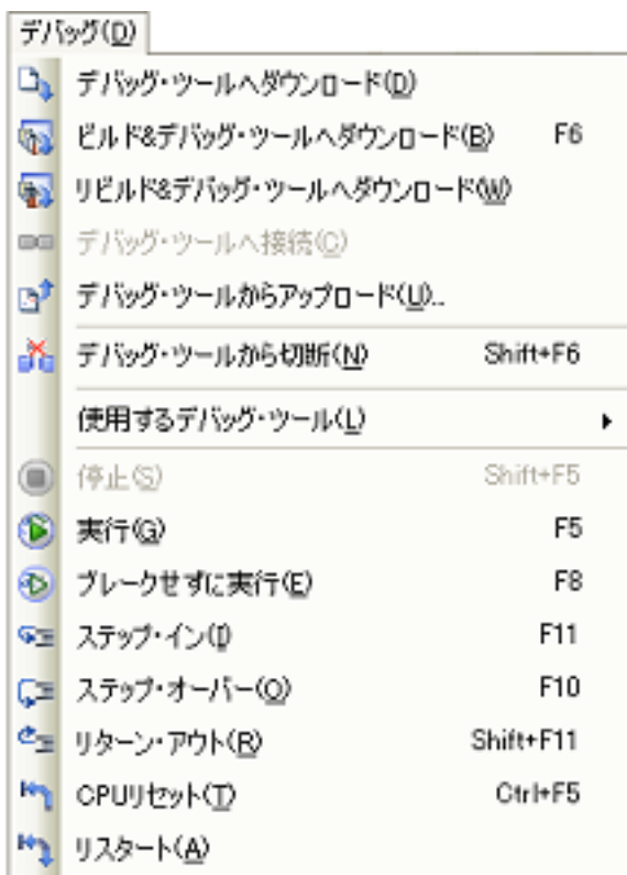
図 2.74 「デバッグ」メニュー
