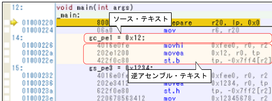
図 2.66 混合表示モード (逆アセンブル パネル)
