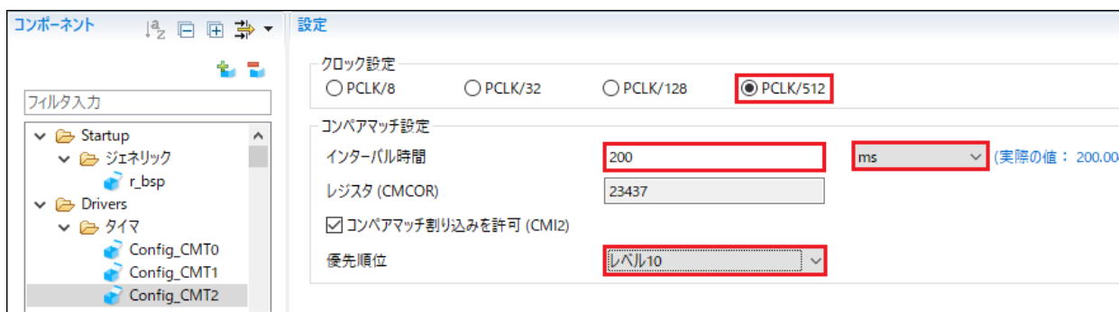
図 4-19: Config_CMT2 設定
