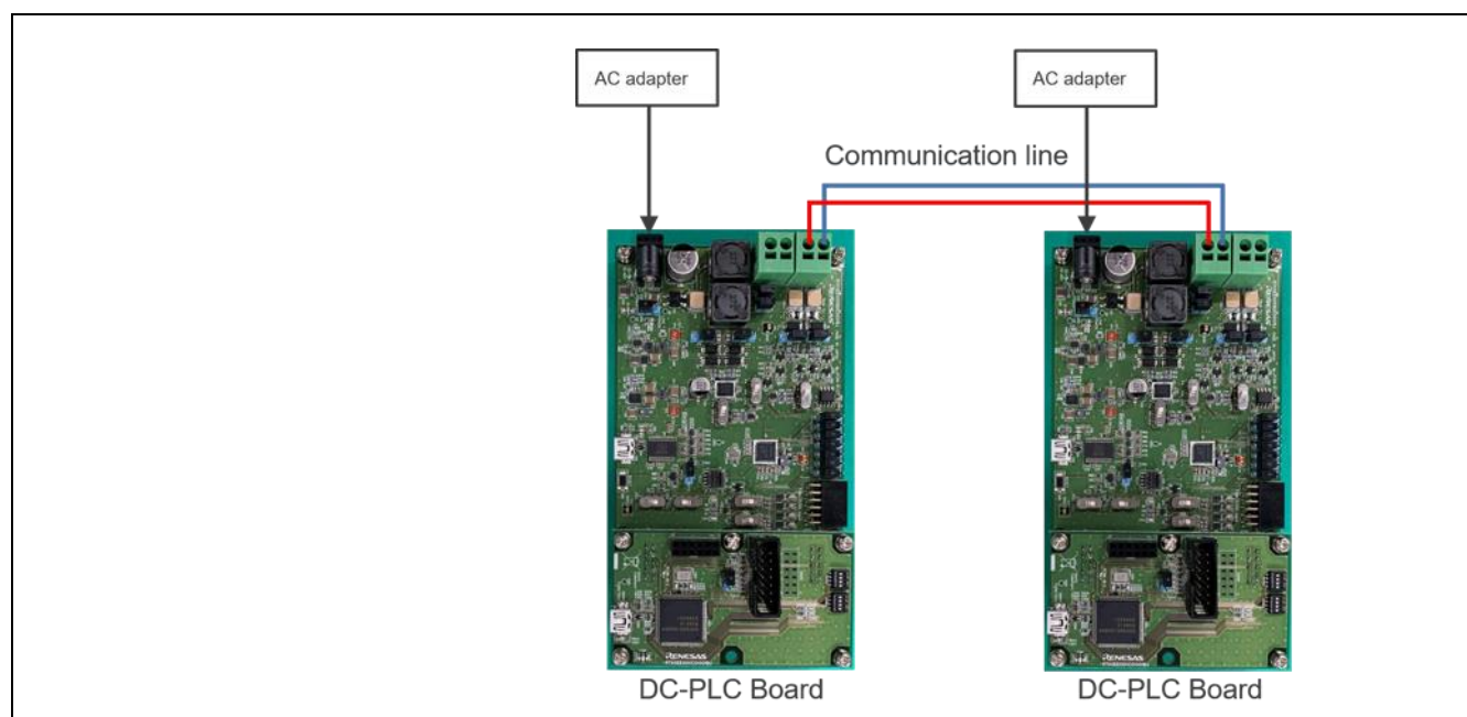
Figure 2-4 通信ラインに電圧をかけない場合の接続例（ACアダプターよりボード給電）
