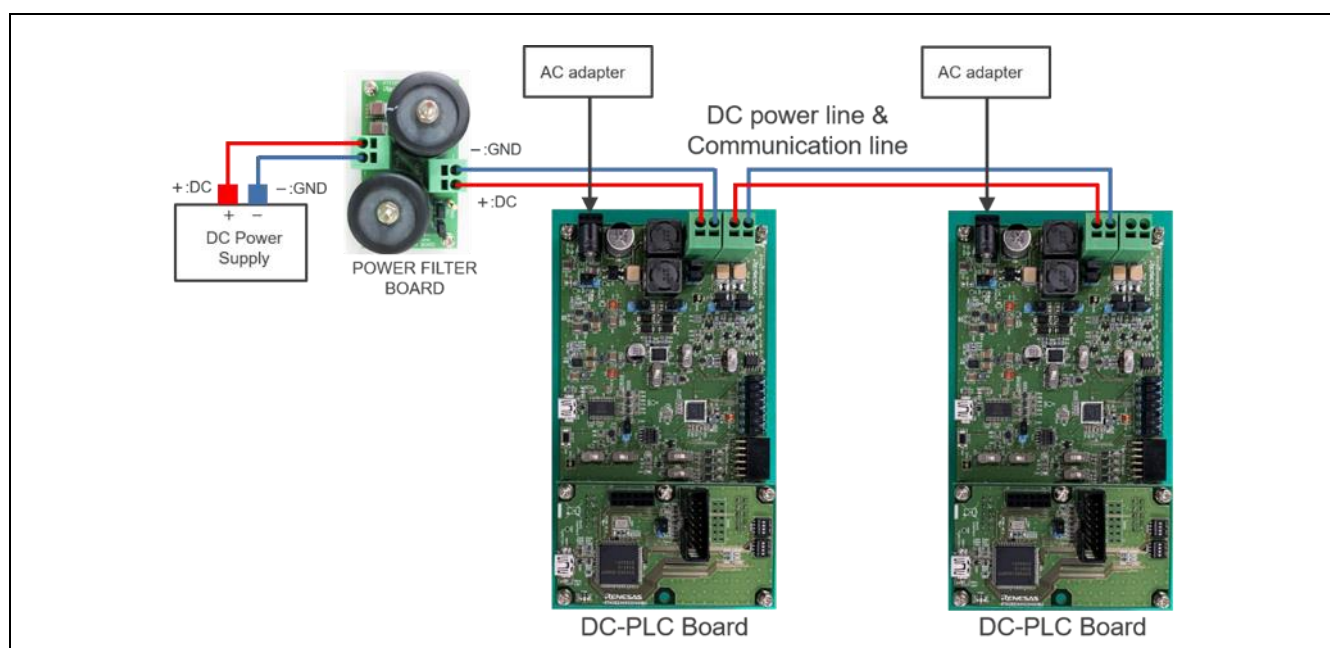
Figure 2-3 通信ラインに電圧をかけた場合の接続例（ACアダプターよりボード給電）
