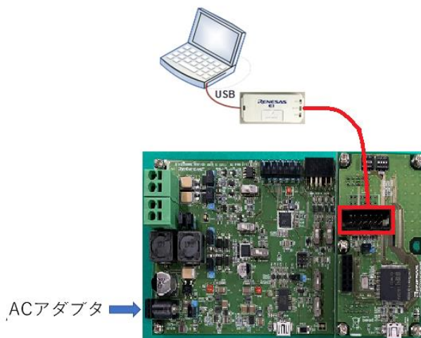
Figure 3-3 エミュレータ - RX651 MCUボード接続構成
