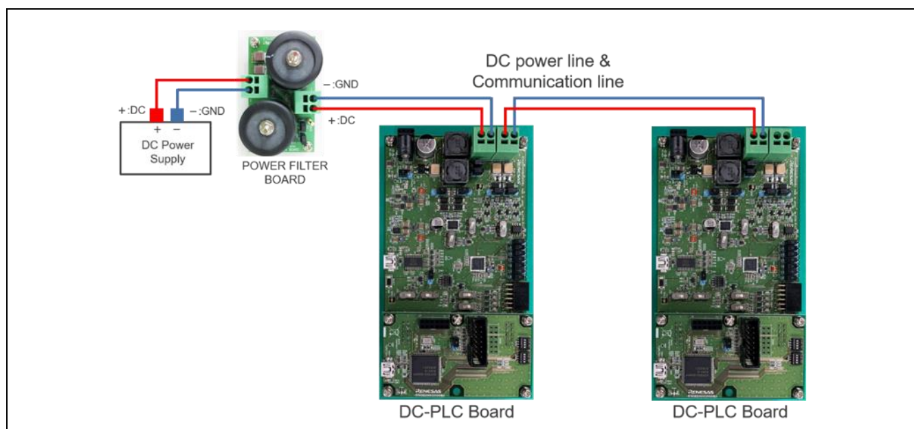
Figure 2-2 通信ラインに電圧をかけた場合の接続例（通信ラインよりボード給電）
