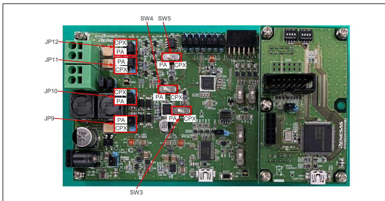
Figure 2-6 駆動方式の設定箇所
